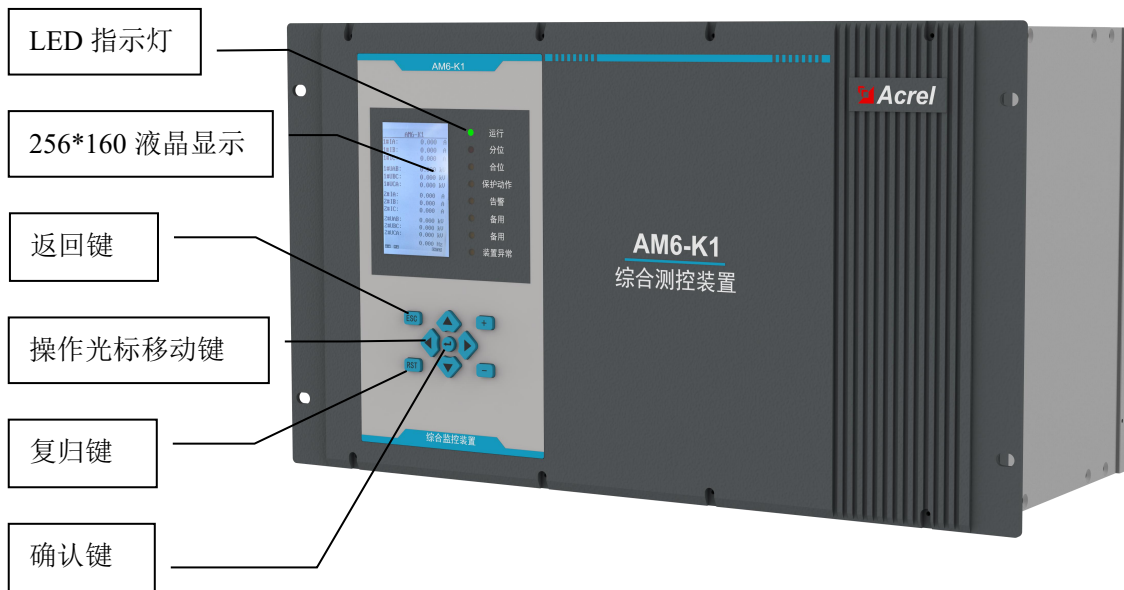
图 3.1 AM6-K1 前面板
