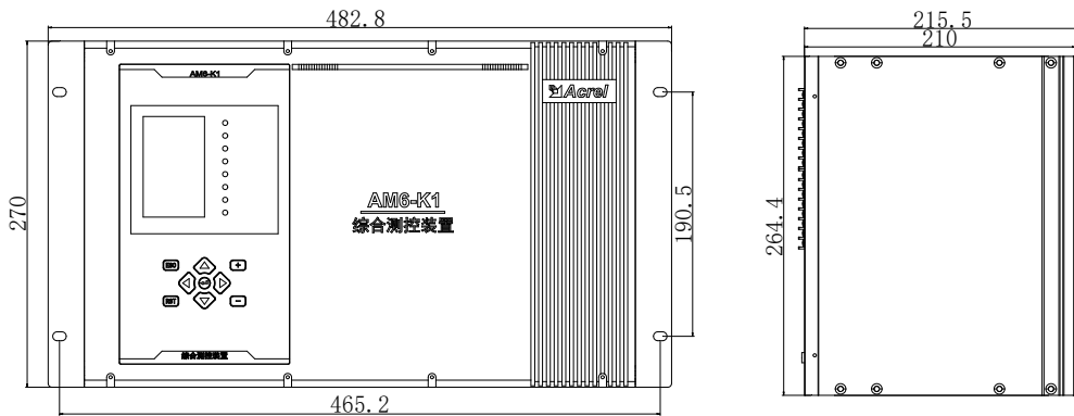
图 4.1 外形尺寸图
