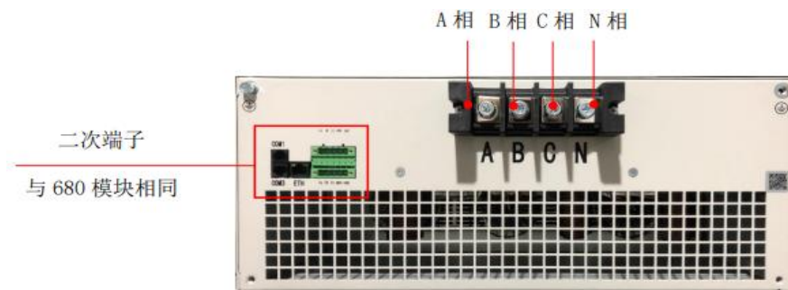
图4-24 50kvar-25A模块端子示意图
