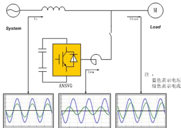
图3-1 ANSVG-G-A 工作原理图
