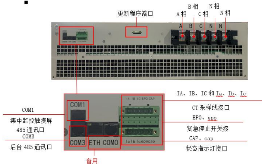
图4-22 150kvar-75A模块端子示意图
