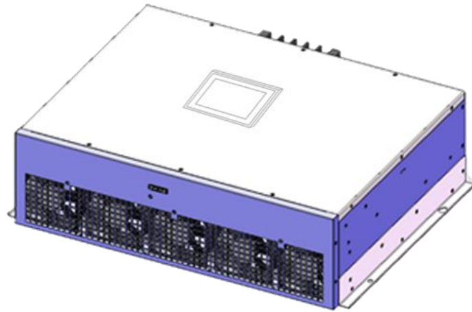
图4-8 75kvar-37.5A/100kvar-50A壁挂式模块外观
