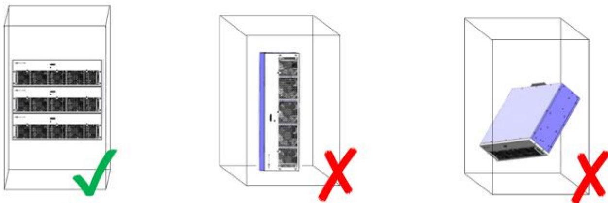
图6-4 模块安装方向示意图
