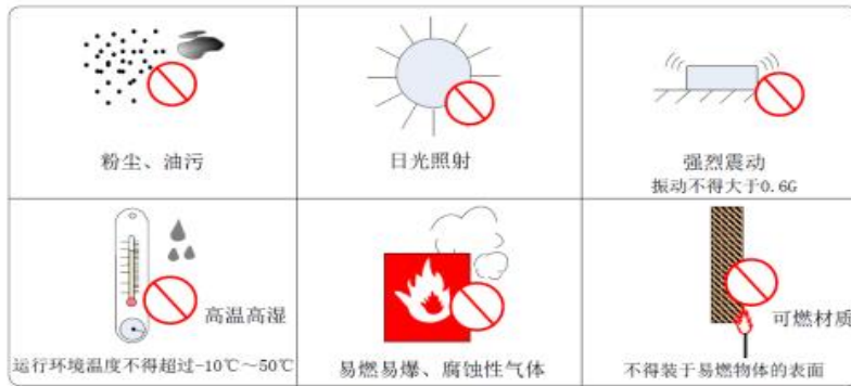
图6-1 安装环境要求示意图
