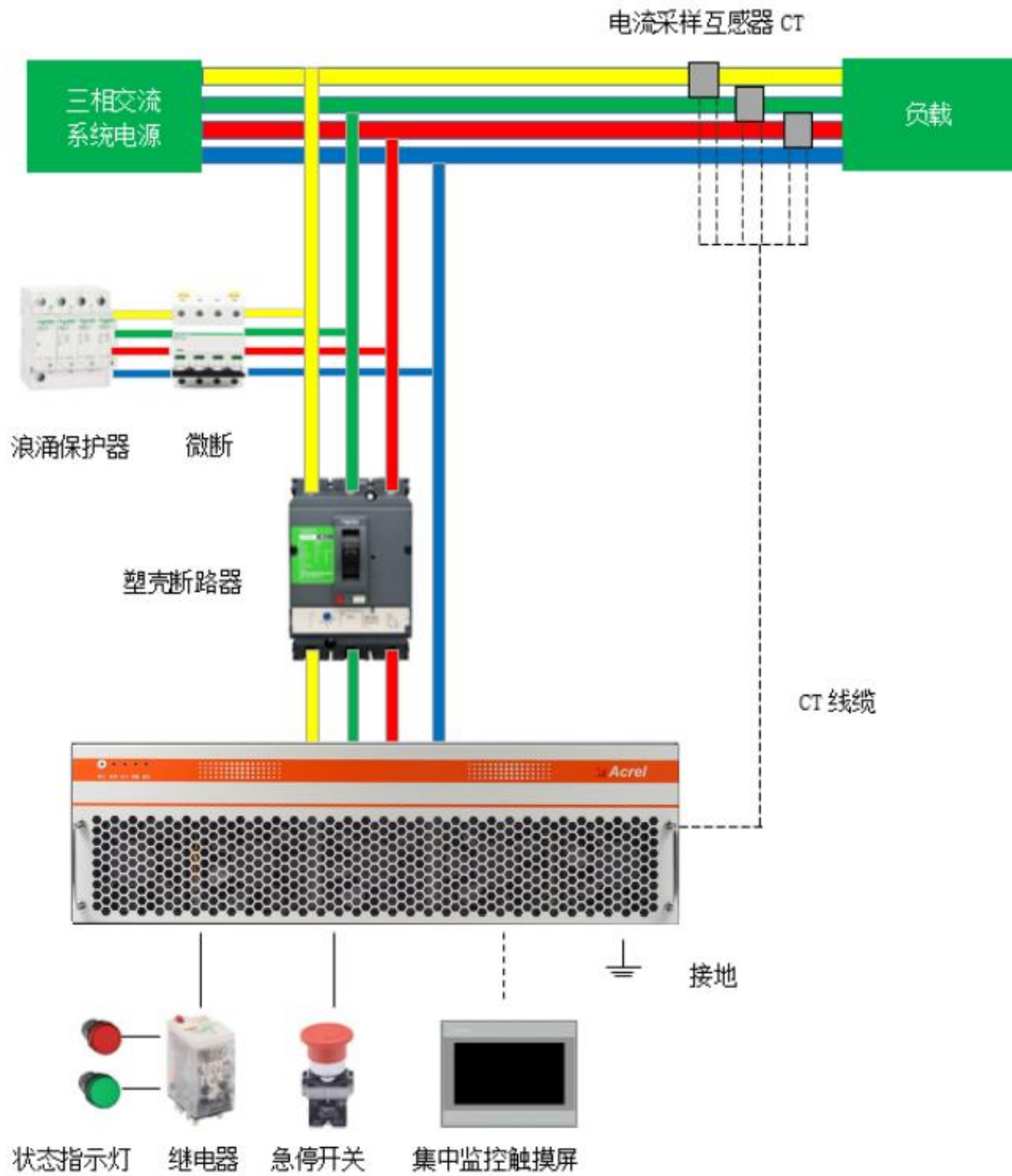
图5-1 ANSVG-G-A单模块系统连接图
