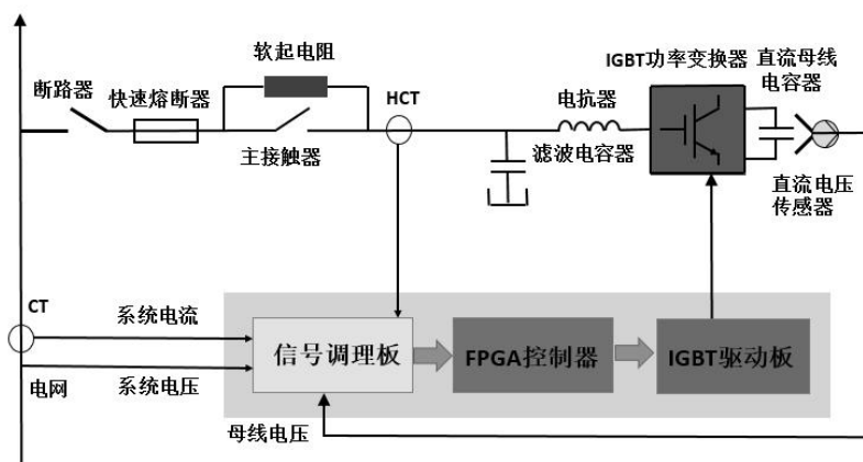
图3-2 ANSVG-G-A 内部控制原理图
