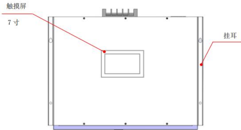
图4-9 75kvar-37.5A/100kvar-50A A壁挂式模块正面
