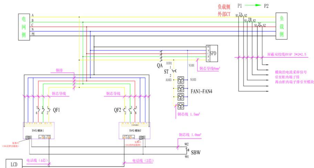
图 6-14 立柜式安装典型接线示意图
