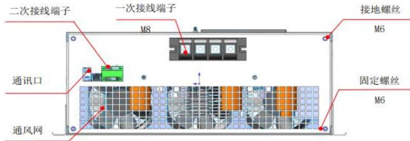
图4-15 50kvar-25A壁挂式模块顶部
