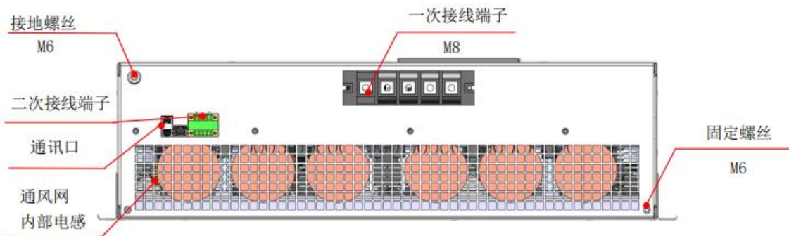
图4-10 75kvar-37.5A/100kvar-50A壁挂式模块顶部
