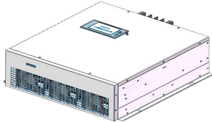
图4-13 50 kvar-25A壁挂式模块外观
