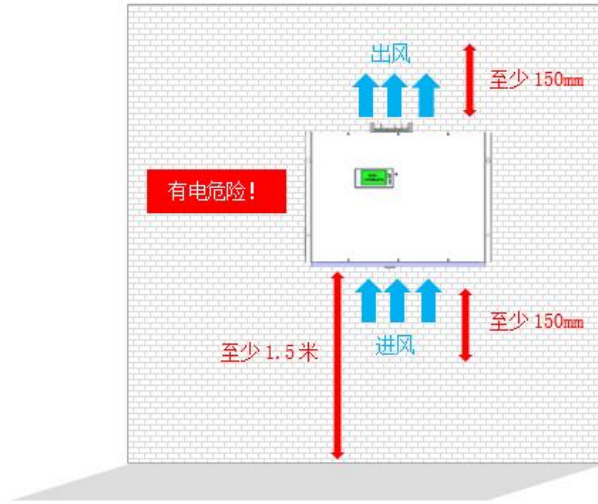
图6-3 立柜式安装空间要求示意图
