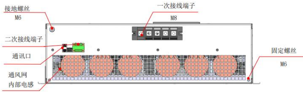
图4-10 150A/100A壁挂式模块顶部
