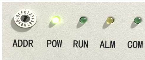
图4-26 拨码开关及状态指示灯示意图
