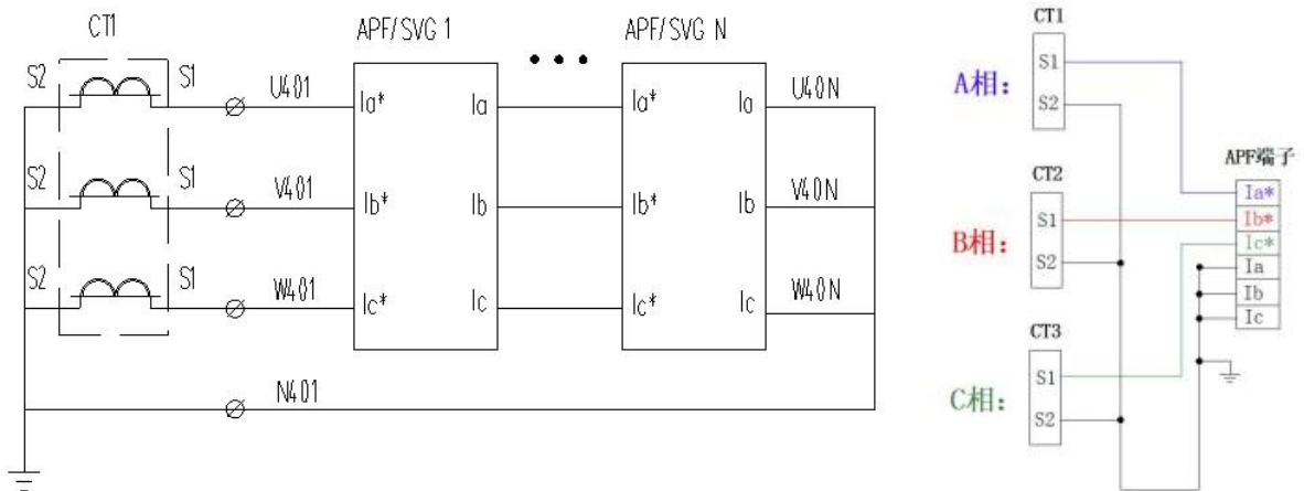
图 6-19 互感器电流采样（负载侧单 CT）回路接线示意图
