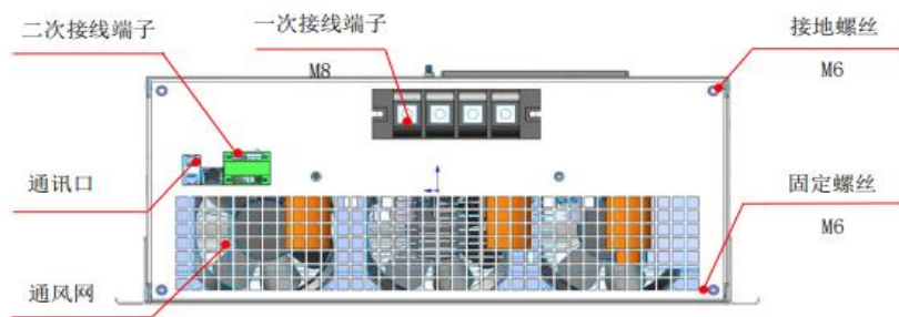
图4-15 50A/75A壁挂式模块顶部
