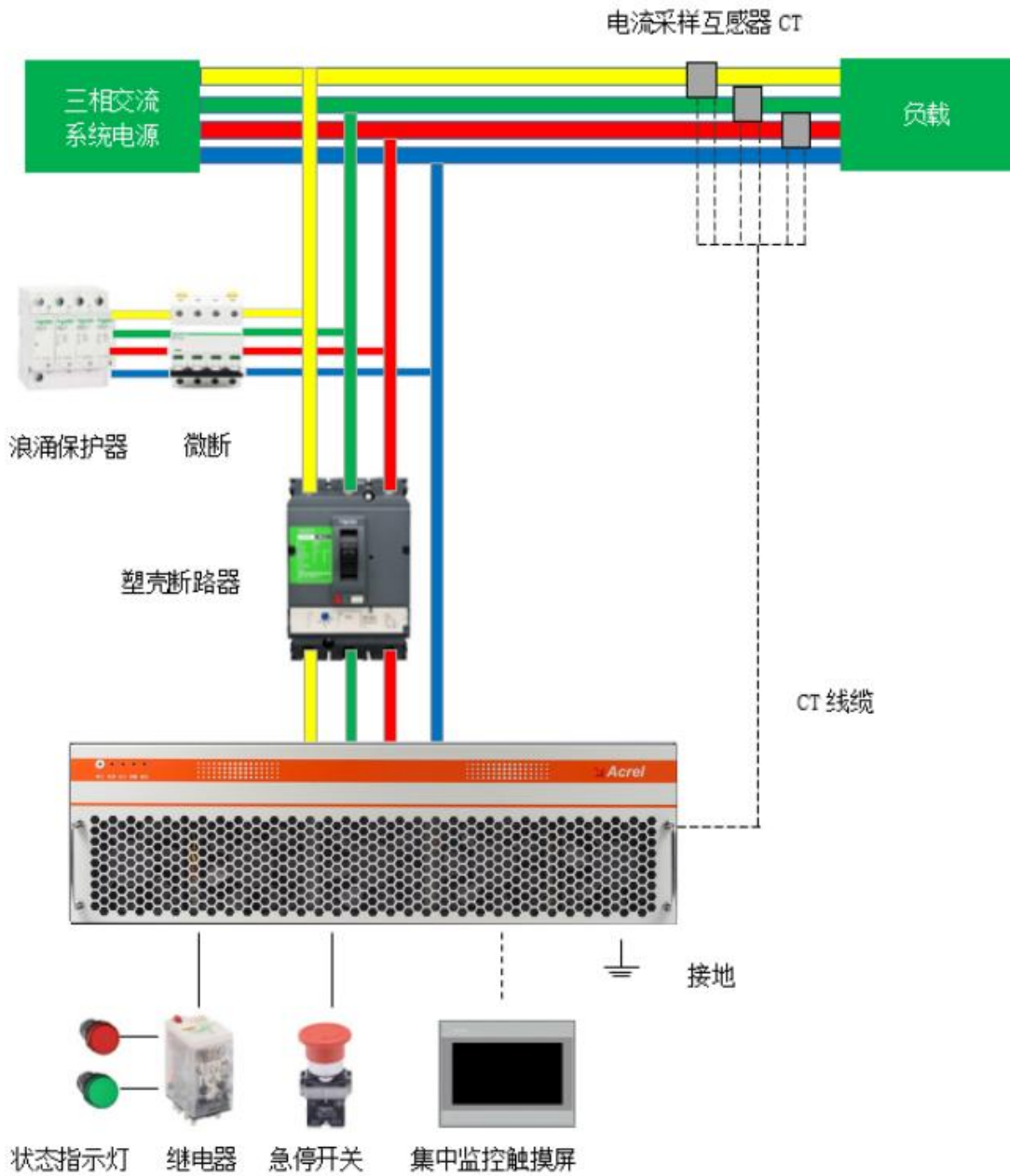
图5-1 ANAPF单模块系统连接图
