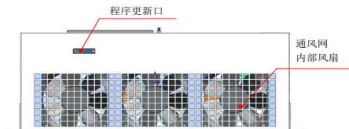
图4-16 50A/75A壁挂式模块底部
