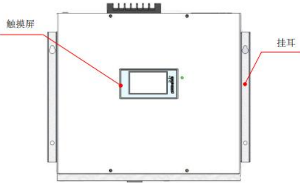
图4-19 30A壁挂式模块正面
