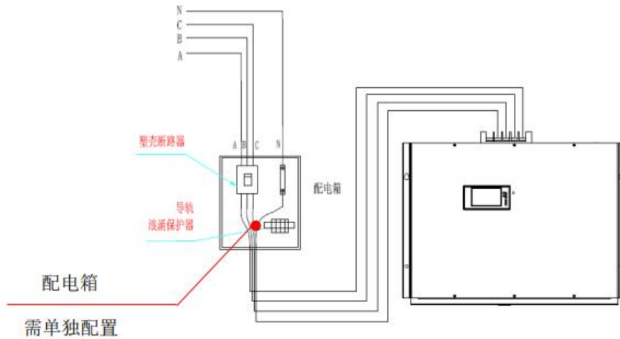
图6-13 壁挂式模块安装示意图（二）
