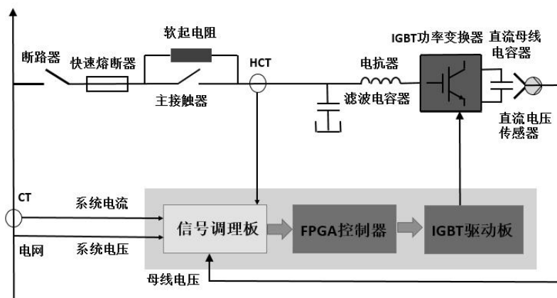
图3-2 ANAPF 内部控制原理图
