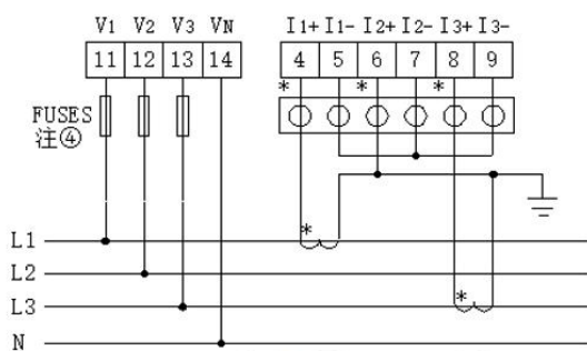
3P4L/2CT (仪表设置为3P4L) 注②
