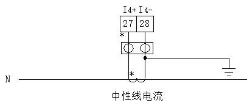
中性线电流
