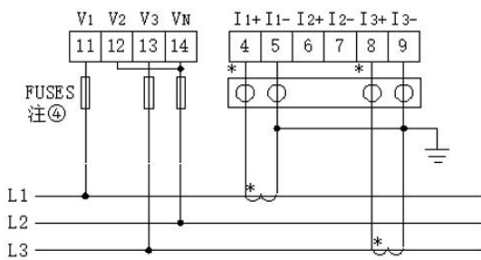
3P3L/2CT (仪表设置为3P3L-2CT)
