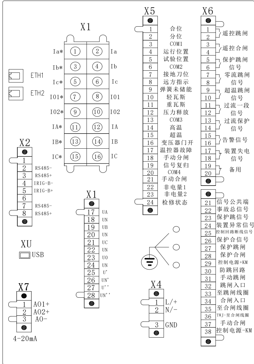
图 2.13 AM5SE-T 电气接线图
