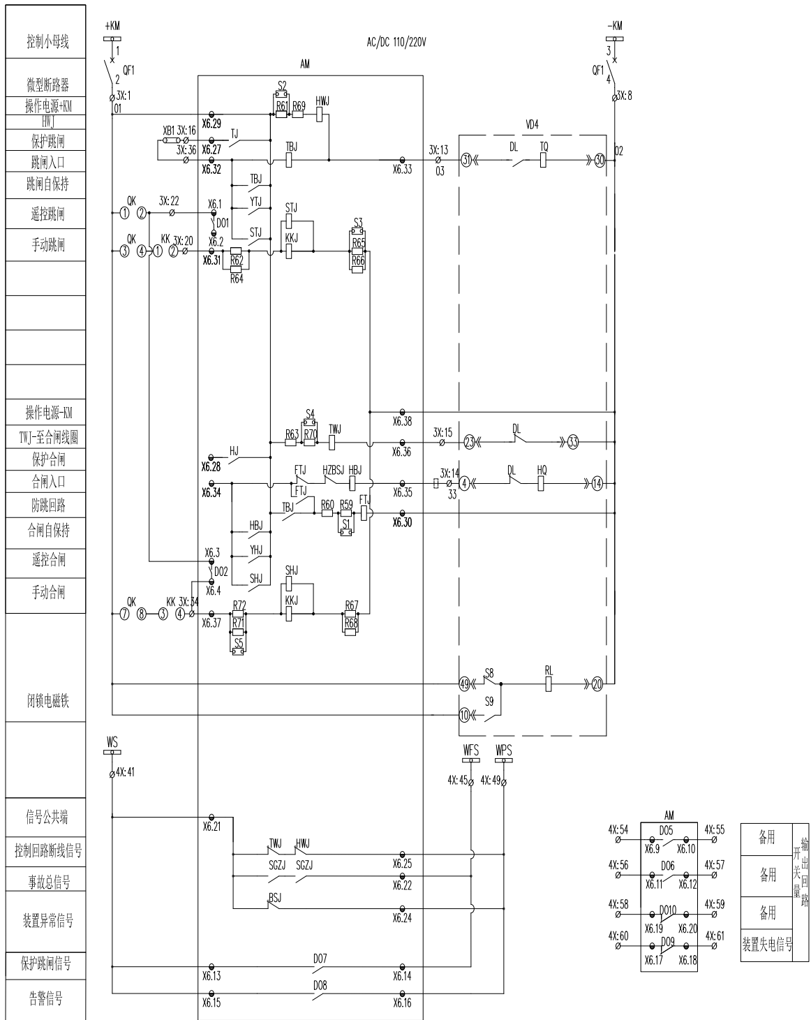
图 6.32 AM5SE-MD 二次原理图 (三)
