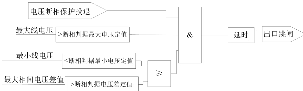
图 3.19 电压断相保护逻辑
