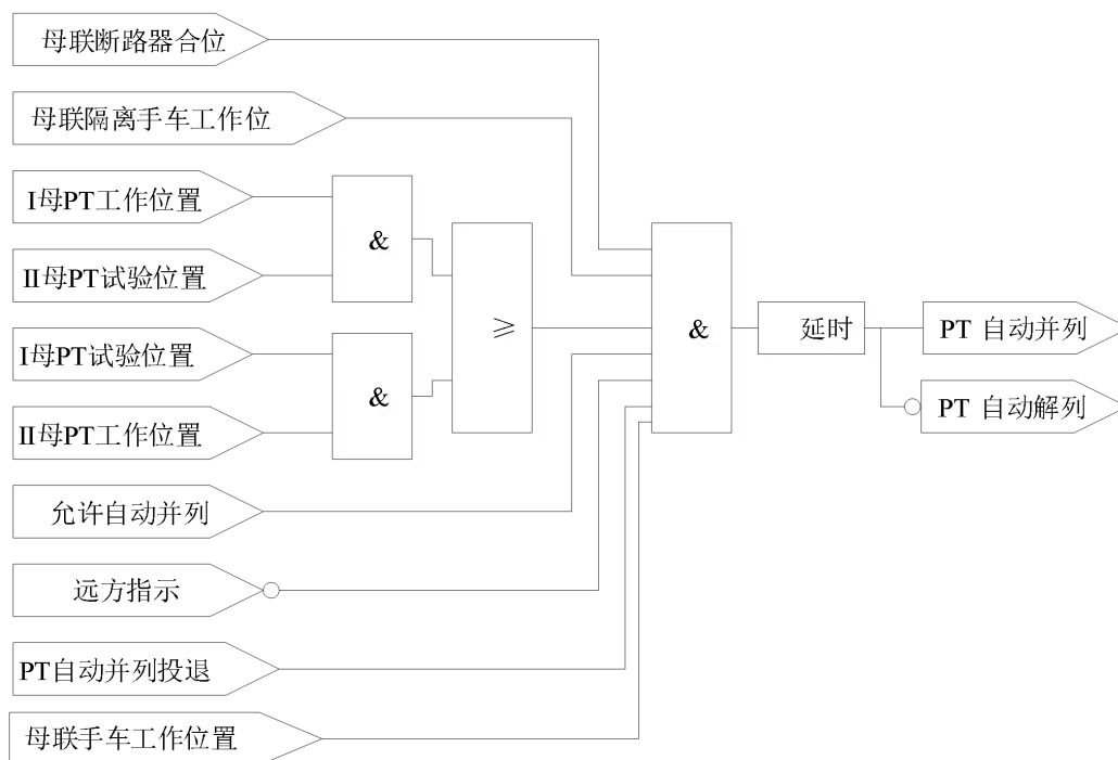
图 9.3 PT 自动并列解列逻辑
