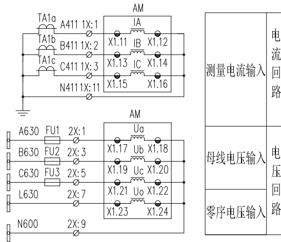
图 13.2 AM5SE-K 二次原理图（一）
