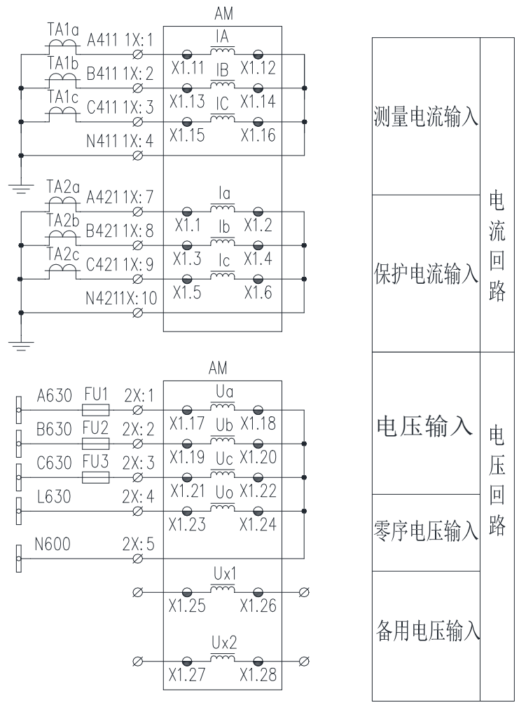
图 14.8 AM5SE-FE 二次原理图 (一)
