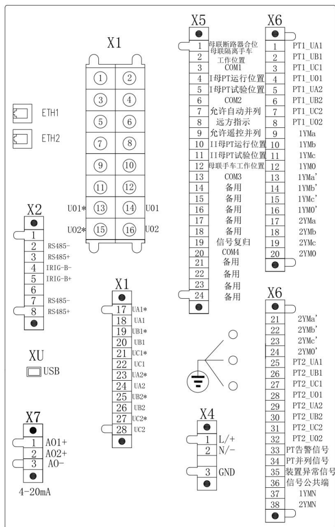
图 9.19 AM5SE-UB 电气接线图
