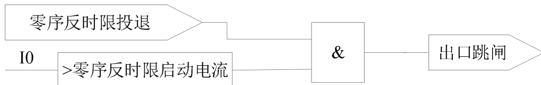
图 8.5 零序反时限过流保护逻辑
