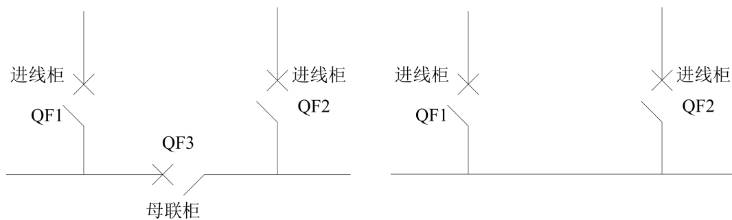
图 4.5 (a) 两进线一母联
