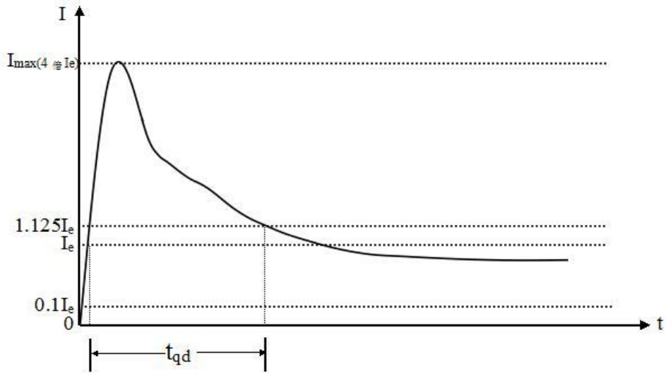
图 6.14 异步电动机启动电流特性图
