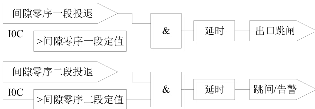
图 8.10 两段式间隙零序过流保护逻辑
