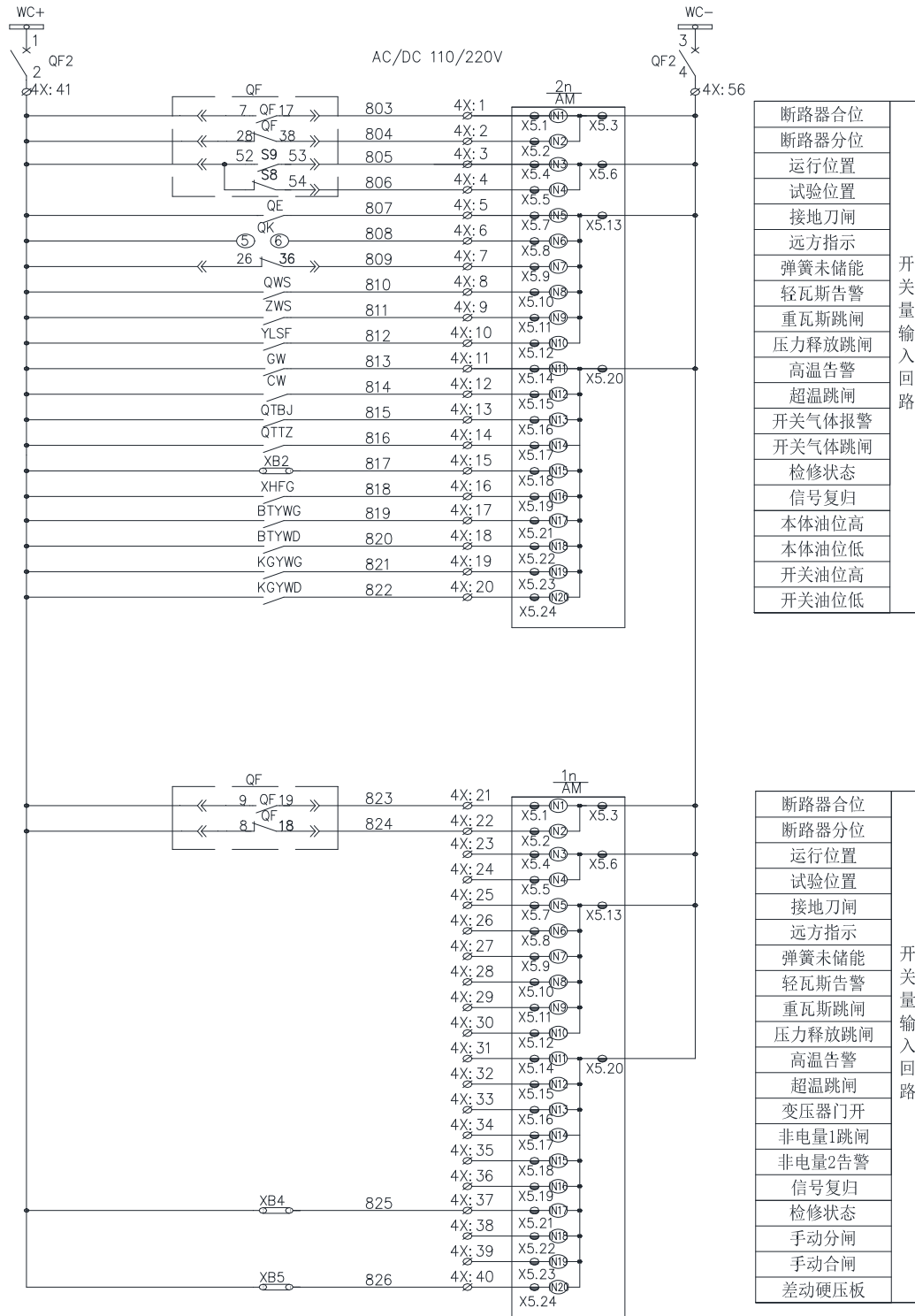
图 8.20 AM5SE-TB 二次原理图（二）
