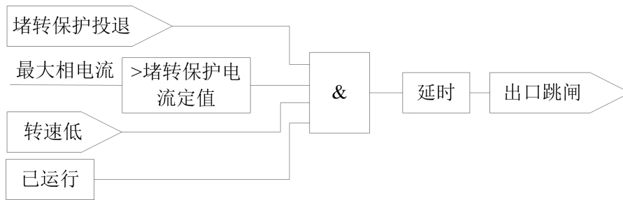
图 3.8 堵转保护逻辑
