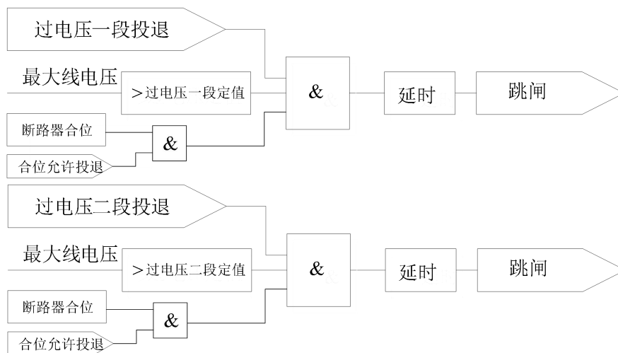
图 15.3 过电压保护逻辑
