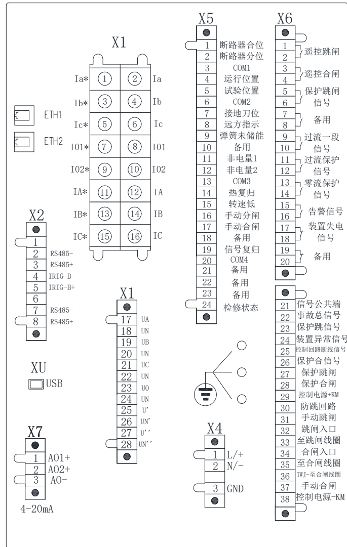
图 3.24 AM5SE-M 电气接线图
