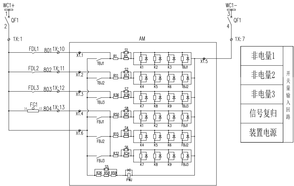
图 12.3 AM5SE-FD 二次原理图 (一)
