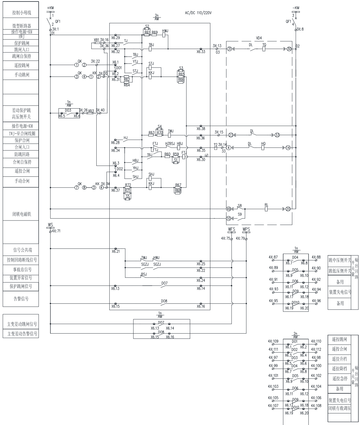
图 10.9 AM5SE-D3 二次原理图（三）
