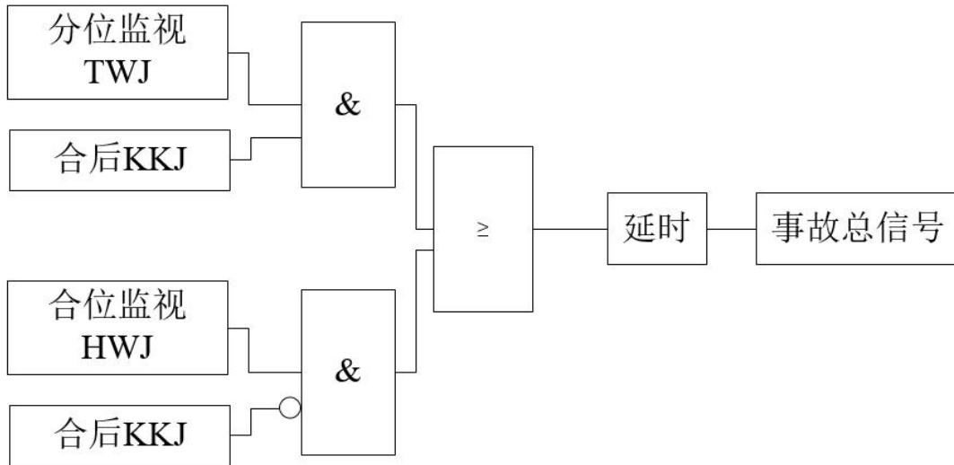
图 11.9 事故总信号逻辑
