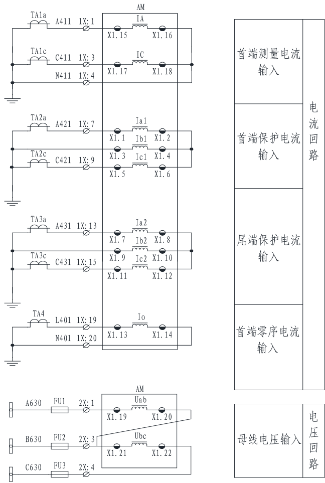
图 6.29 2PT 2CT 接线方法
