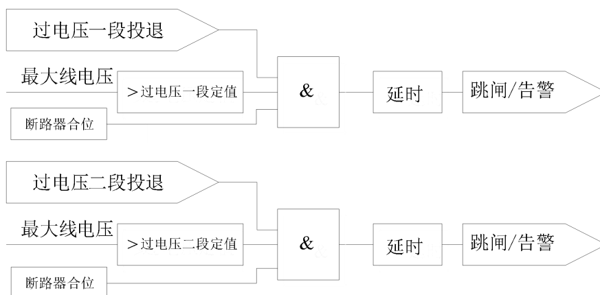
图 11.4 过电压保护逻辑
