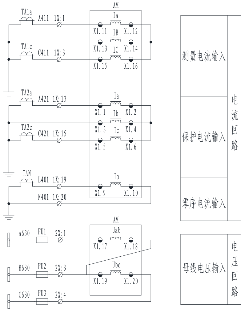
图 5.16 2PT 2CT 接线方法
