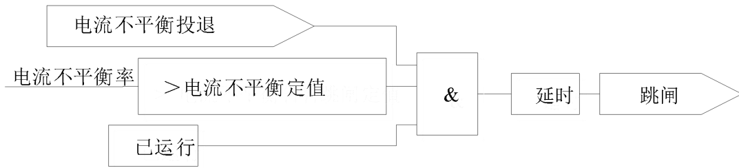
图 6.16 不平衡电流保护逻辑
