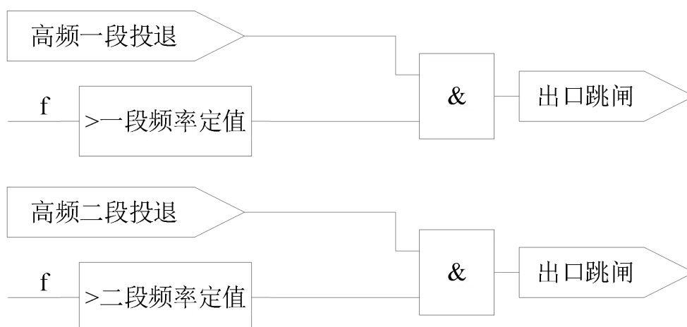
图 15.1 高频保护逻辑
