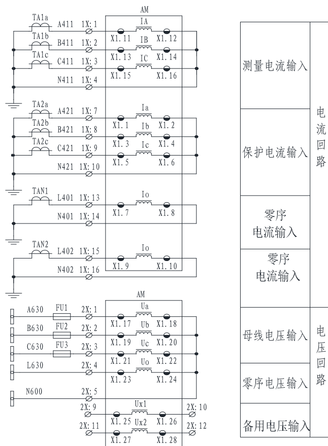
图 3.26 AM5SE-M 二次原理图（一）
