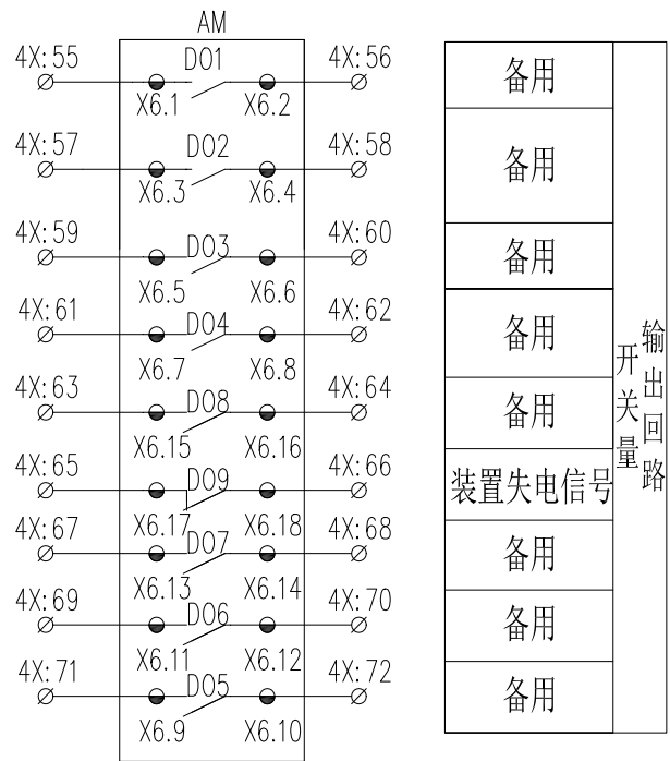
图 13.4 AM5SE-K 二次原理图 (三)
