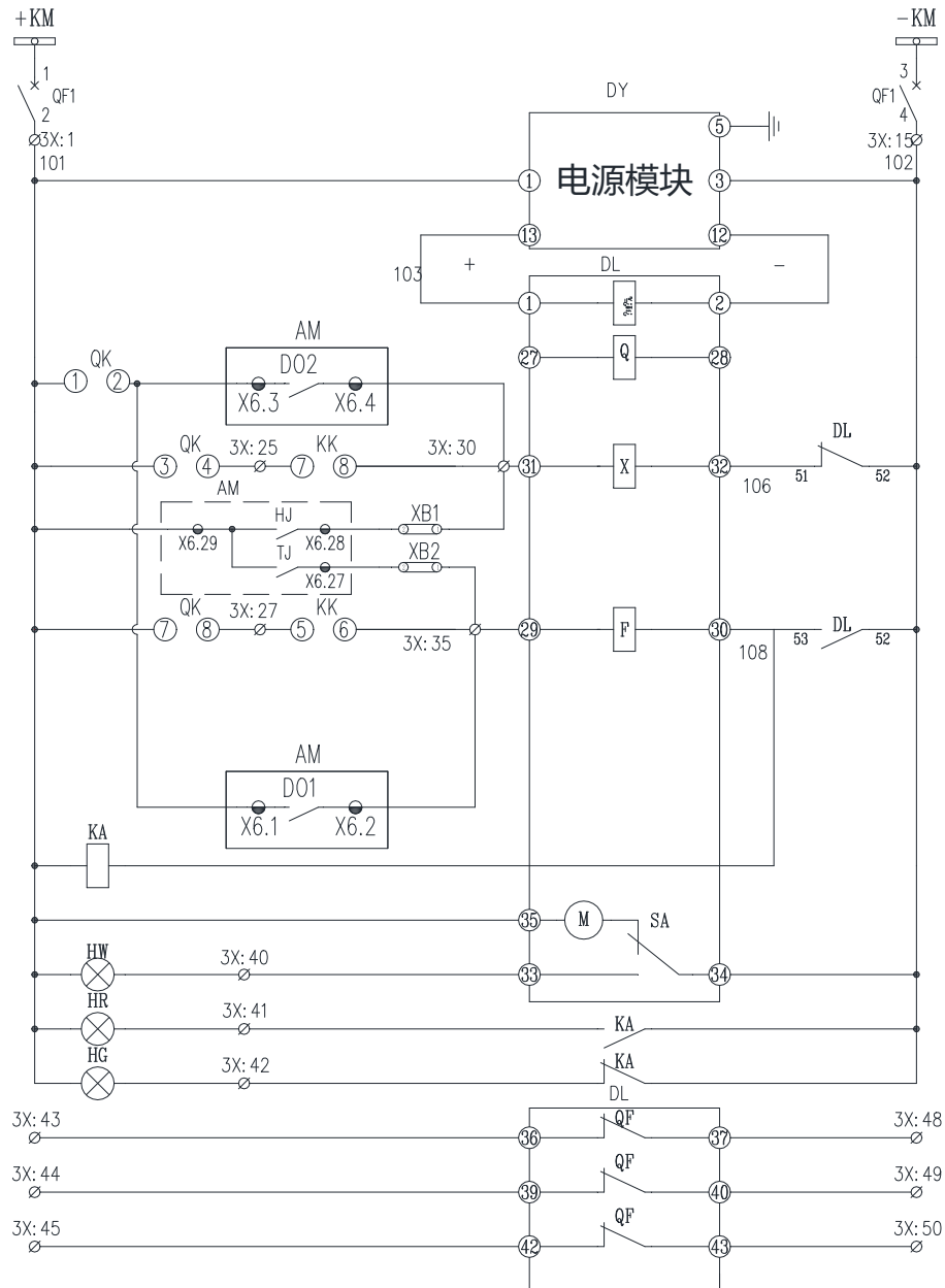
图 11.19 AM5SE-IS 二次原理图 (低压) (五)
