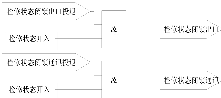
图 3.23 检修状态闭锁逻辑
