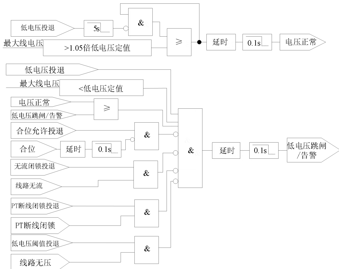
图 6.17 低电压保护逻辑
