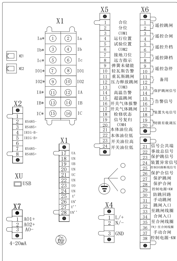
图 8.17 AM5SE-TB 电气接线图
