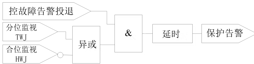
图 6.26 控制回路断线告警逻辑
