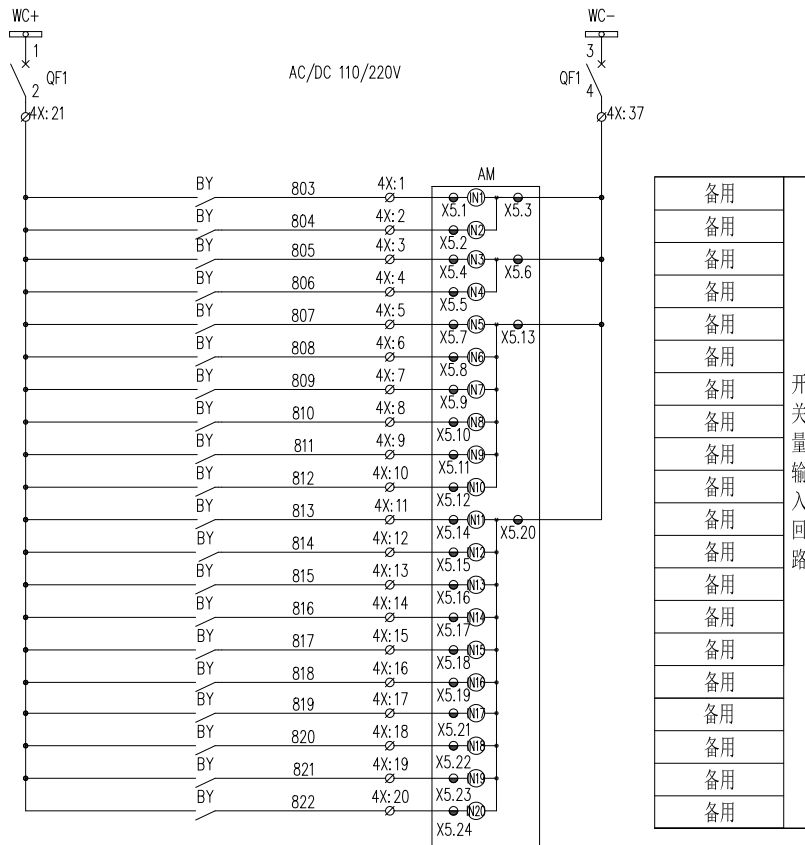
图 13.3 AM5SE-K 二次原理图（二）
