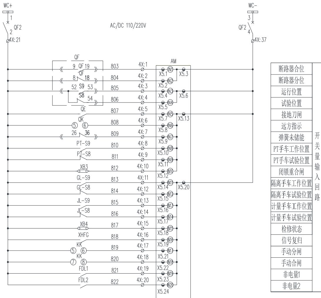
图 1.21 AM5SE-F 二次原理图（二）
