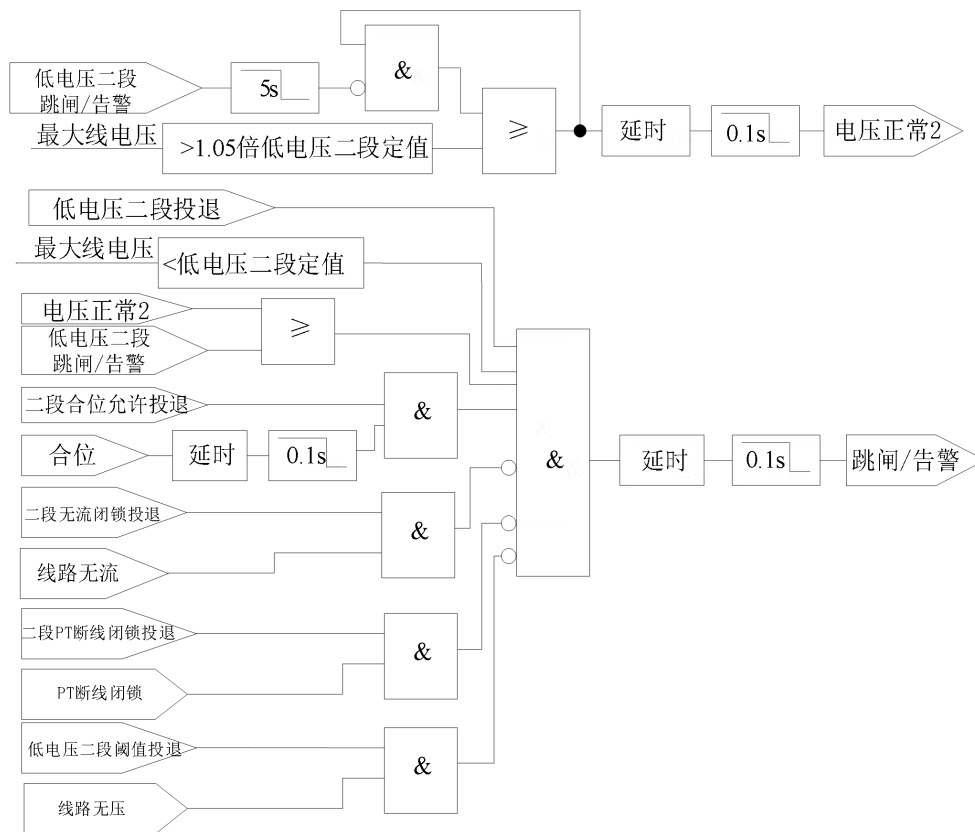
图 11.2 低电压保护逻辑
