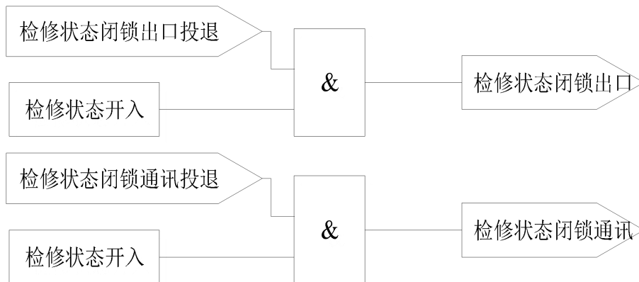
图 6.27 检修状态闭锁逻辑
