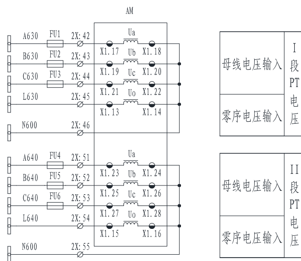
图 9.21 AM5SE-UB 二次原理图 (一)
