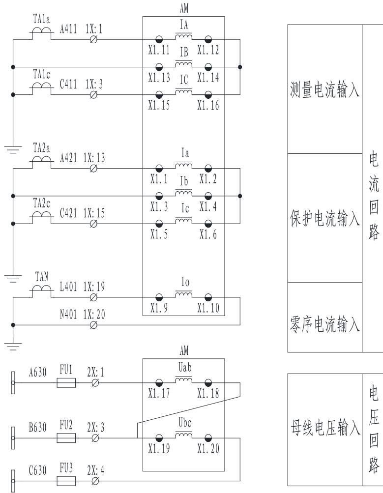
图 15.6 2PT 2CT 接线方法
