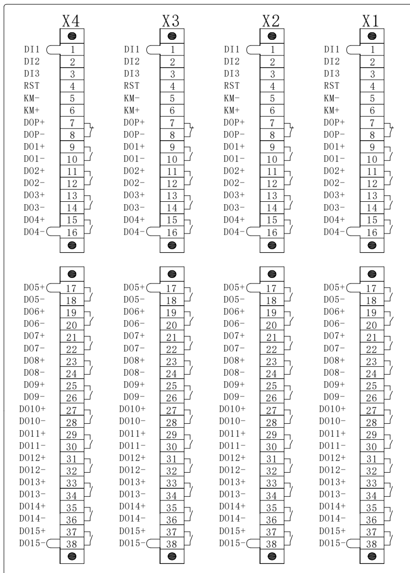
图 12.1 AM5SE-FD 电气接线图
