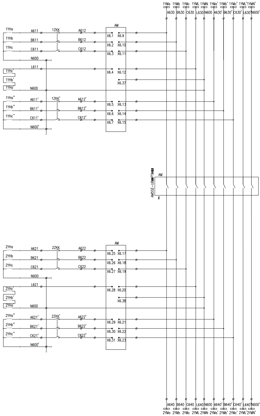
图 9.23 AM5SE-UB 二次原理图 (三)
