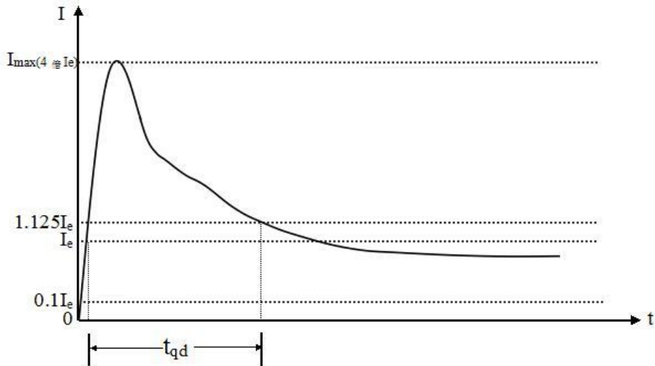
图 3.9 异步电动机启动电流特性图
