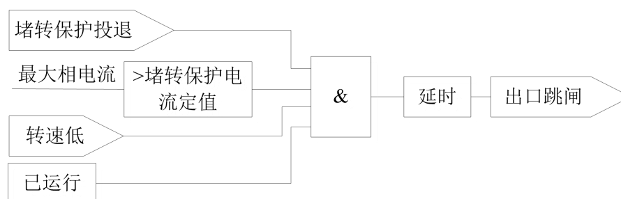
图 6.12 堵转保护逻辑
