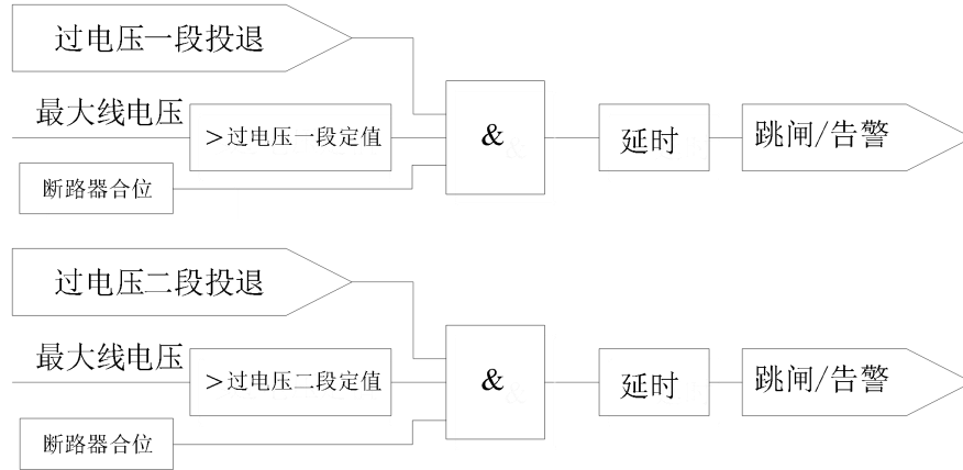
图 14.3 过电压保护逻辑
