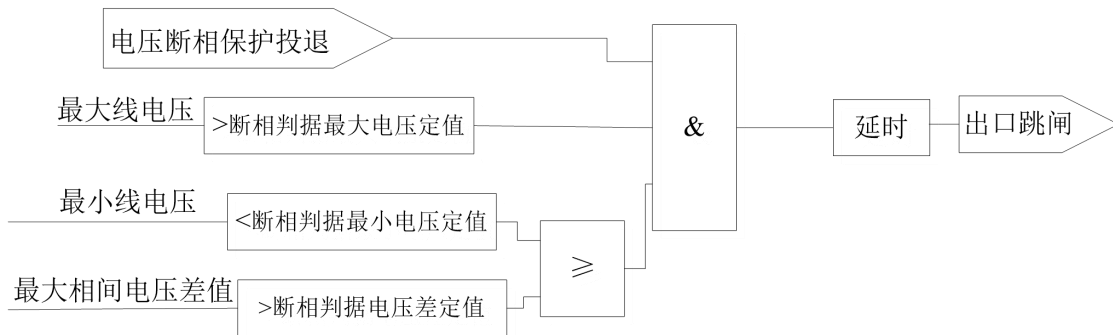
图 6.22 电压断相保护逻辑
