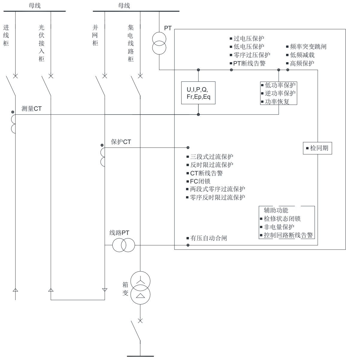
图 11.12 高压并网柜功能接线图
