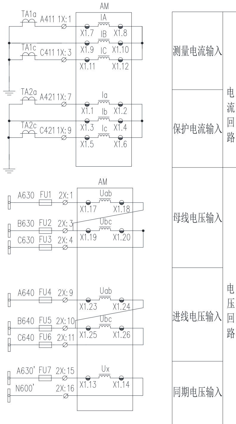
图 11.11 2PT 2CT 接线方法
