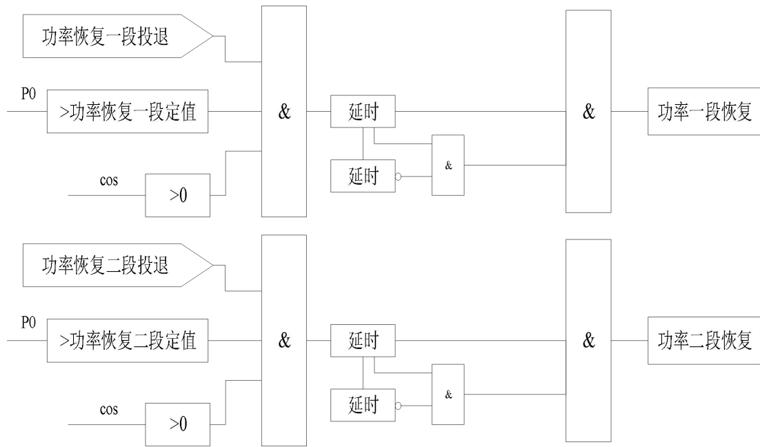
图 11.7 功率恢复保护逻辑
