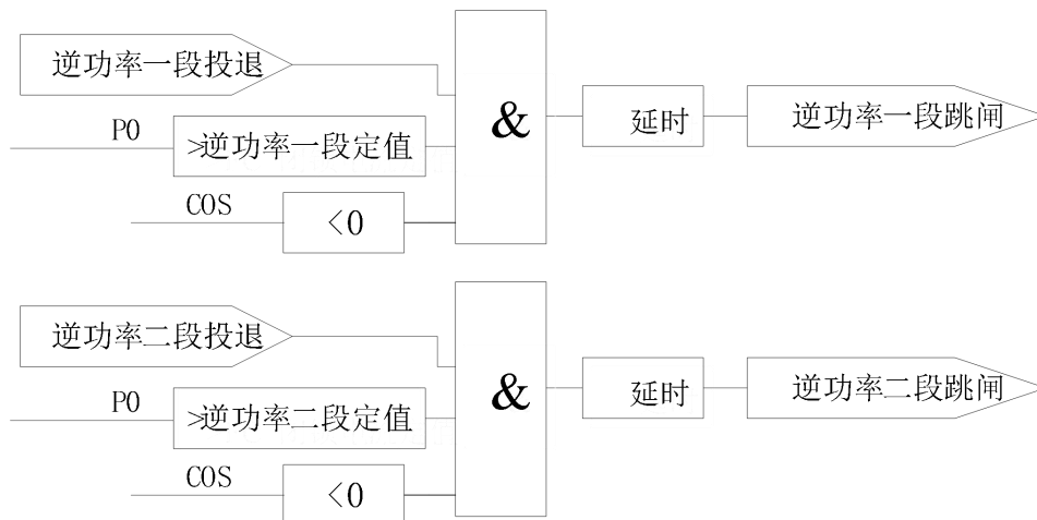
图 11.3 逆功率保护逻辑
