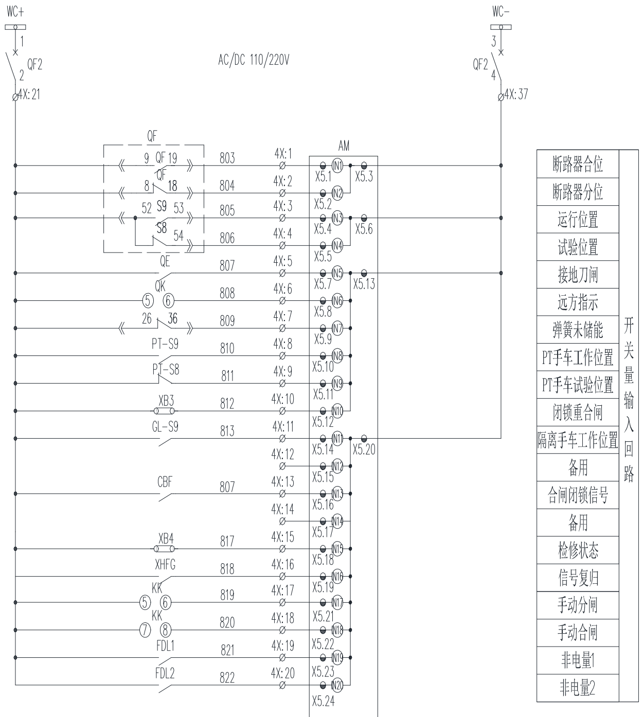
图 11.16 AM5SE-1S 二次原理图（高压）（二）
