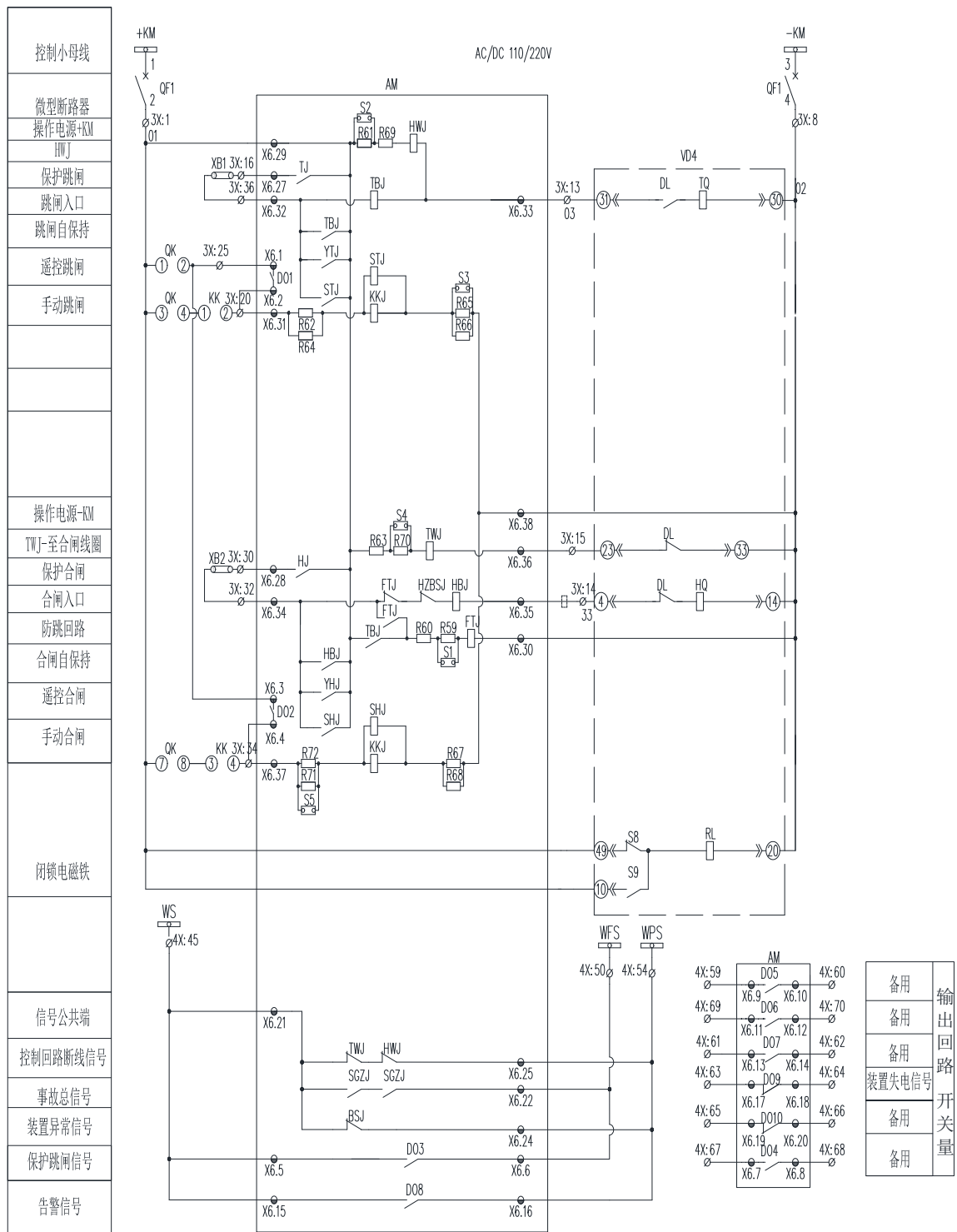
图 15.10 AM5SE-FA 二次原理图 (三)
