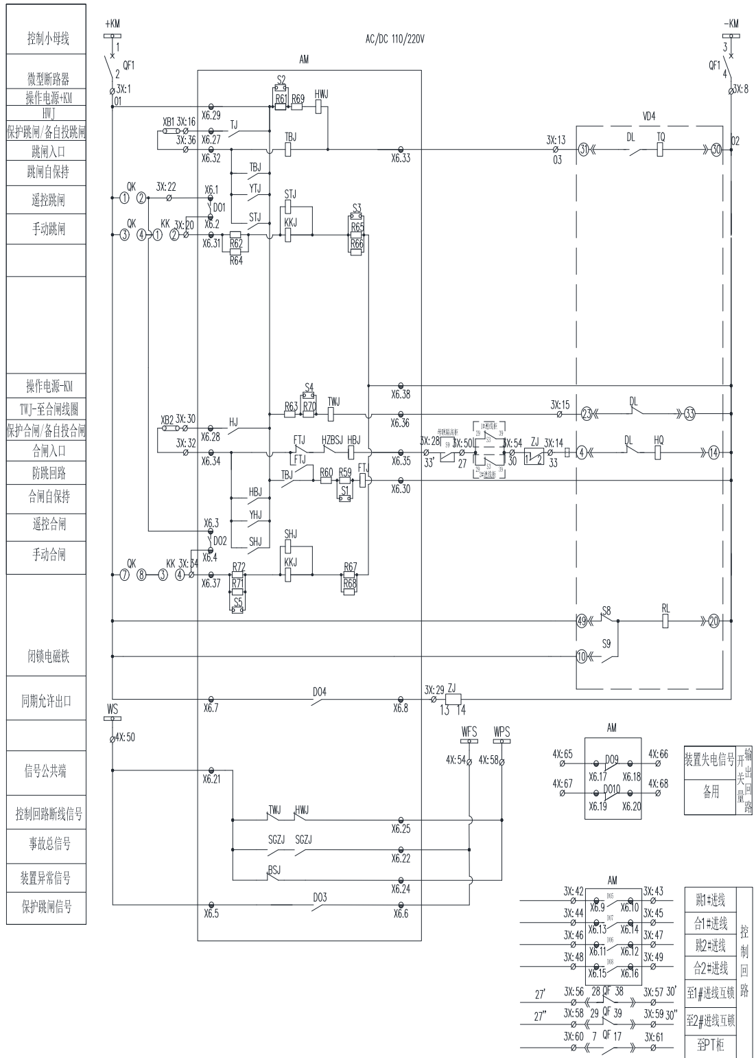
图 4.16 AM5SE-B 备自投二次原理图（三）
