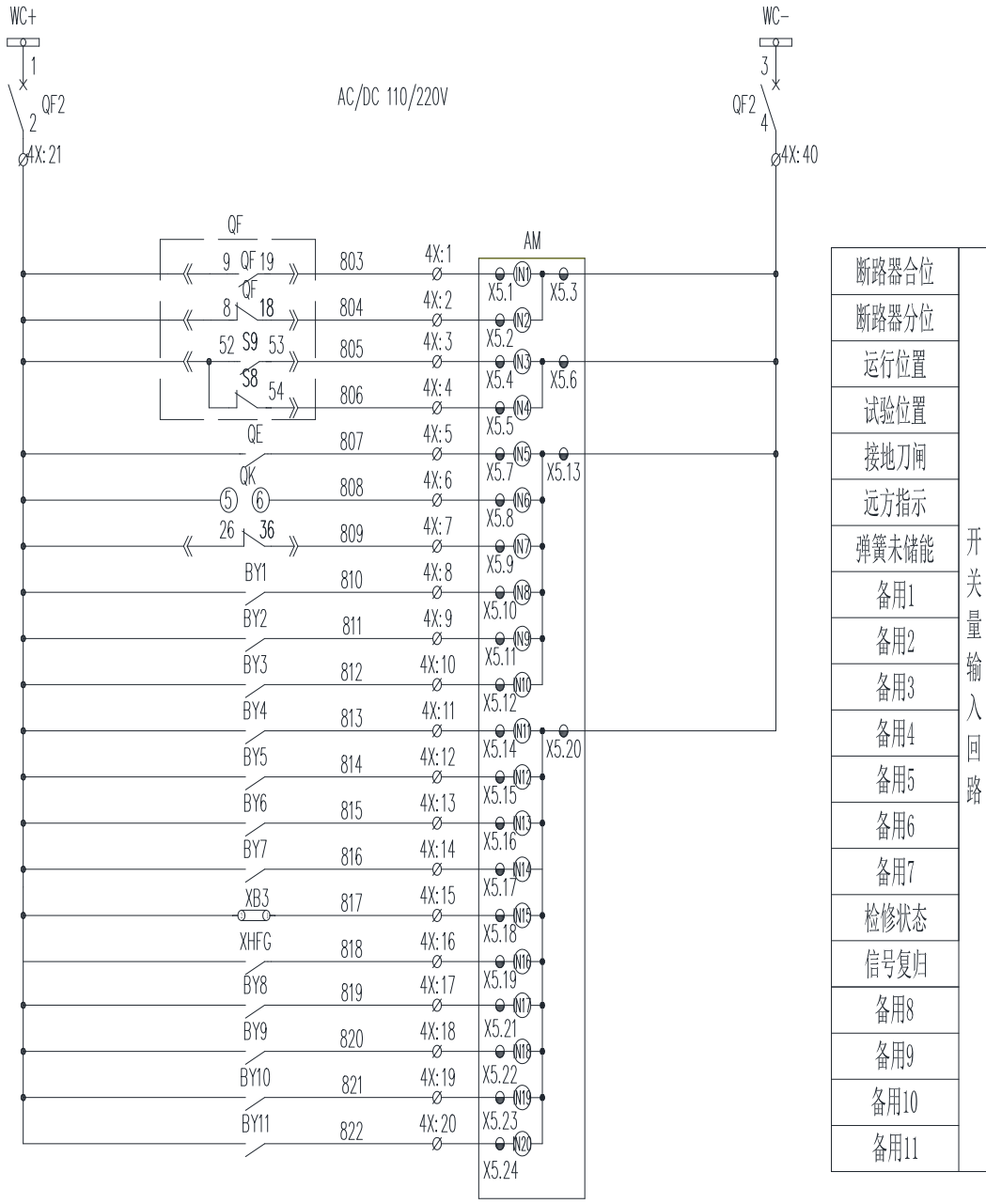
图 15.9 AM5SE-FA 二次原理图（二）
