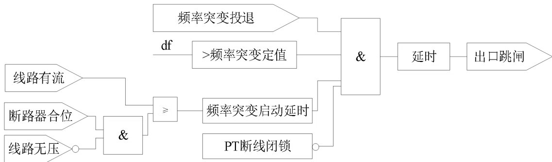
图 14.4 频率突变跳闸逻辑
