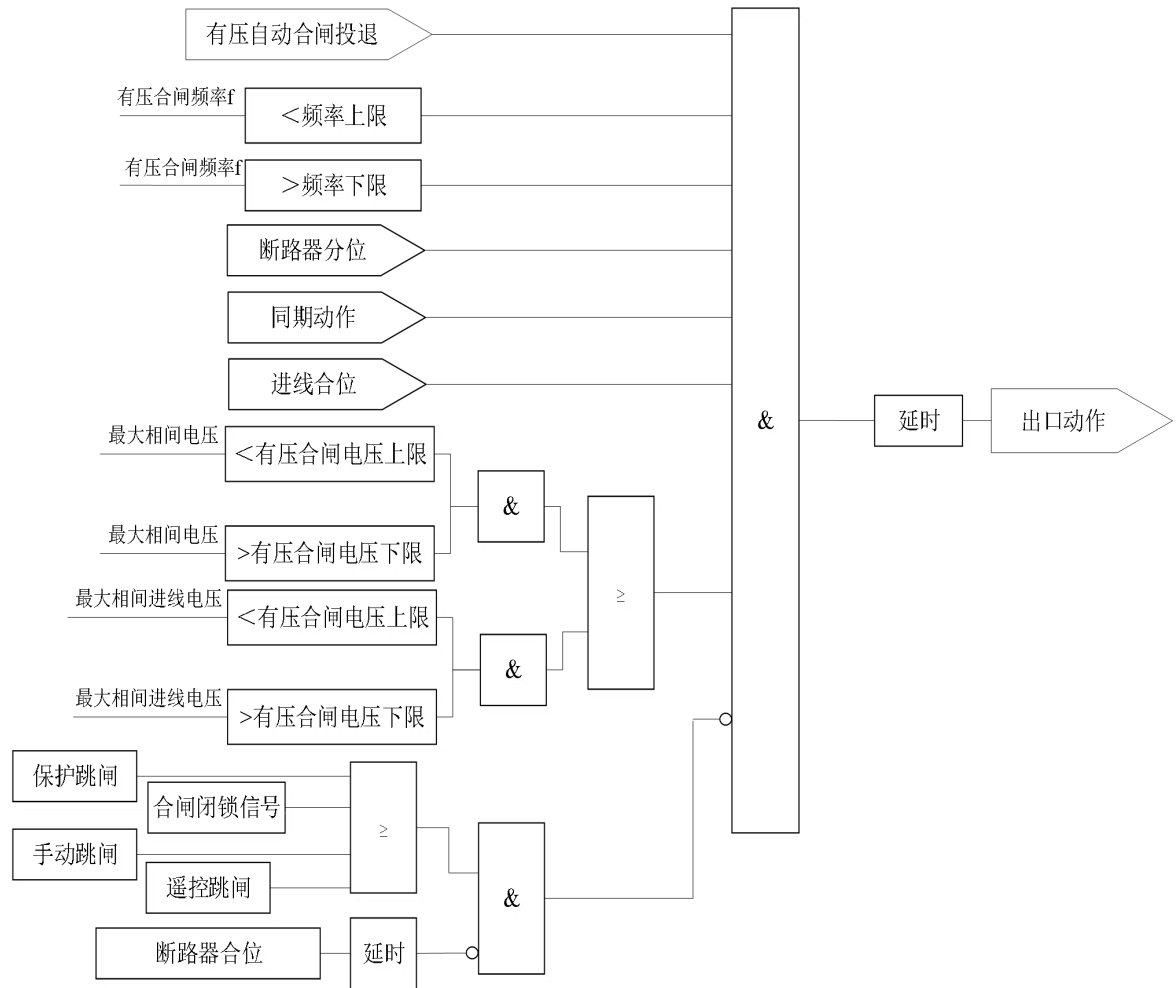
图 11.6 有压自动合闸逻辑
