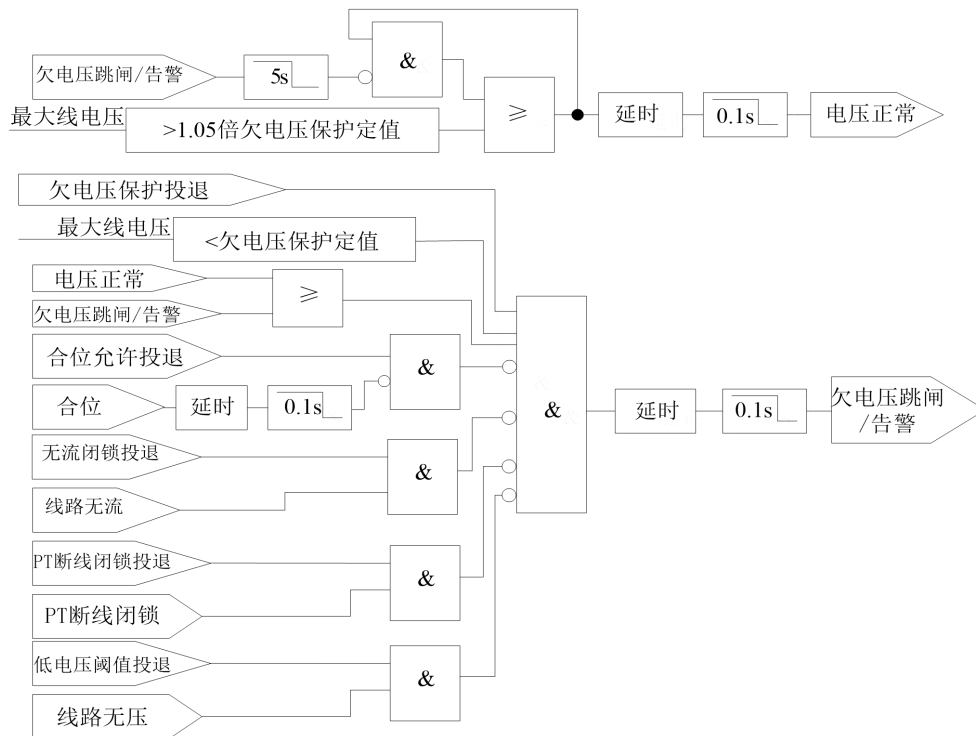
图 5.4 欠电压保护逻辑
