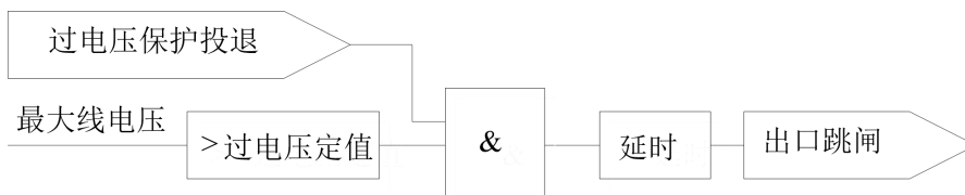
图 3.20 过电压保护逻辑
