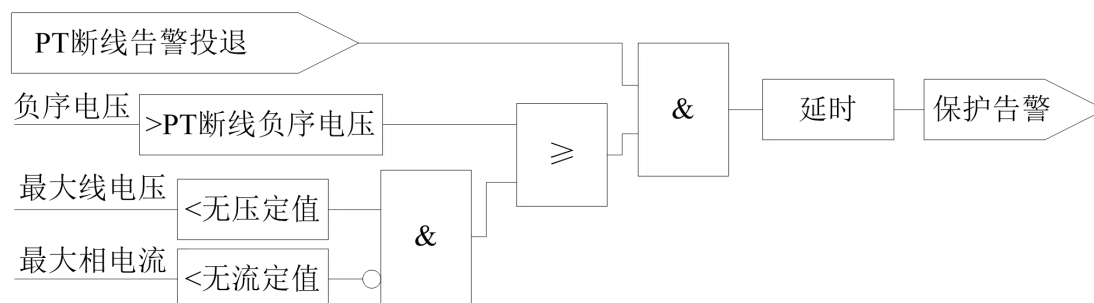
图 5.10 PT 断线告警逻辑
