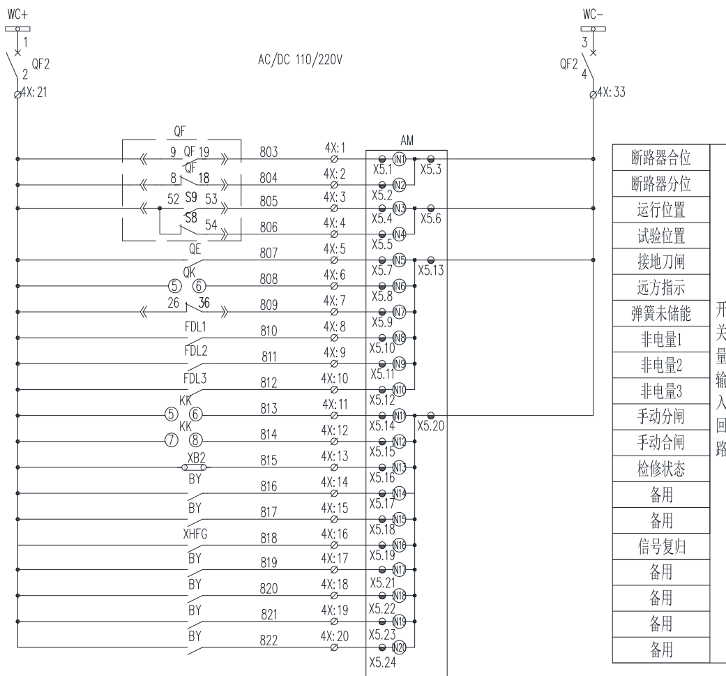
图 5.18 AM5SE-C 二次原理图 (二)
