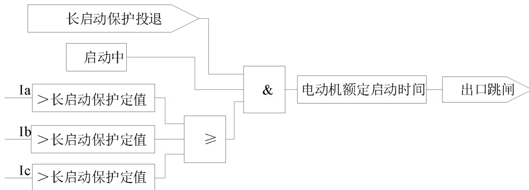
图 6.15 长启动保护逻辑
