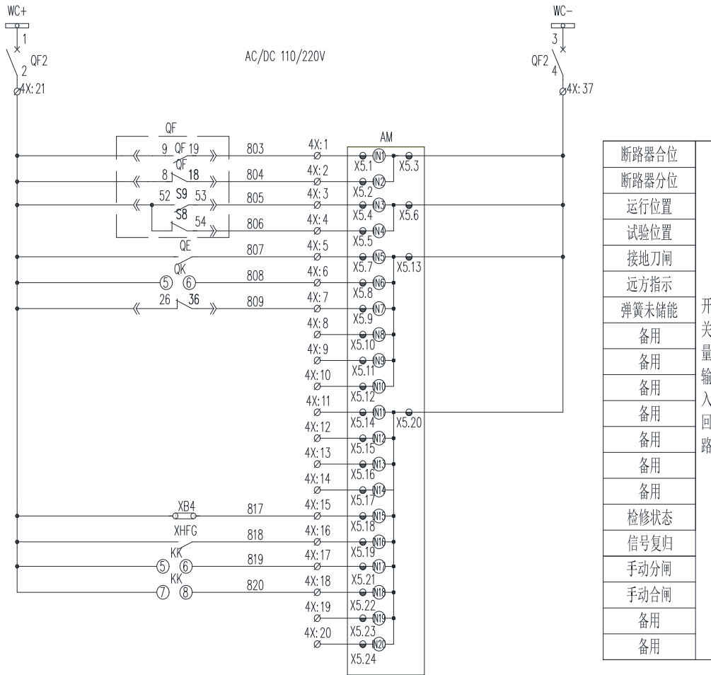
图 14.9 AM5SE-FE 二次原理图（二）
