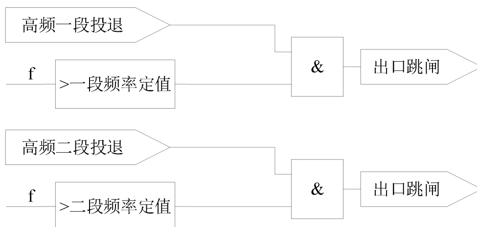
图 14.1 高频保护逻辑
