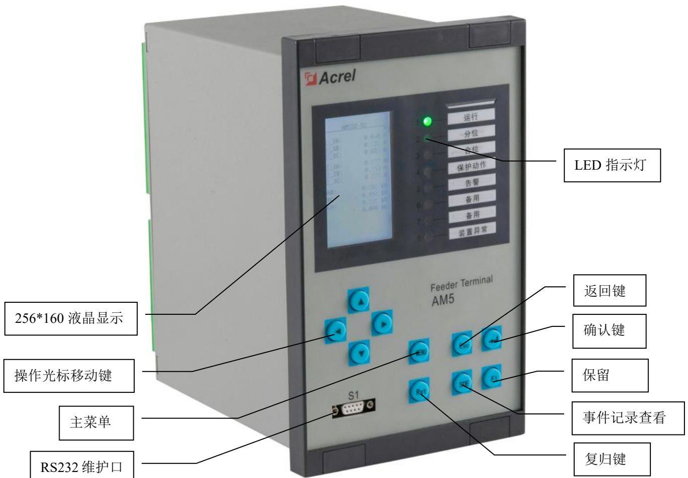
图 3.1 AM5SE 前面板
