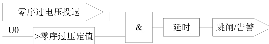
图 6.19 零序过压保护逻辑
