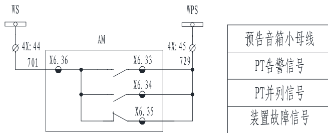
图 9.24 AM5SE-UB 二次原理图 (四)
