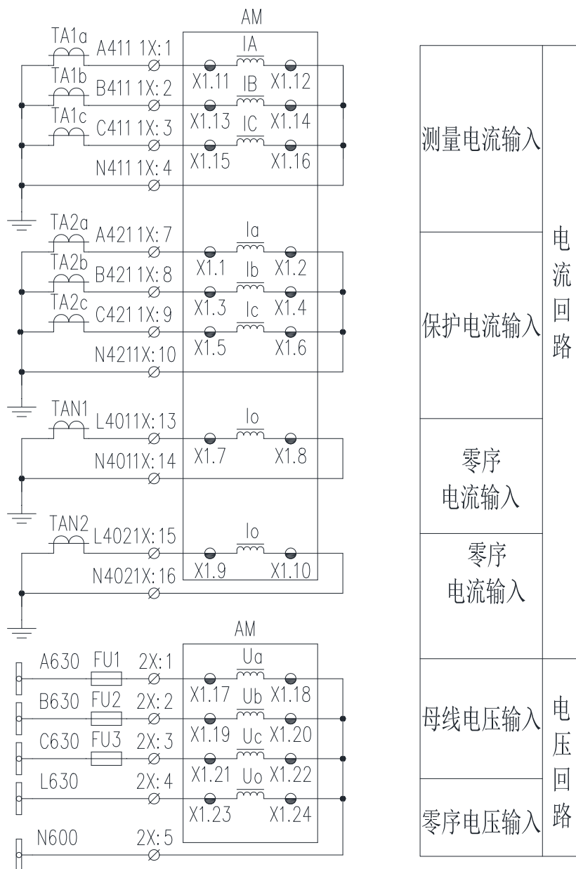
图 15.8 AM5SE-FA 二次原理图 (一)
