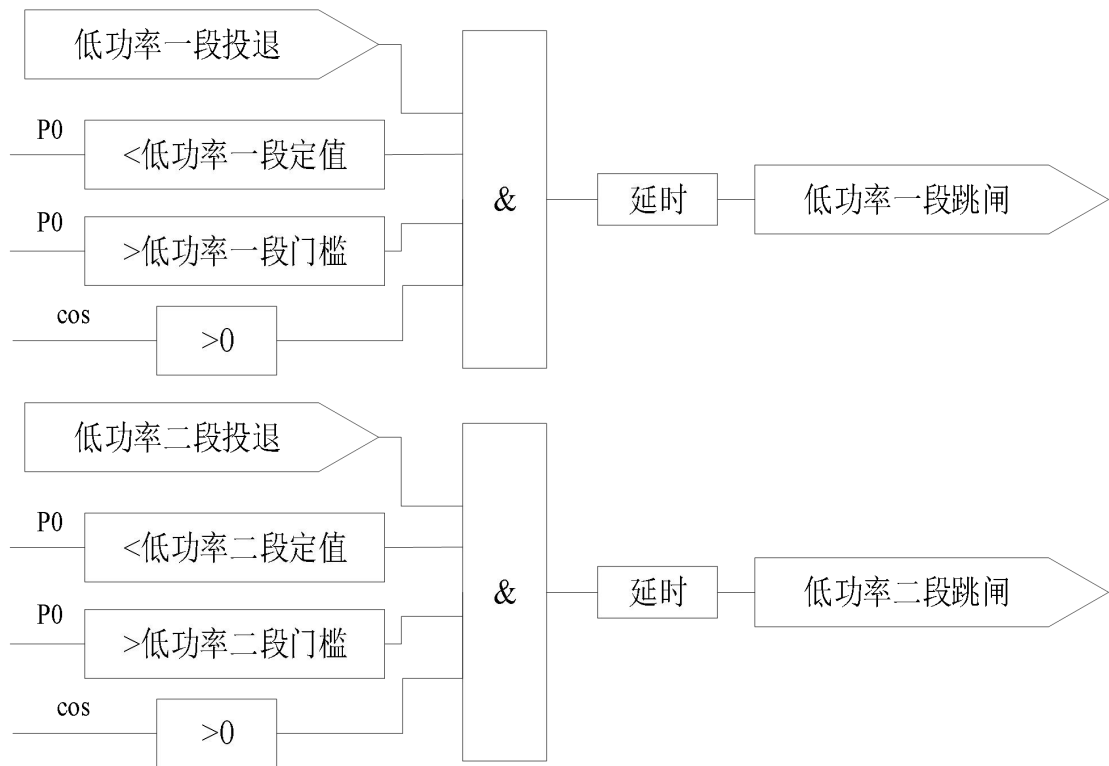
图 11.8 低功率保护逻辑
