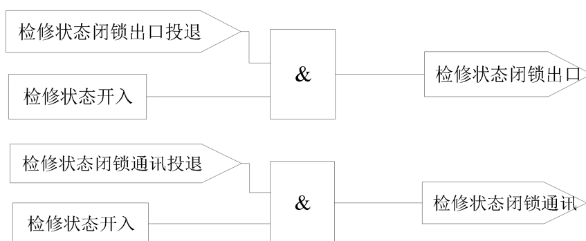
图 8.16 检修状态闭锁逻辑
