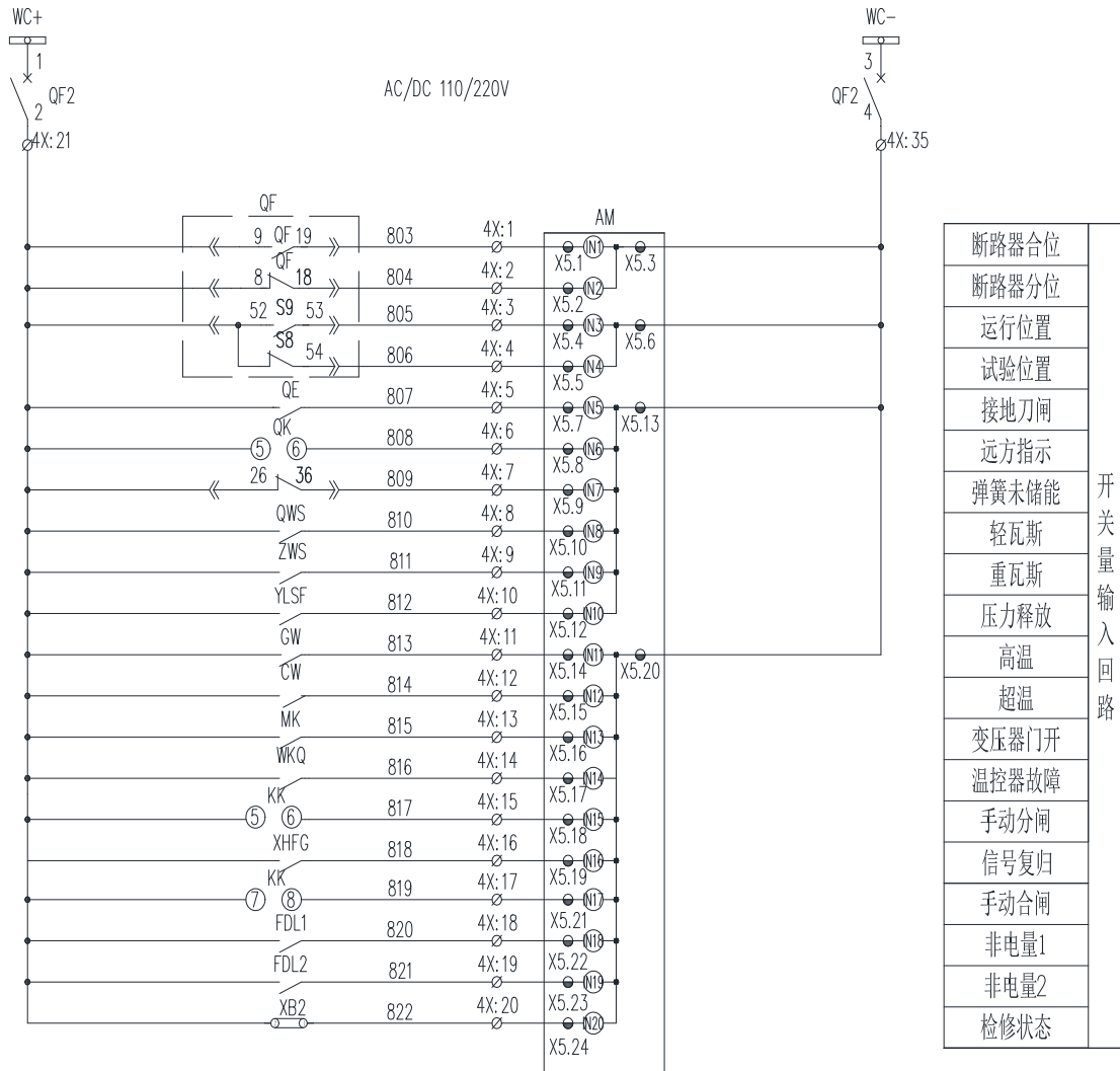
图 2.16 AM5SE-T 二次原理图 (二)
