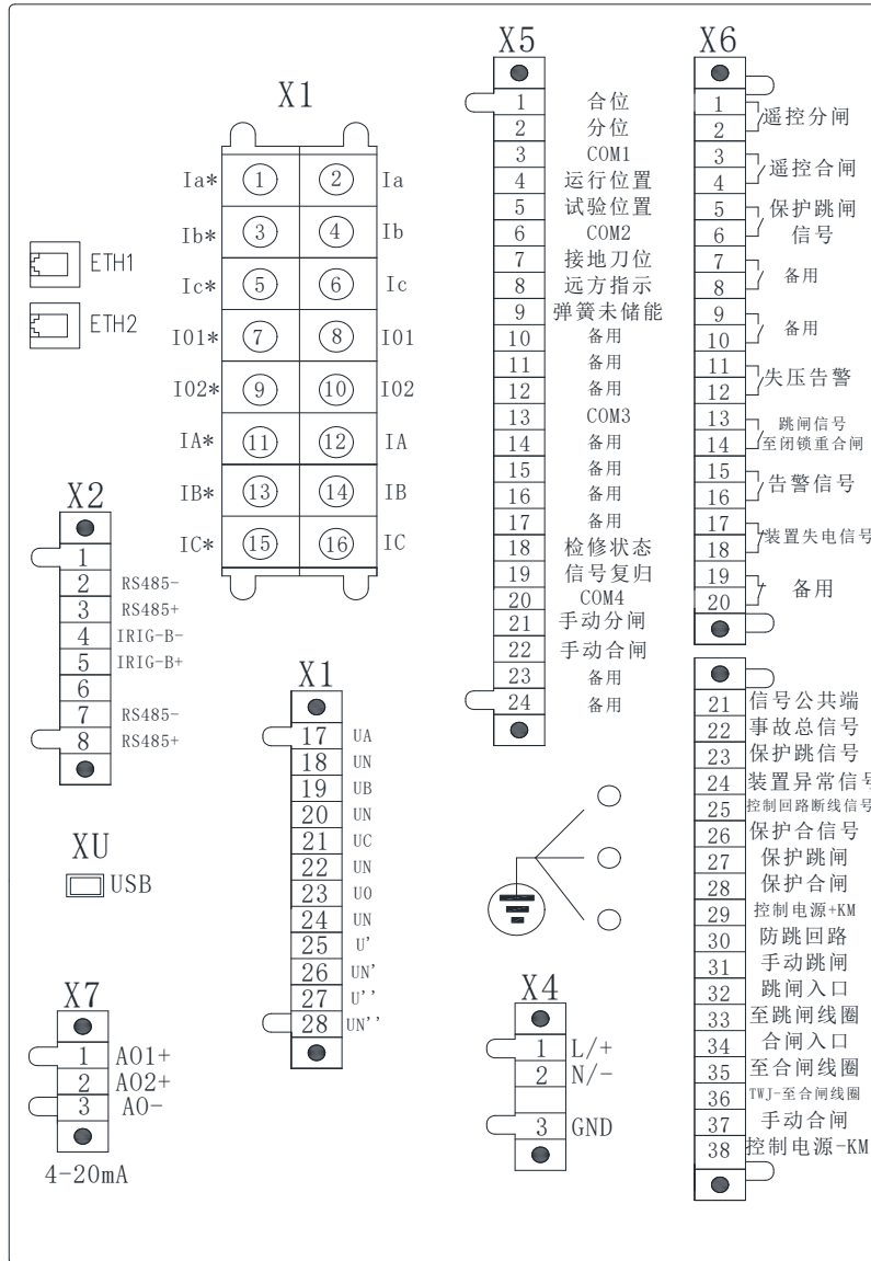
图 14.5 AM5SE-FE 电气接线图
