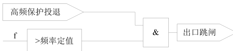
图 1.9 高频保护逻辑
