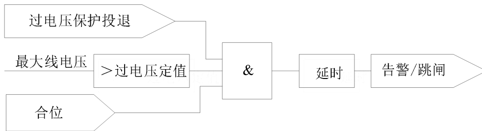
图 1.13 过电压保护逻辑
