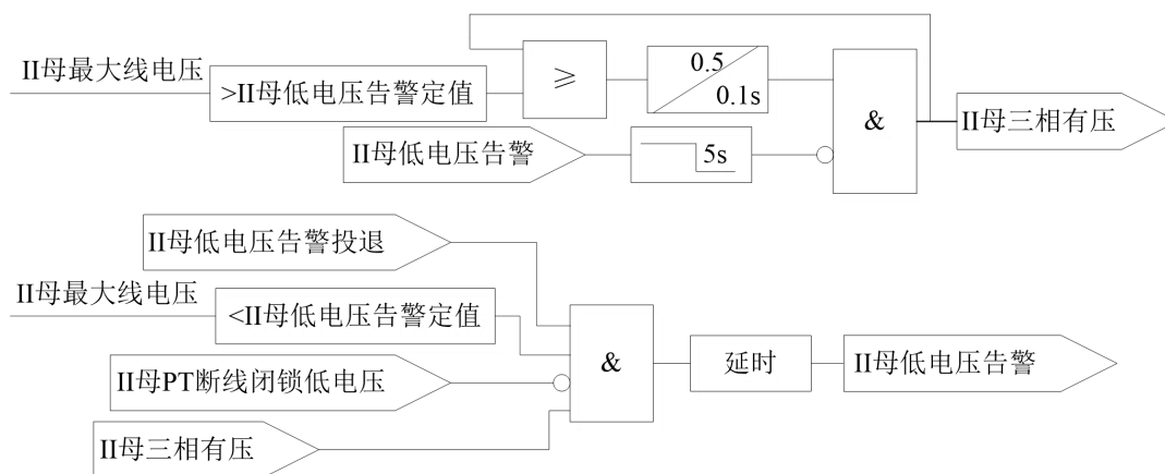
图 9.9 II 母 PT 低电压告警逻辑
