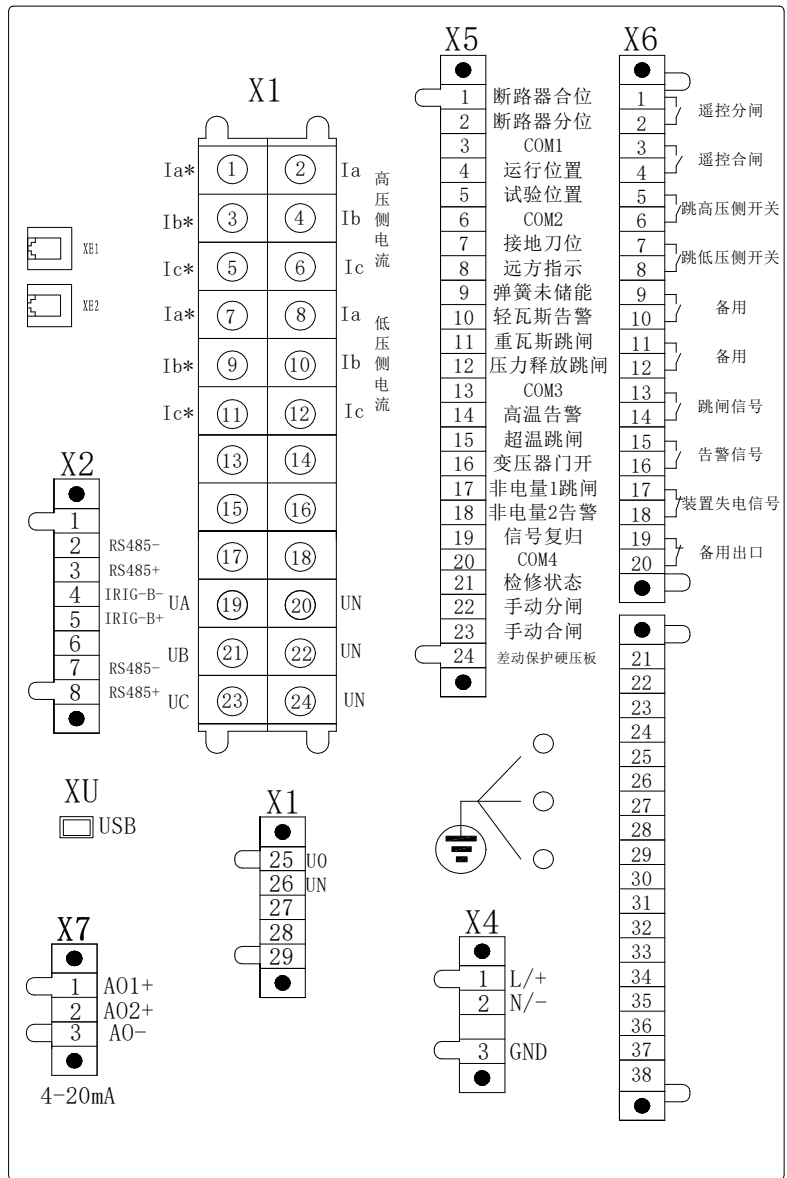
图 7.6 AM5SE-D2 电气接线图
