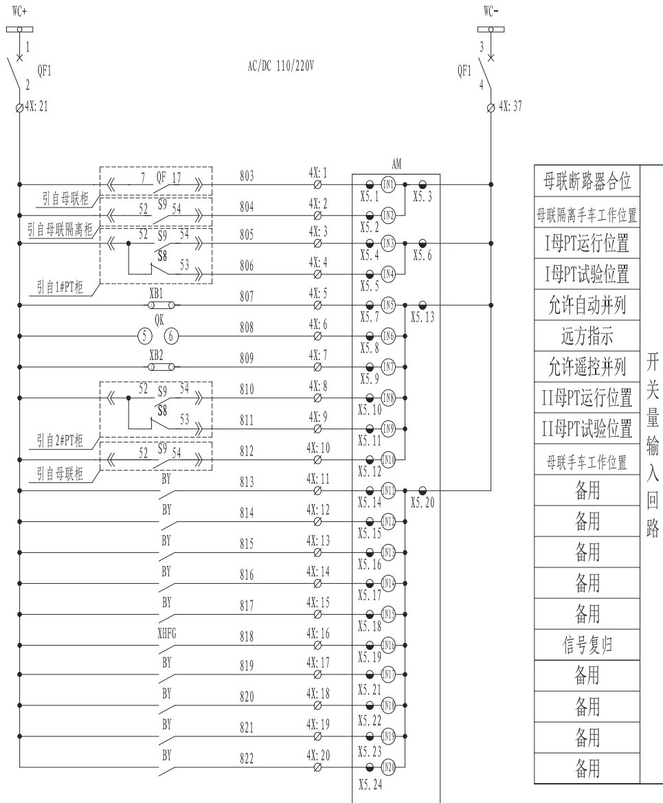
图 9.22 AM5SE-UB 二次原理图 (二)
