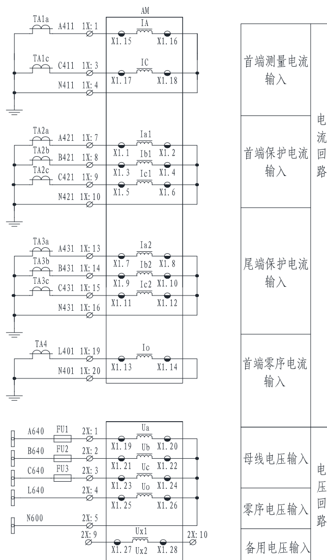
图 6.30 AM5SE-MD 二次原理图（一）
