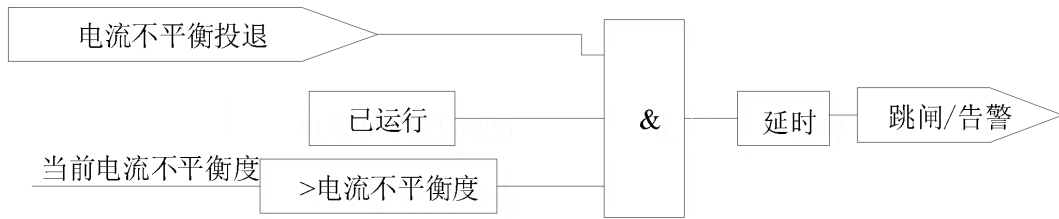
图 3.21 电流不平衡保护逻辑
