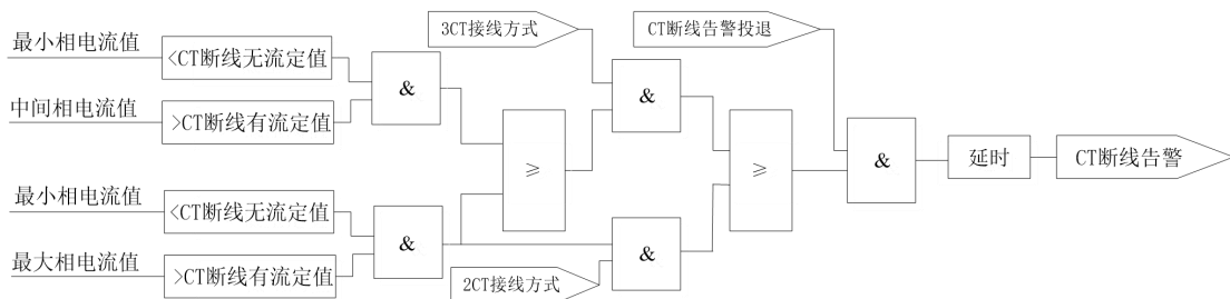
图 5.13 CT 断线告警逻辑
