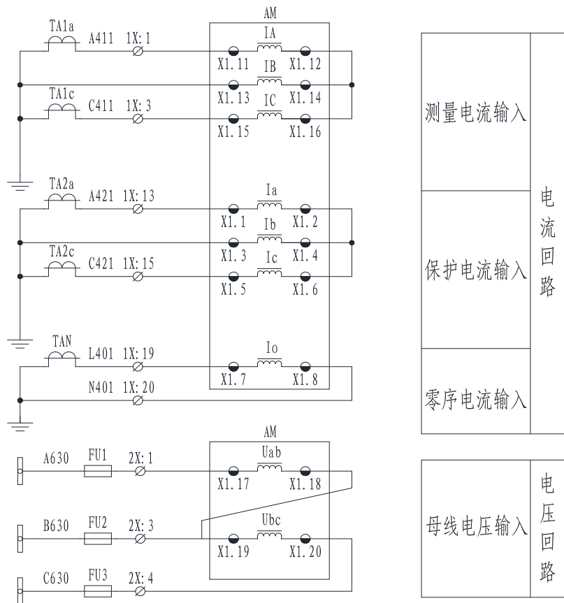
图 3.25 2PT 2CT 接线方法
