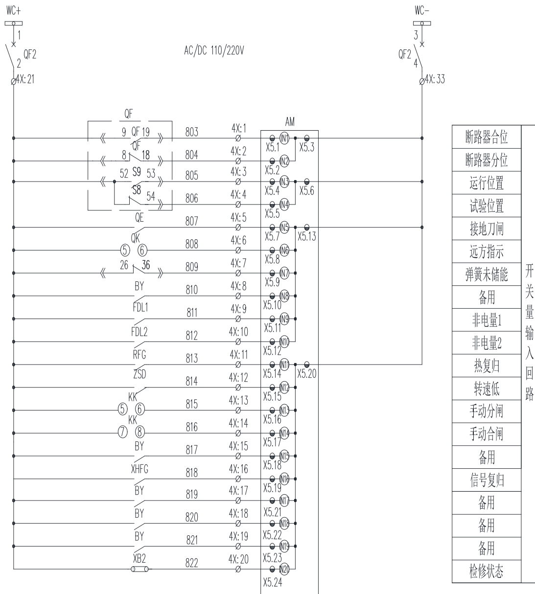
图 3.27 AM5SE-M 二次原理图 (二)
