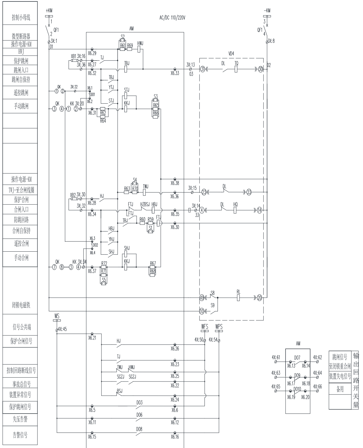
图 14. 10 AM5SE-FE 二次原理图 (三)
