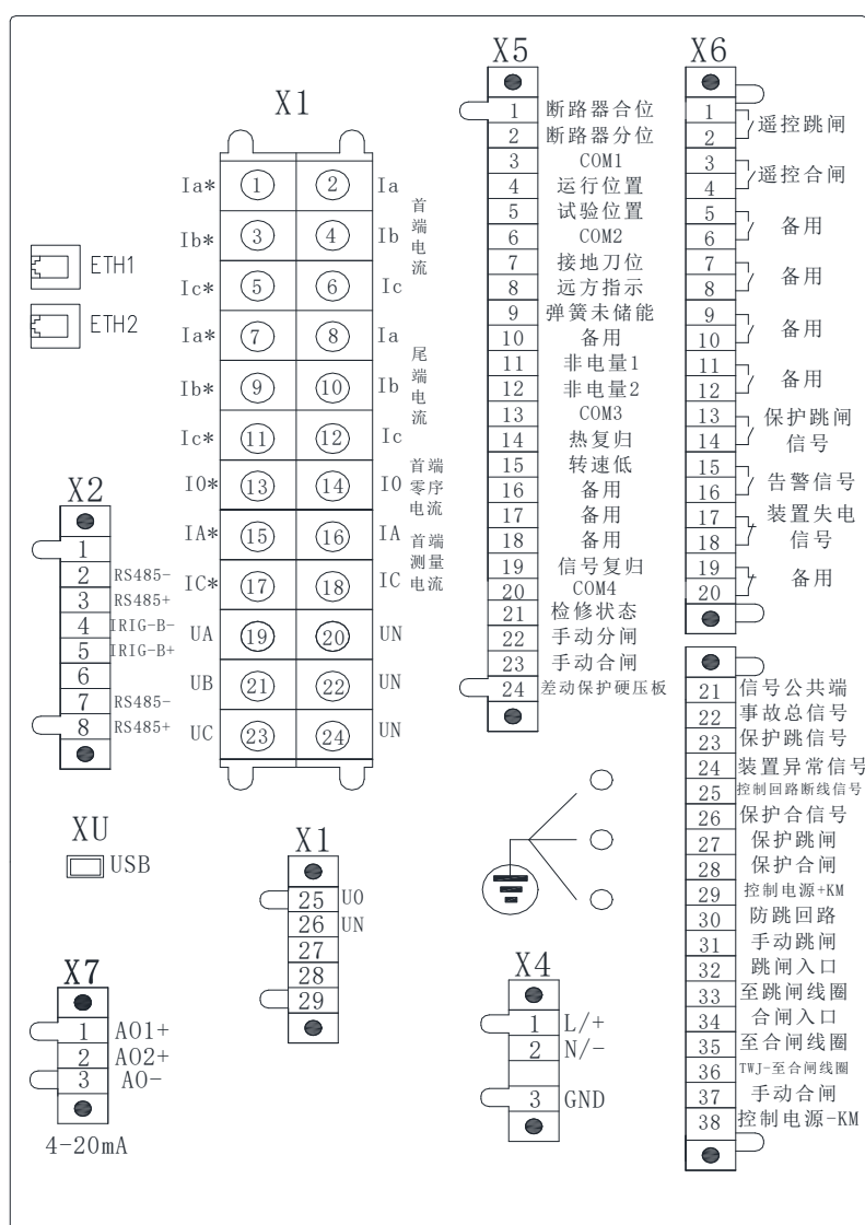
图 6.28 AM5SE-MD 电气接线图
