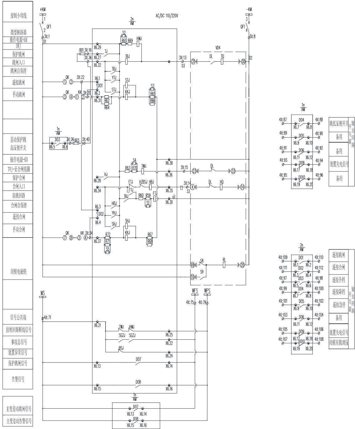
图 8.22 AM5SE-TB 二次原理图 (四)
