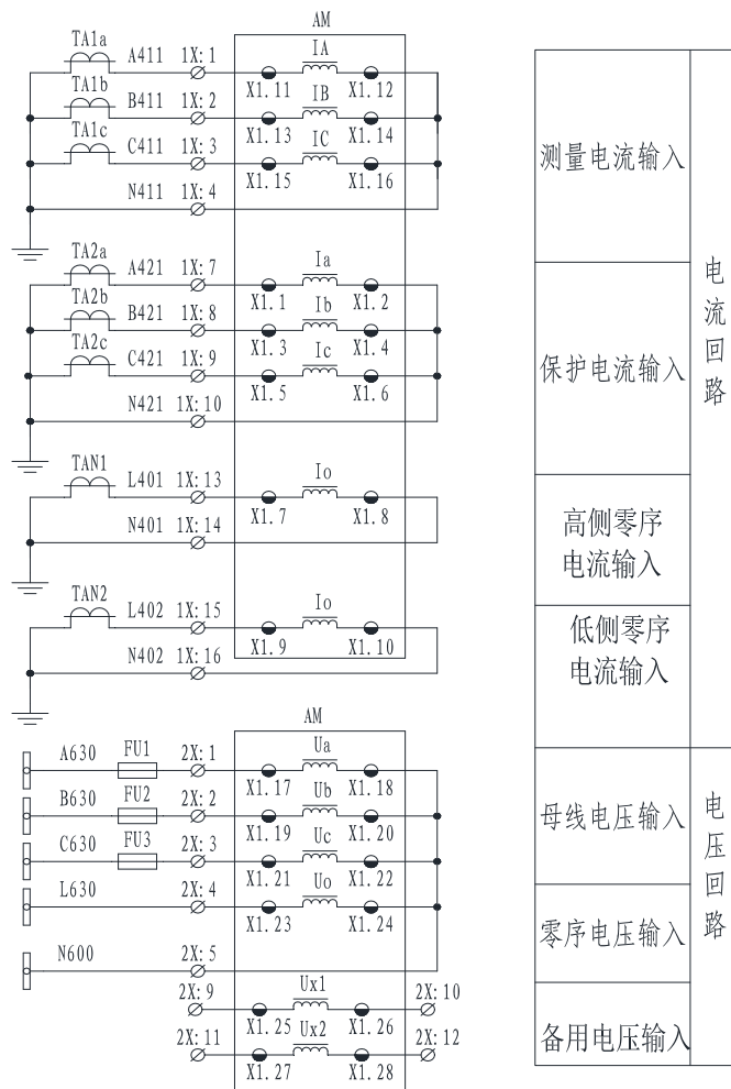
图 2.15 AM5SE-T 二次原理图（一）
