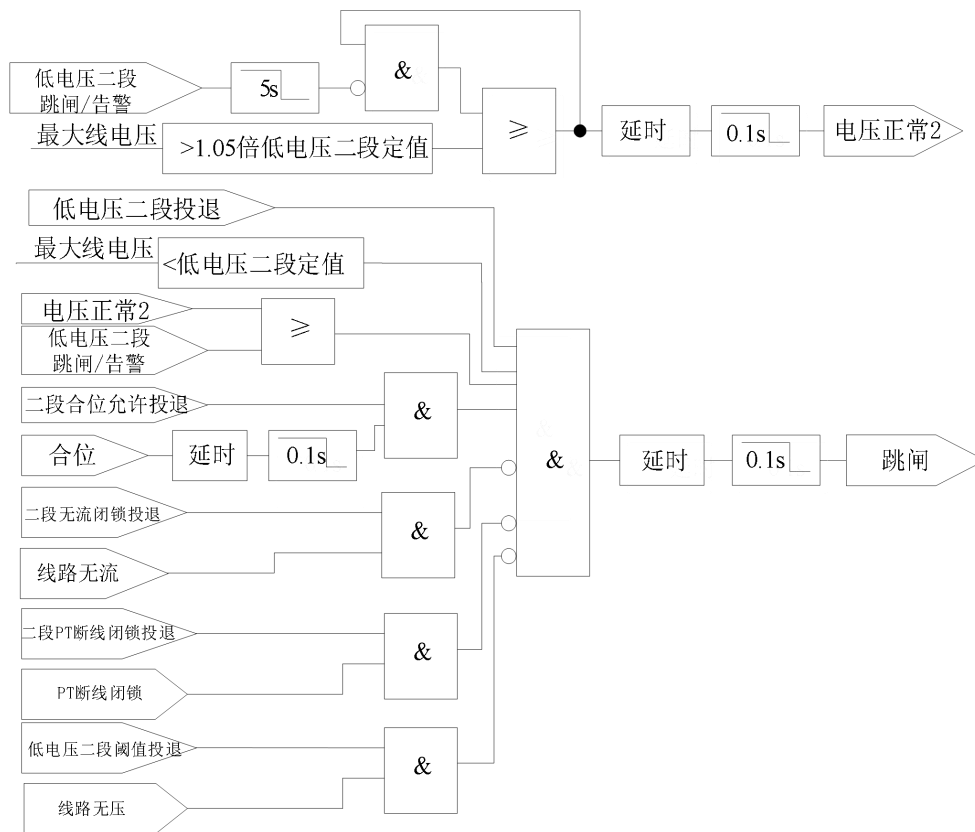
图 15.2 低电压保护逻辑
