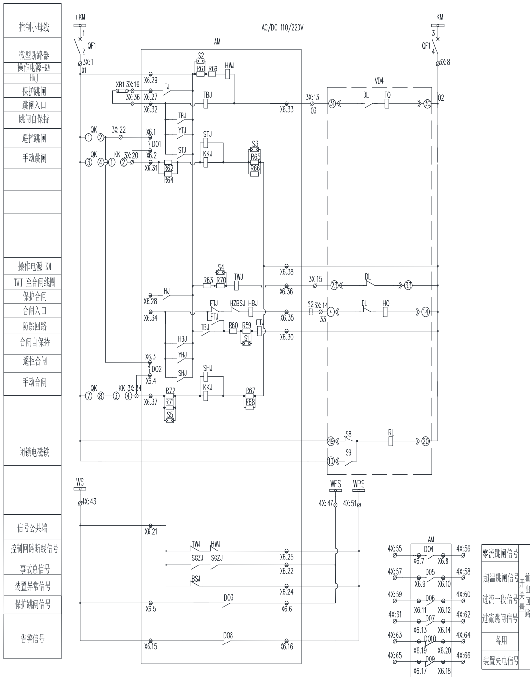
图 2.17 AM5SE-T 二次原理图 (三)
