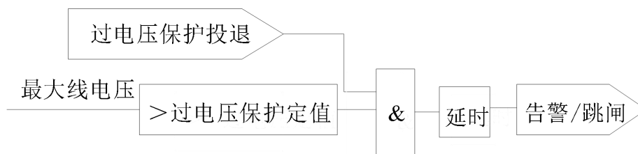
图 6.18 过电压保护逻辑
