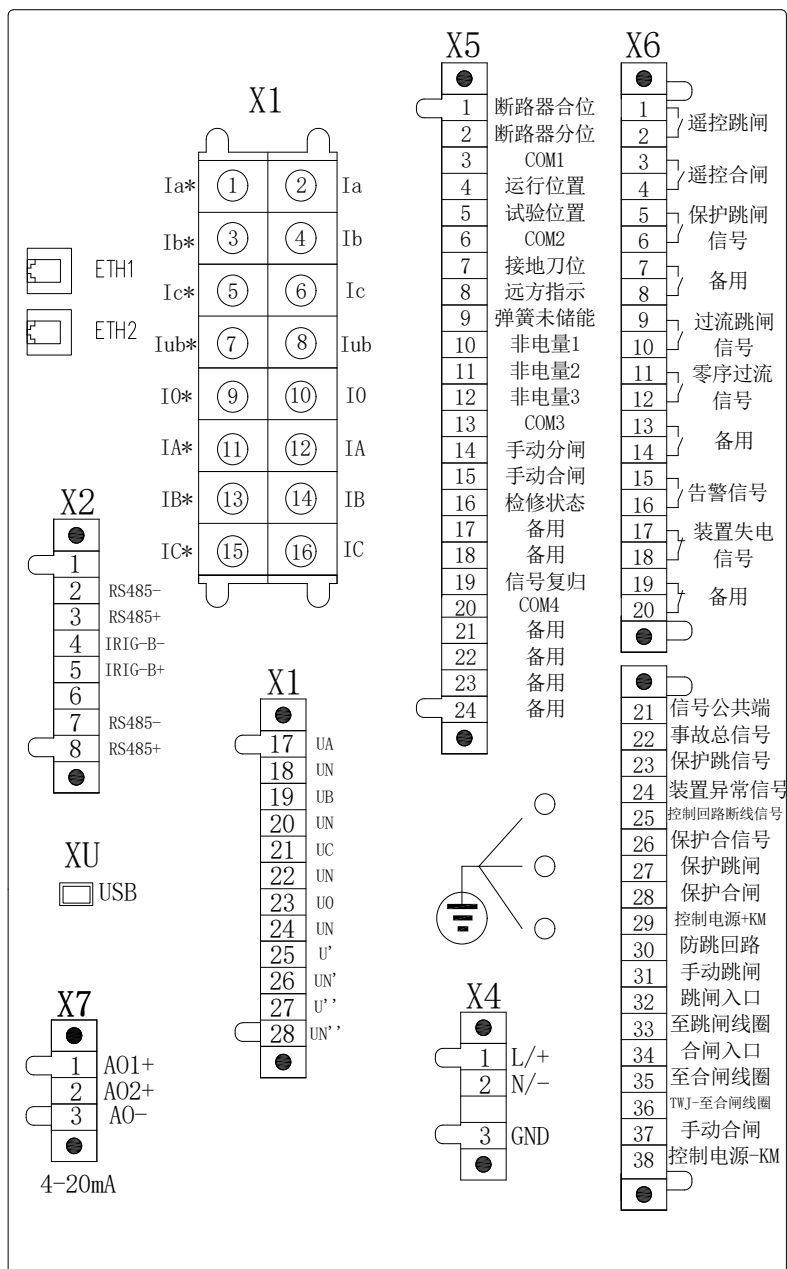
图 5.15 AM5SE-C 电气接线图
