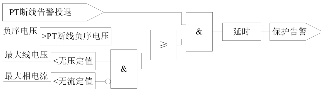
图 6.25 PT 断线告警逻辑
