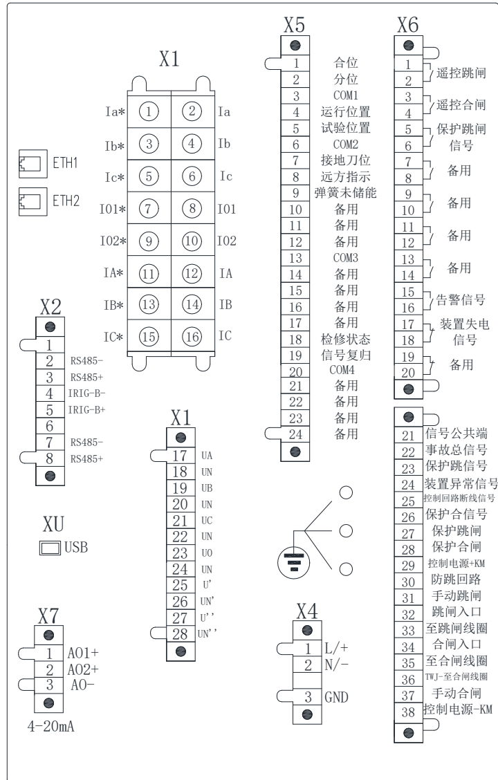
图 15.5 AM5SE-FA 电气接线图
