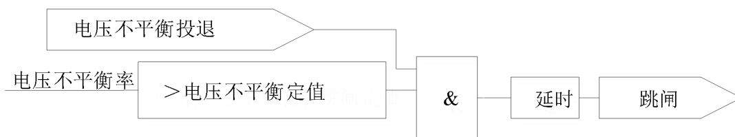
图 6.20 电压不平衡保护逻辑
