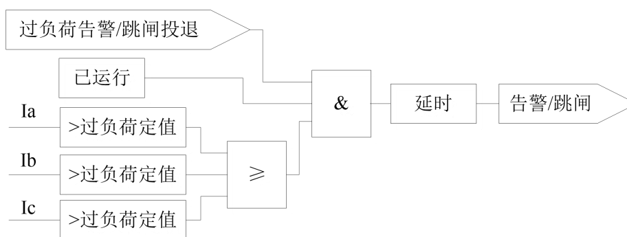
图 3.7 过负荷保护逻辑
