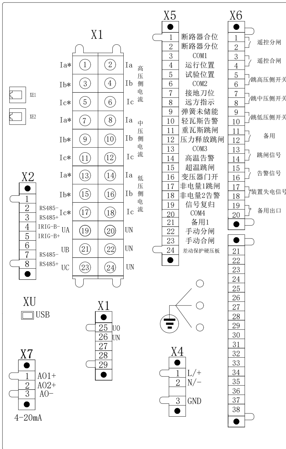
图 10.5 AM5SE-D3 电气接线图
