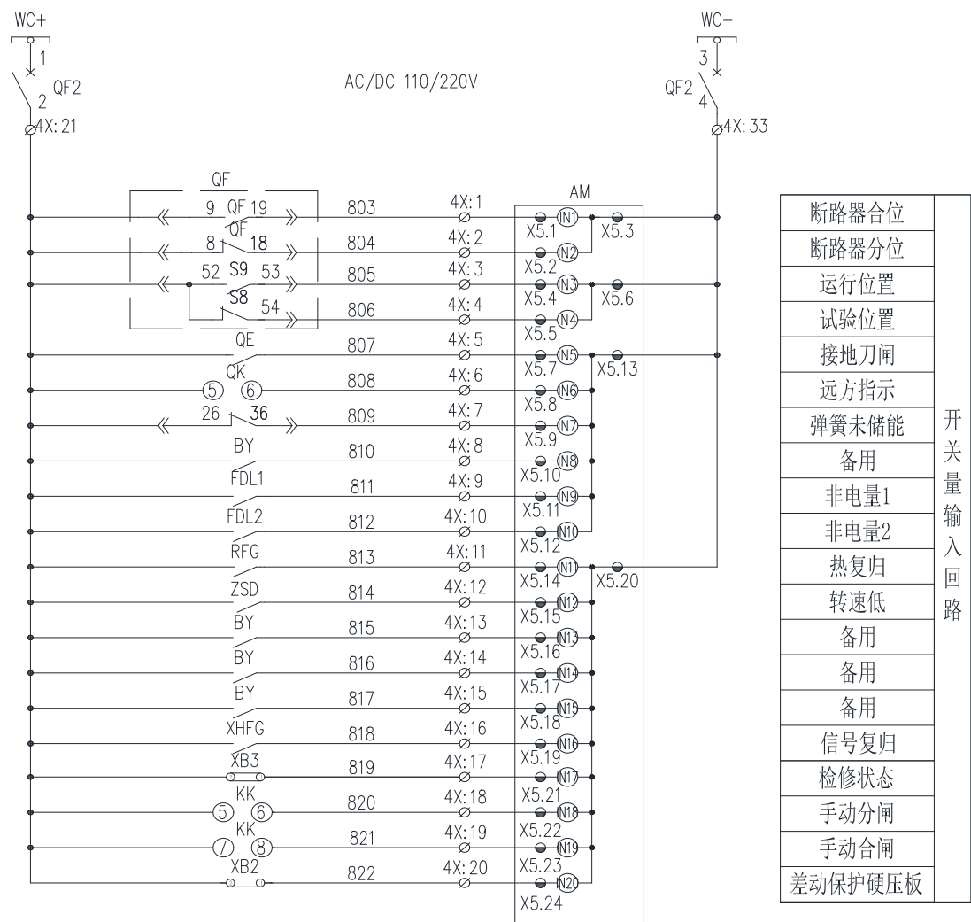
图 6.31 AM5SE-MD 二次原理图 (二)
