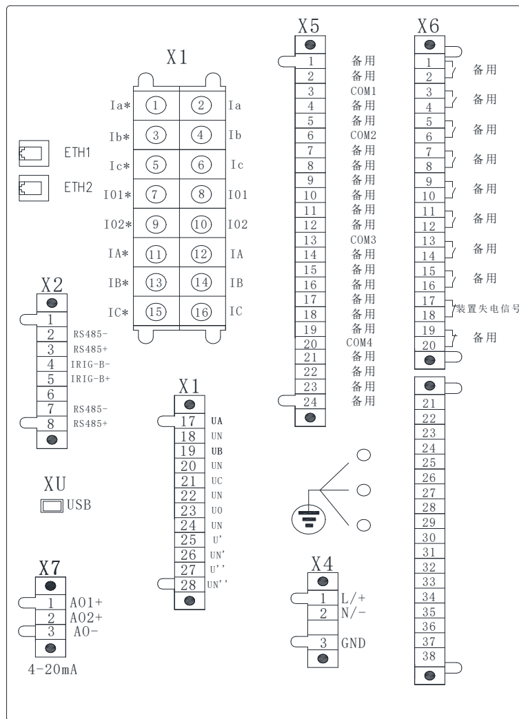
图 13.1 AM5SE-K 电气接线图
