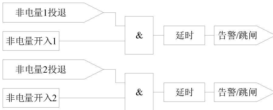
图 6.23 非电量保护逻辑
