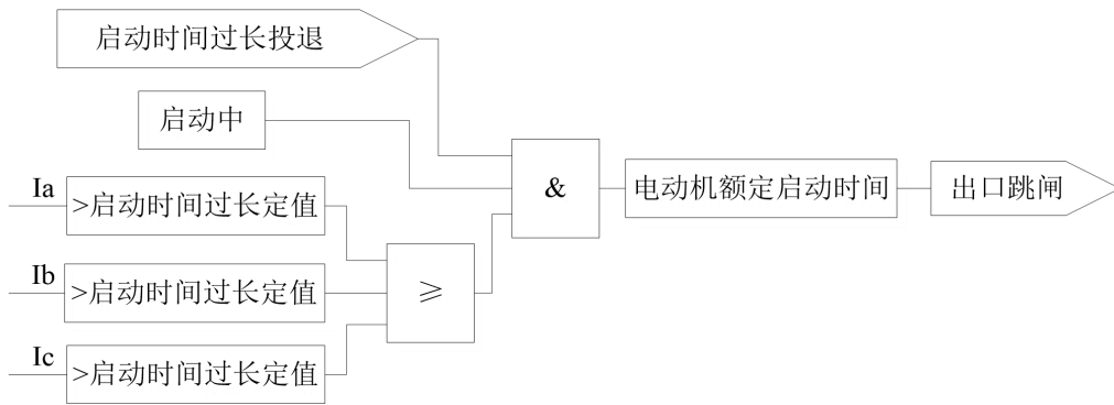
图 3.10 启动时间过长保护逻辑
