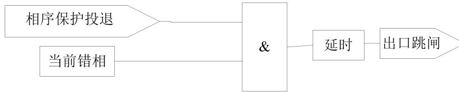
图 3.18 相序保护逻辑
