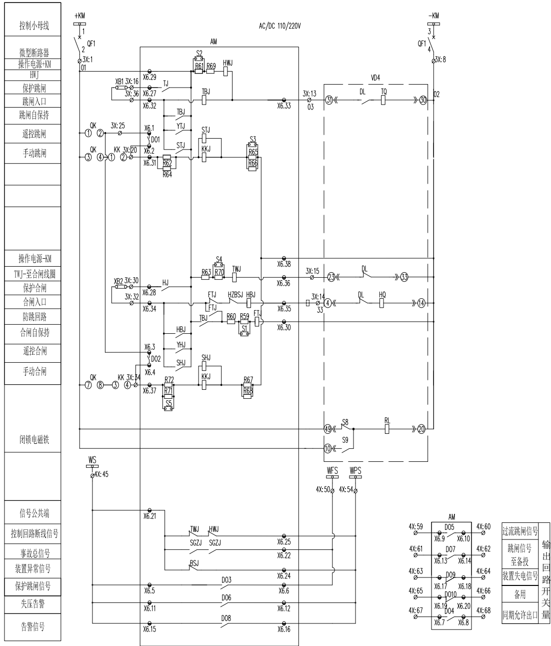
图 1.22 AM5SE-F 二次原理图 (三)
