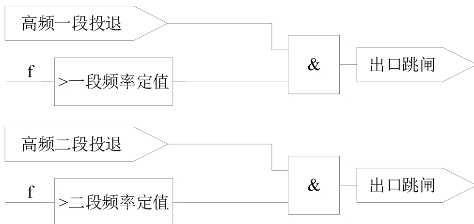
图 11.1 高频保护逻辑
