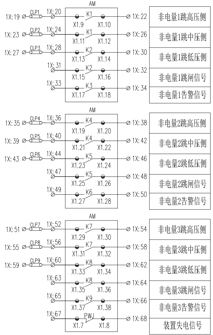
图 12.4 AM5SE-FD 二次原理图 (三)
