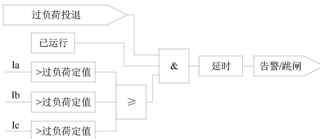
图 6.11 过负荷保护逻辑
