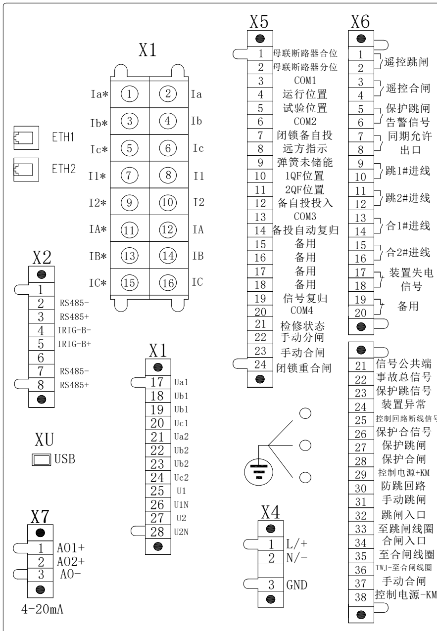
图 4.13 AM5SE-B 电气接线图
