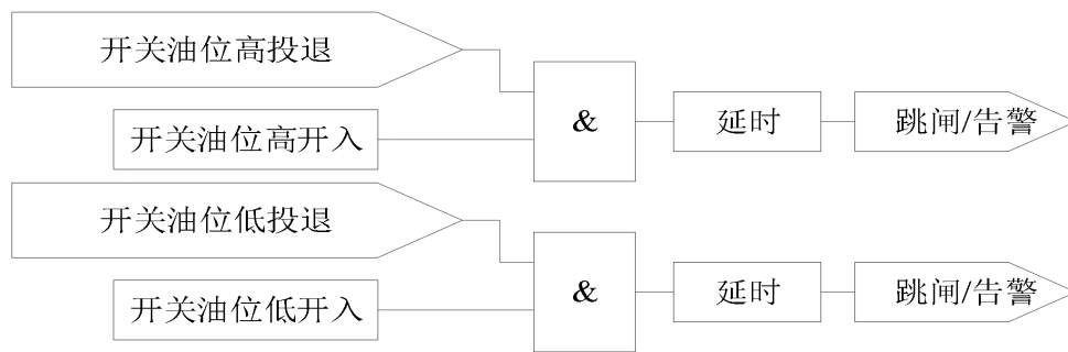
图 8.9 非电量保护逻辑
