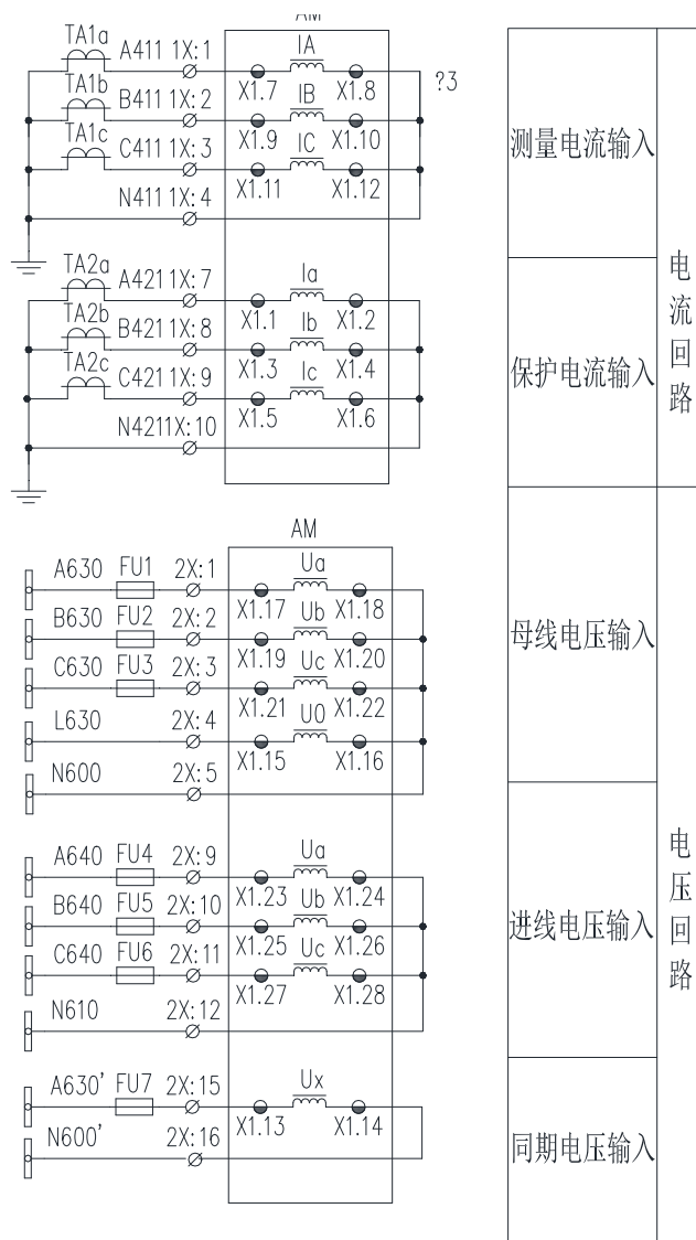
图 11.15 AM5SE-IS 二次原理图（高压）（一）
