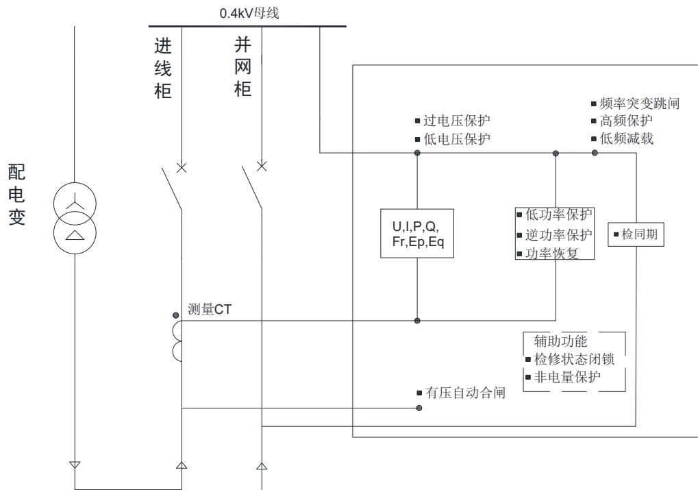
图 11.13 低压并网柜功能接线图
