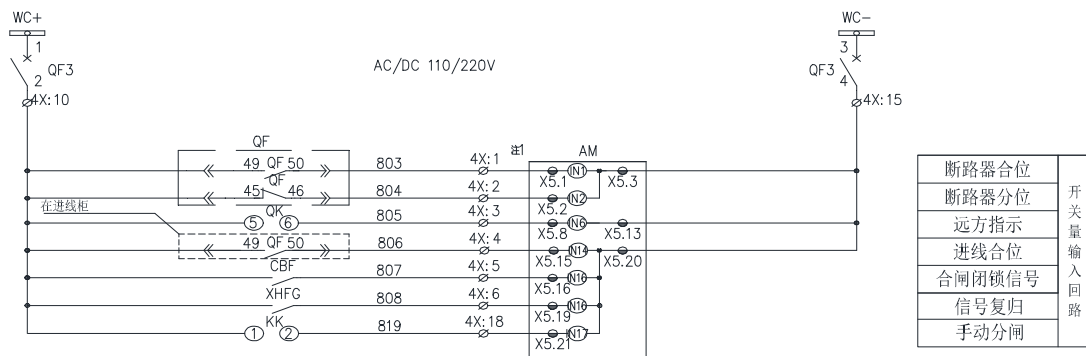
图 11.18 AM5SE-1S 二次原理图（低压）（四）
