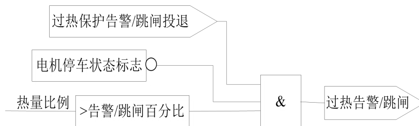
图 6.13 过热保护逻辑
