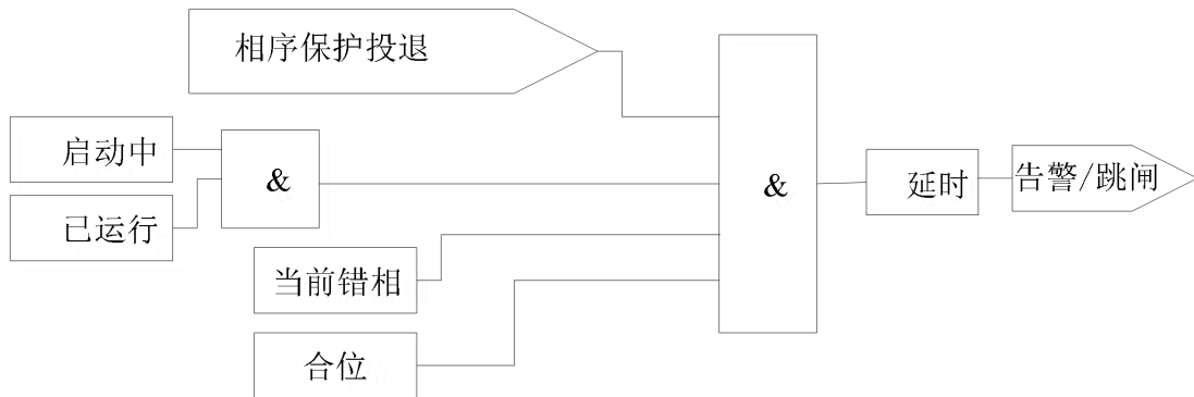
图 6.21 相序保护逻辑
