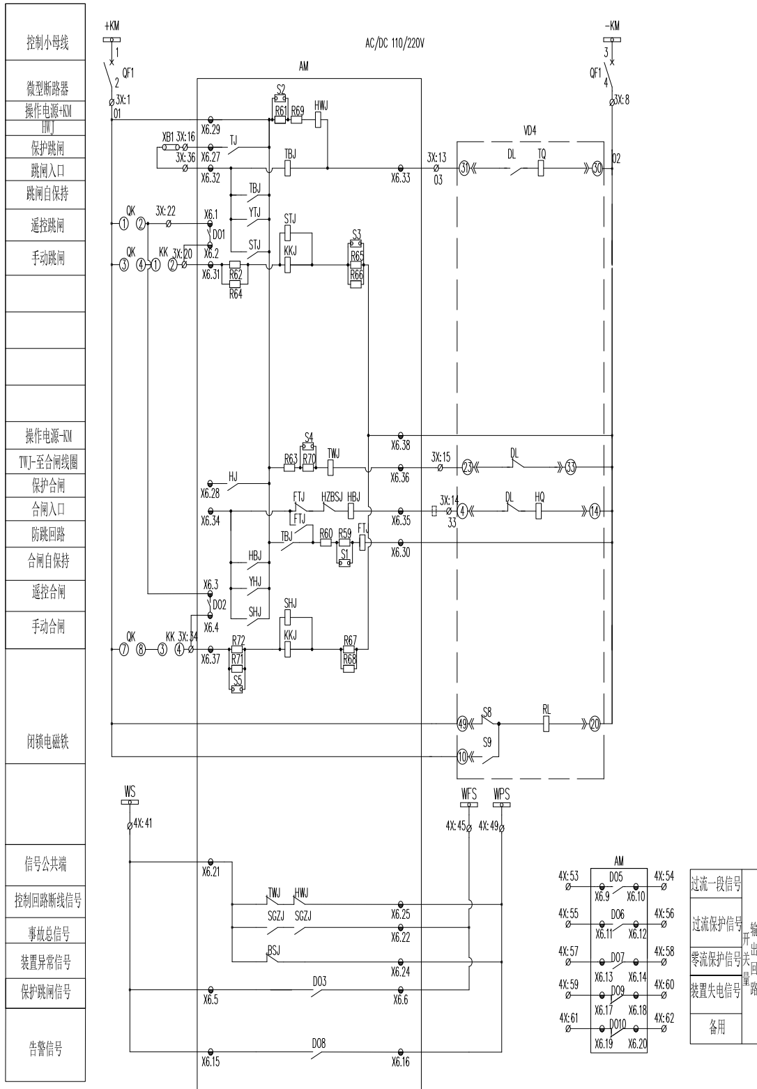
图 3.28 AM5SE-M 二次原理图 (三)
