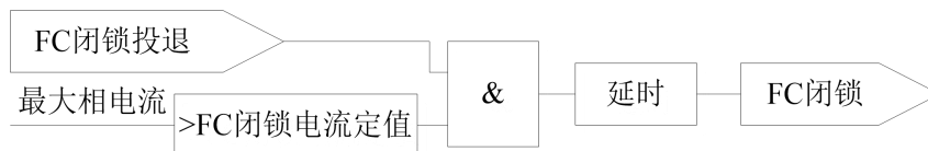
图 6.24 FC 回路配合的过流闭锁功能逻辑
