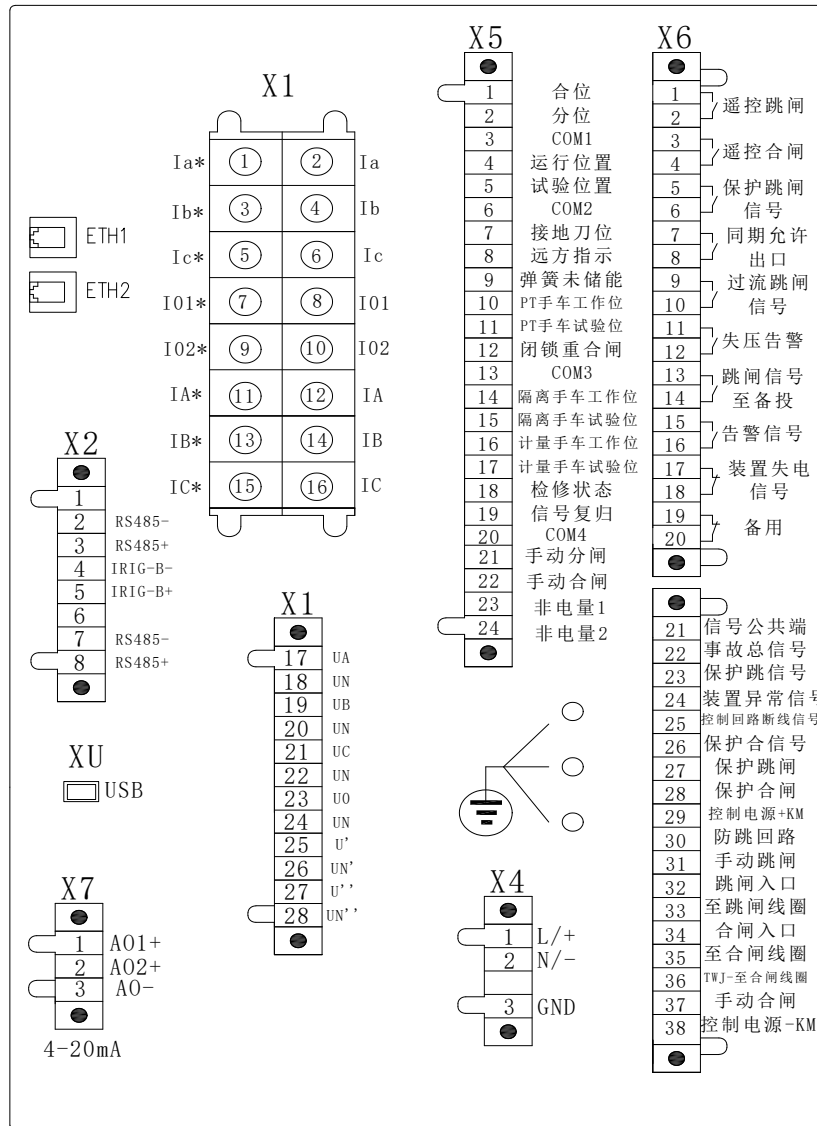
图 1.18 AM5SE-F 电气接线图
