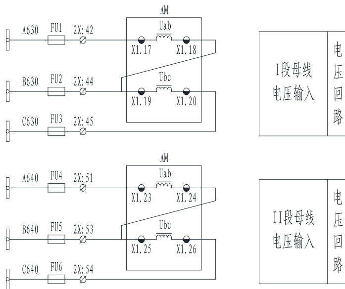
图 9.20 2PT 接线方法
