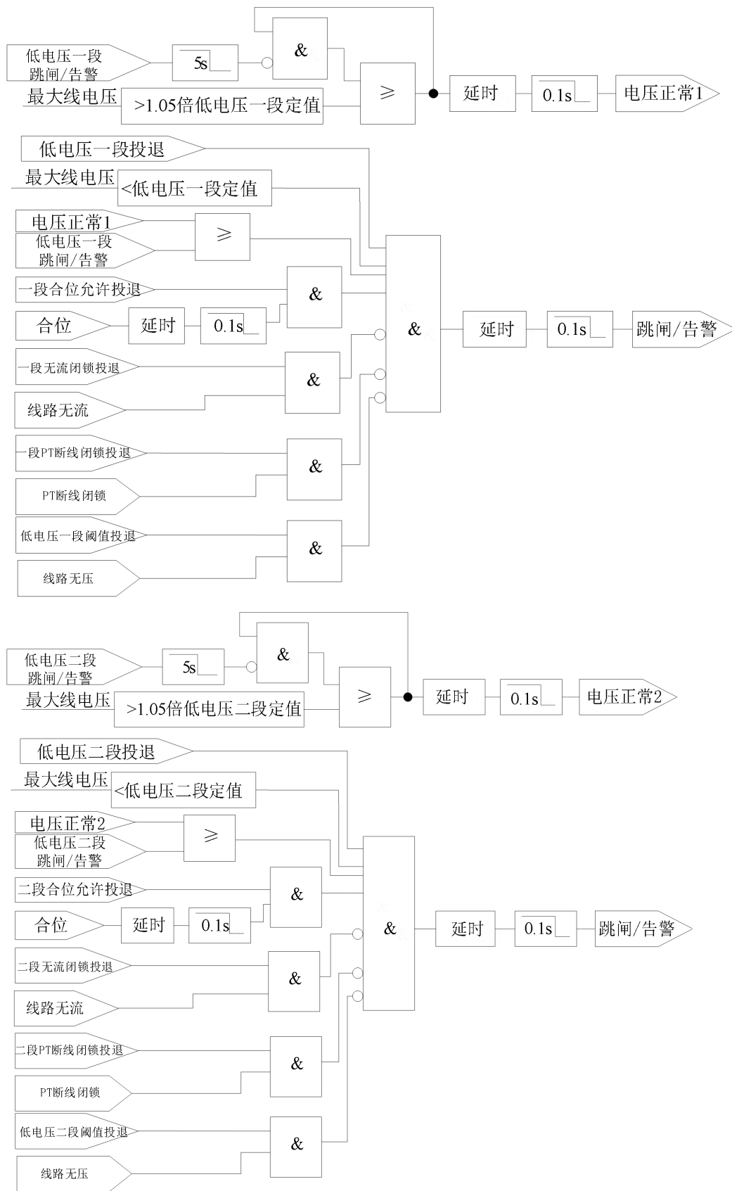
图 14.2 低电压保护逻辑
