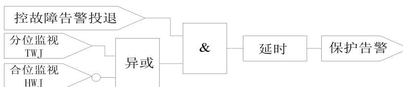
图 1.8 控制回路断线告警逻辑
