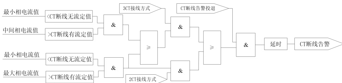
图 3.22 CT 断线告警逻辑
