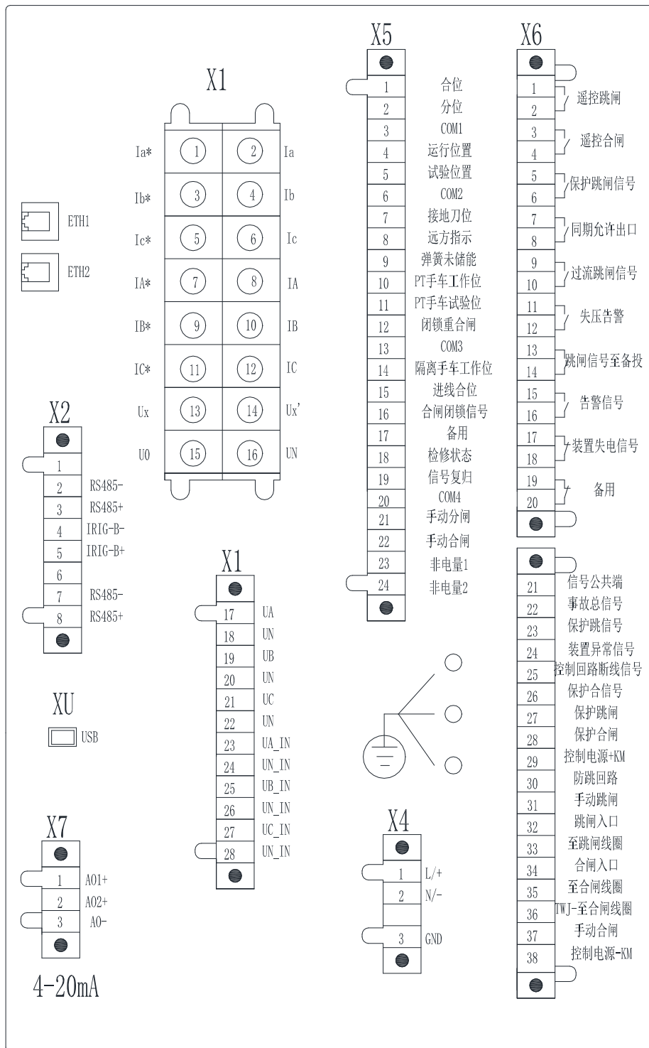
图 11.10 AM5SE-IS 电气接线图
