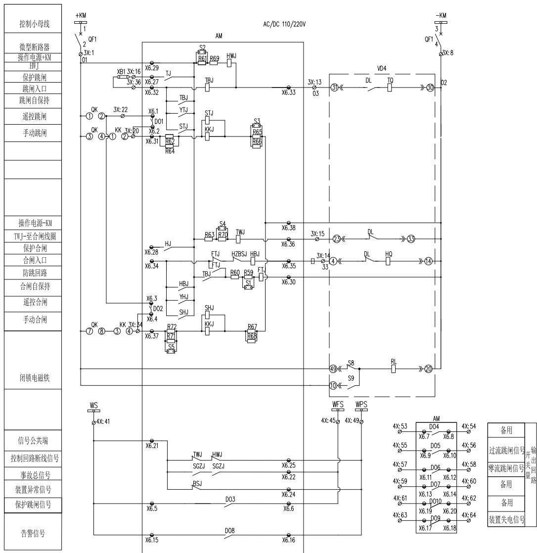
图 5.19 AM5SE-C 二次原理图 (三)
