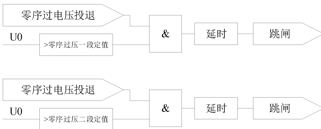
图 15.4 零序过电压保护逻辑
