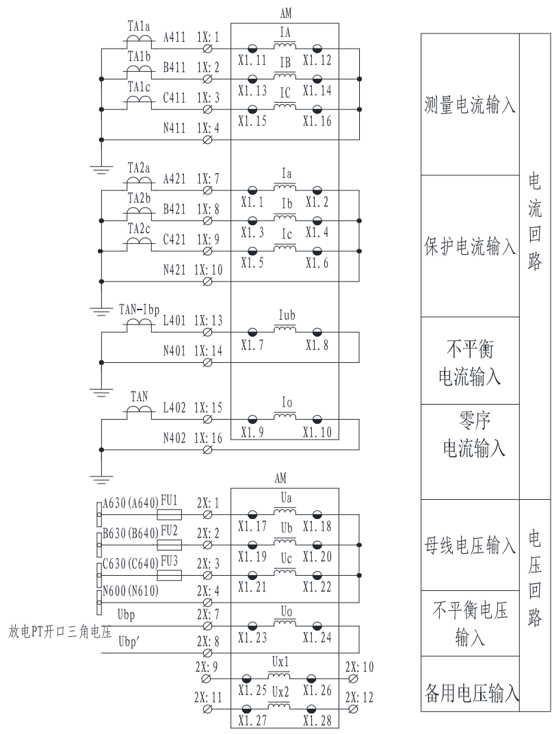
图 5.17 AM5SE-C 二次原理图 (一)
