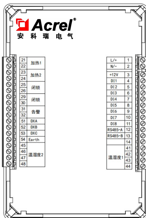
图 1.13 ASD100G 背面端子图
