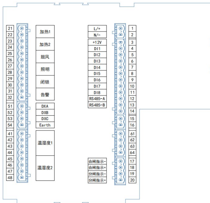
图 1.16 ASD200/310 背面端子图
