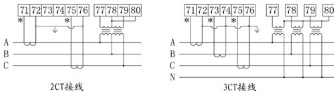
图 2.4 接线方式
