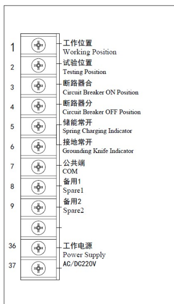
图 1.12 ASD100L 背面端子图
