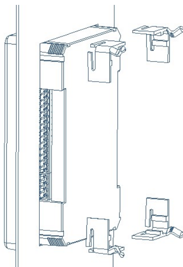
图 1.2 ASD100G 安装方法
