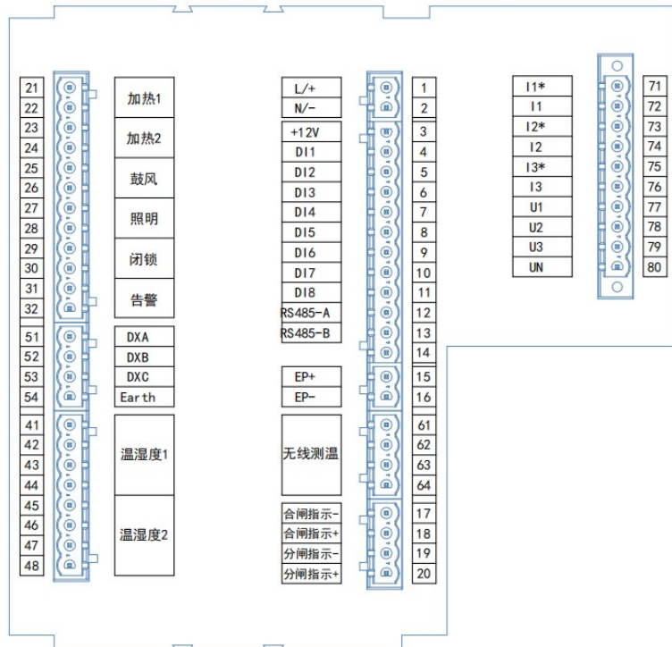
图 1.14 ASD300 背面端子图 Figure 1.14 ASD300 back terminal diagram
