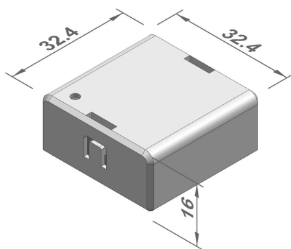
图 1.9 磁吸式无线温度传感器 ATE100M
