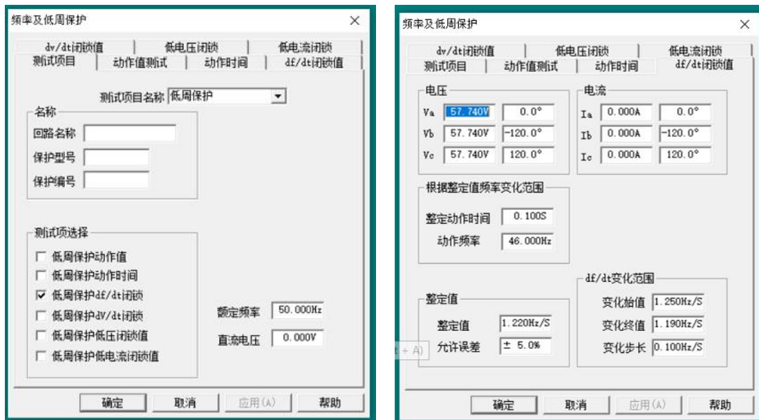
图 2.13 频率突变参数设置
