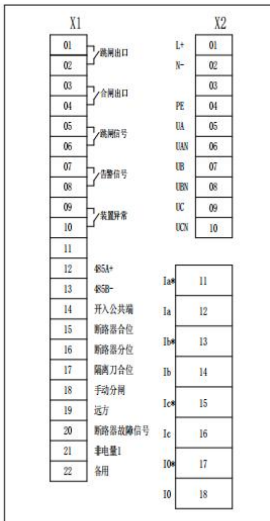
图 2.11 AM2SE-V 电气接线图
