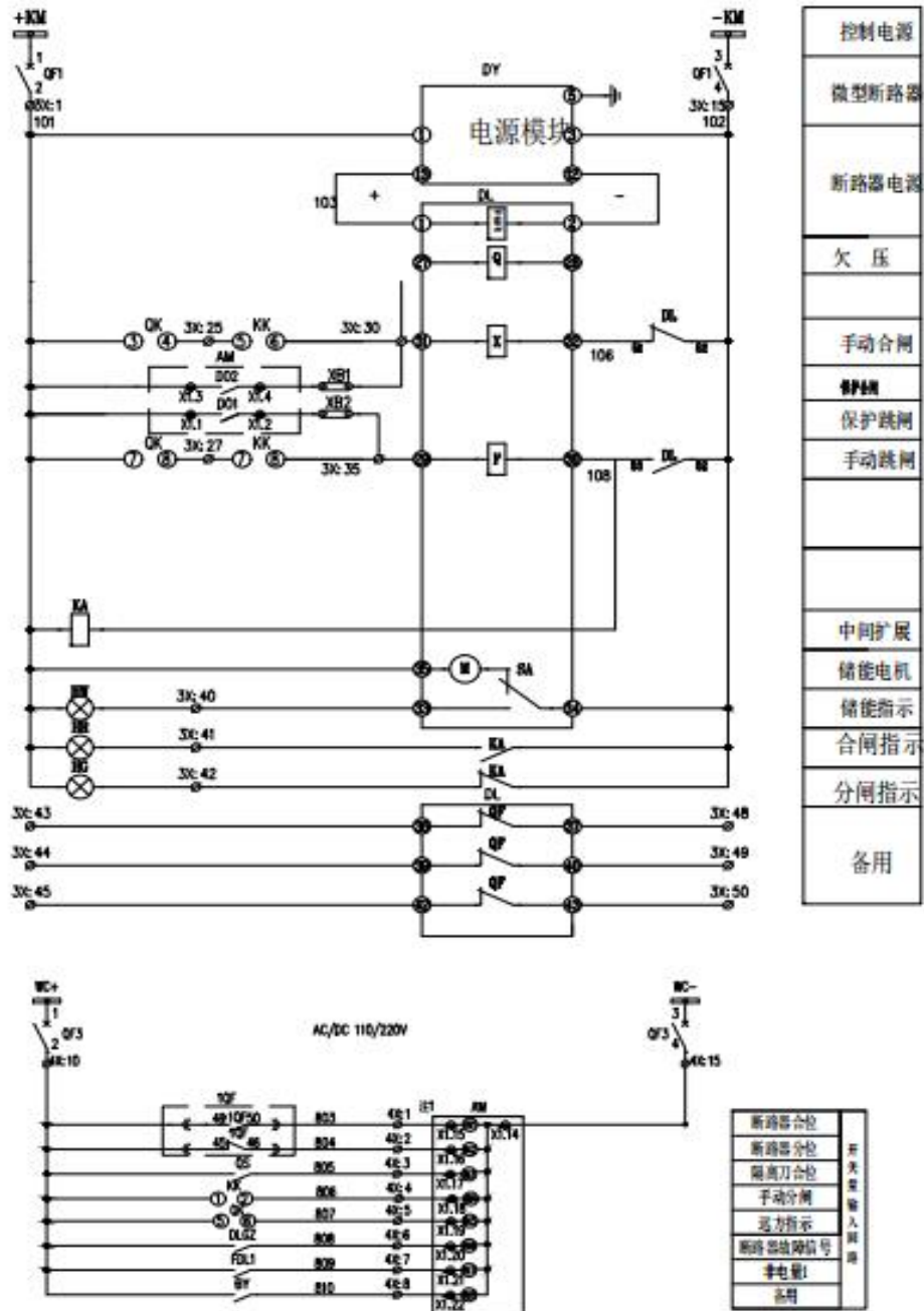
图 2.15 AM2SE-V 二次原理图（二）
