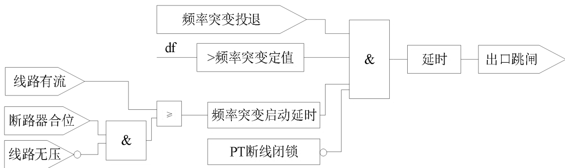
图 2.7 频率突变跳闸逻辑
