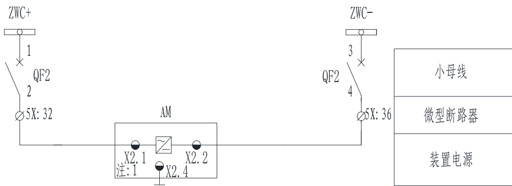
图 2.14 AM2SE-V 二次原理图 (一)
