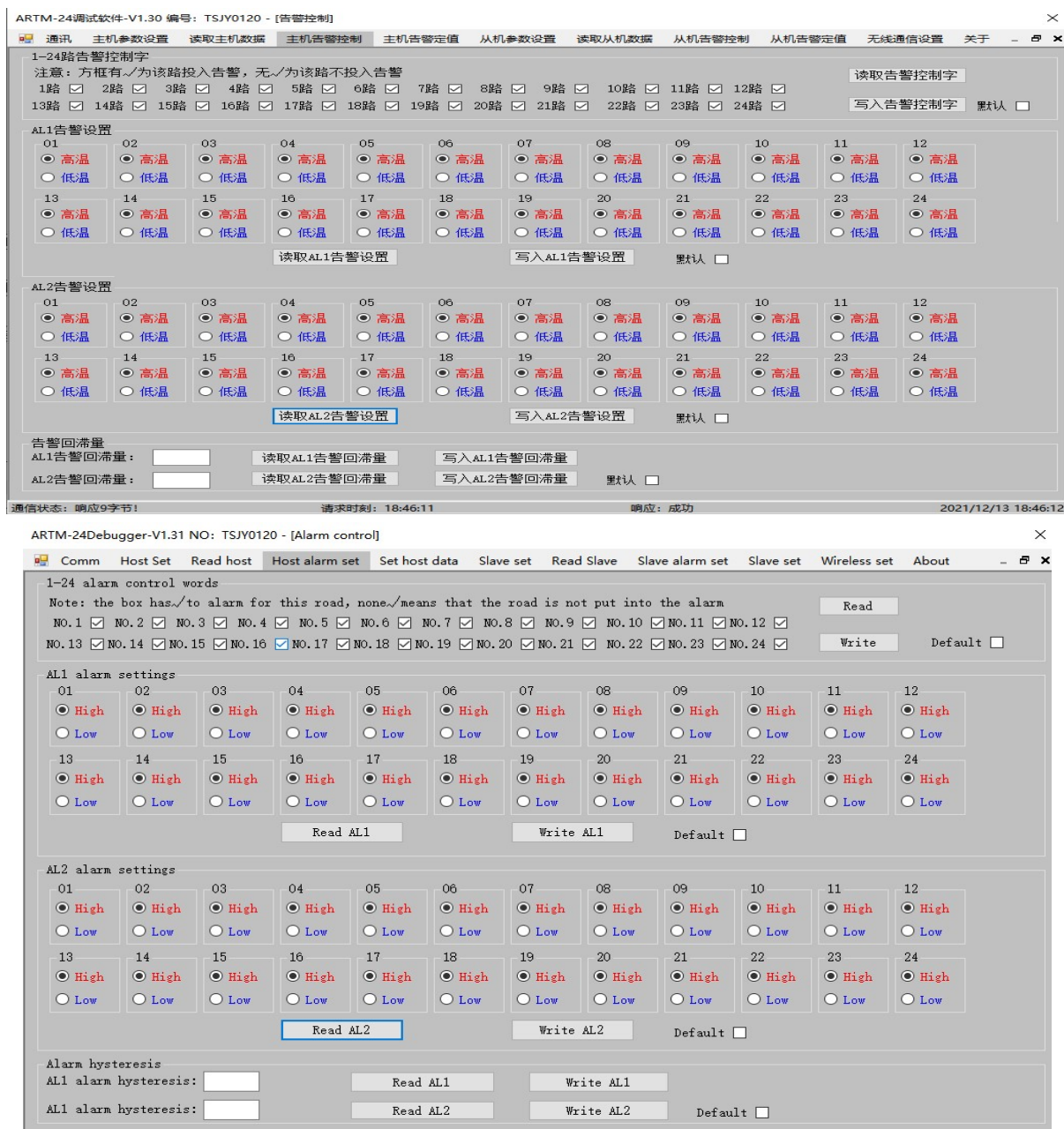
图 1.10 ARTM-24 调试软件主机告警设置界面
