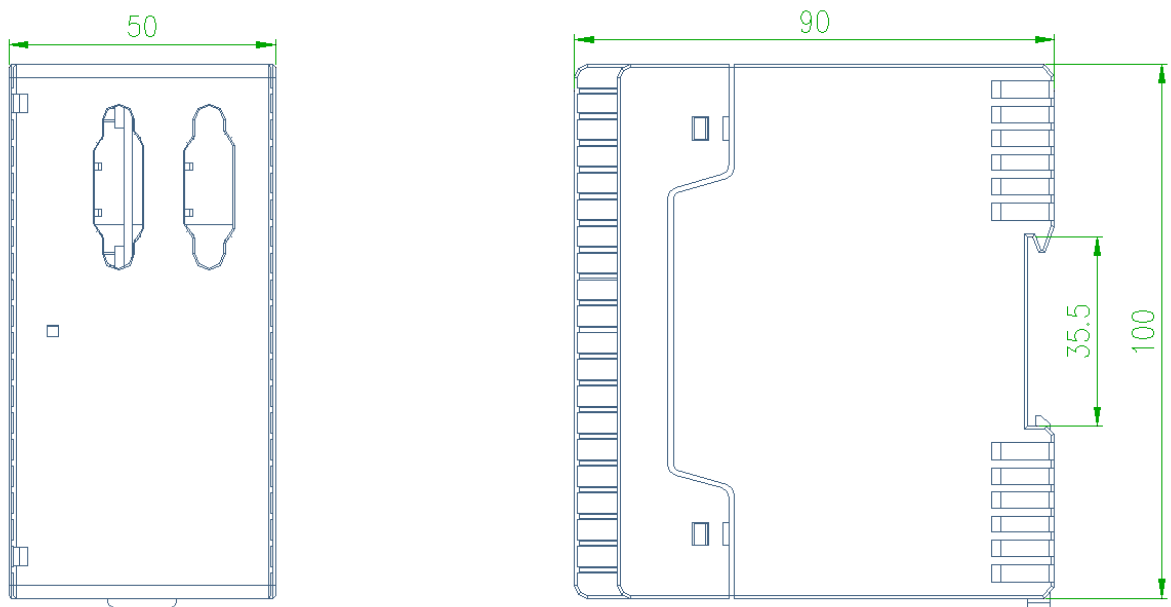
正视图
