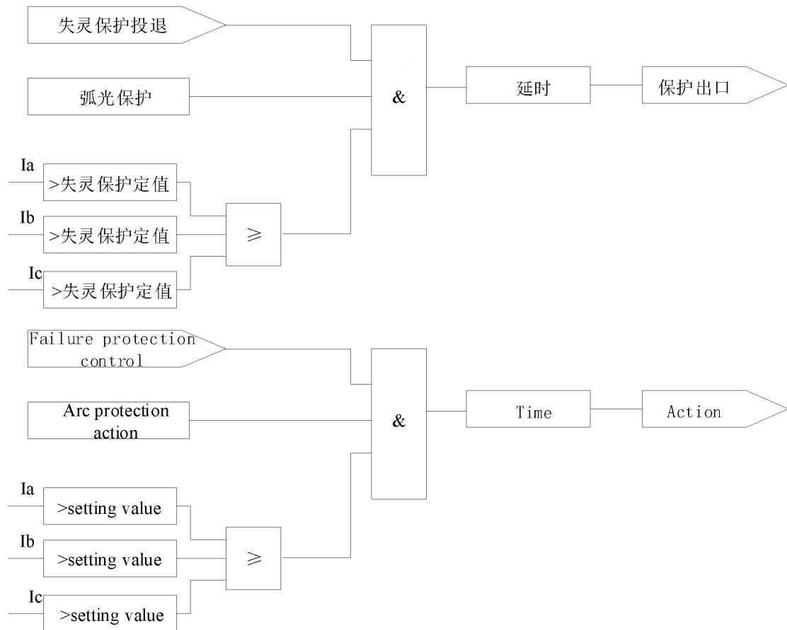
图 1.6 失灵保护逻辑示意图
