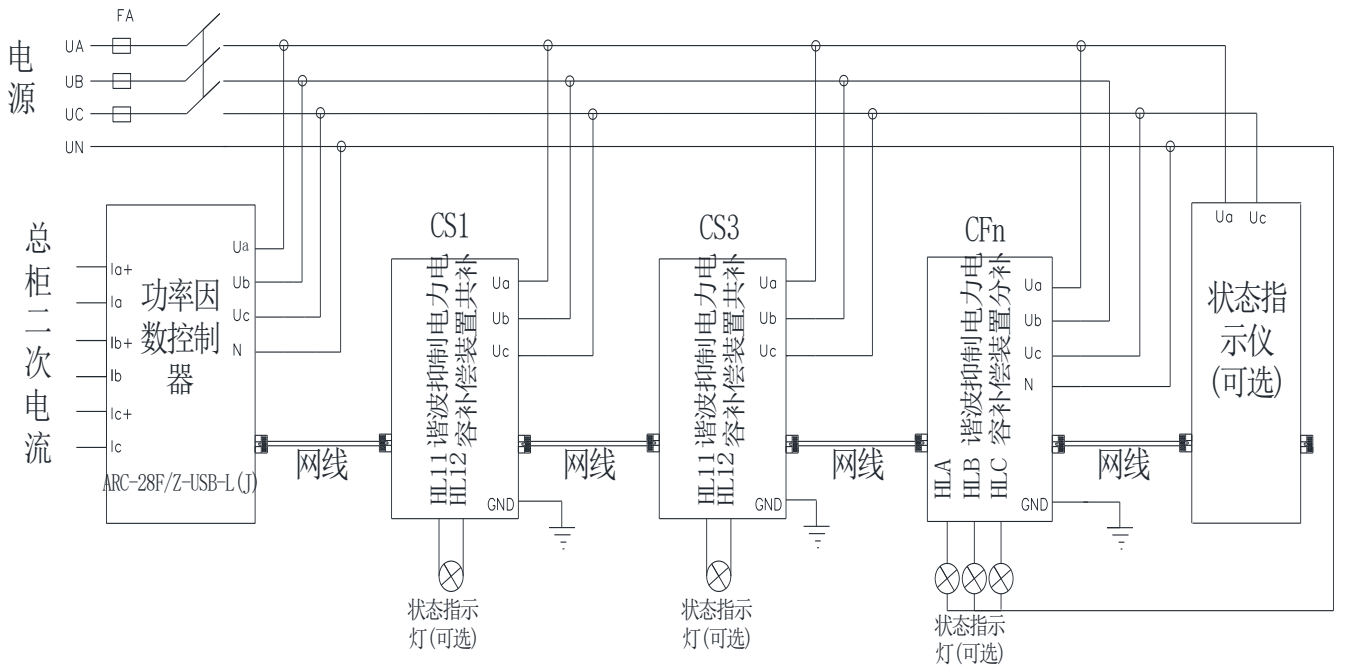
图 119 混补接线图
