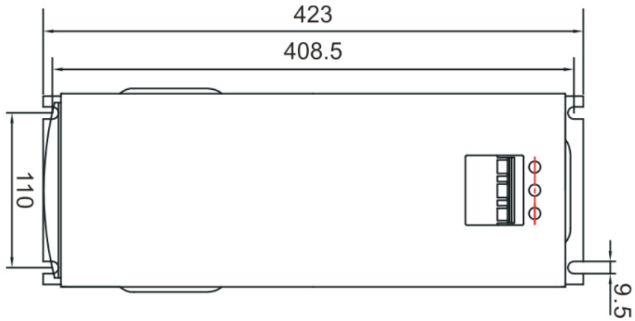
图 115 安装尺寸图
