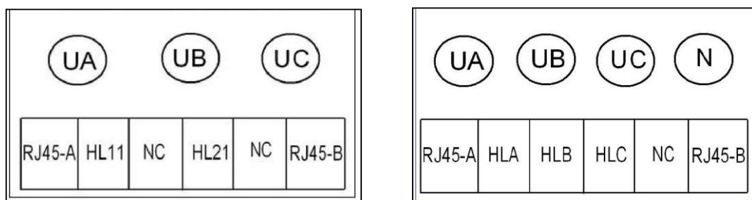
图 78 接线端子图
