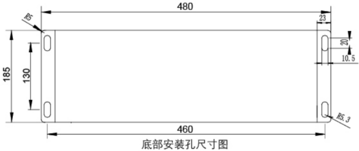
图 76 安装尺寸图
