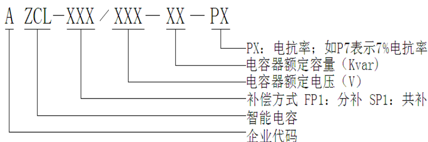
图 56 型号说明
