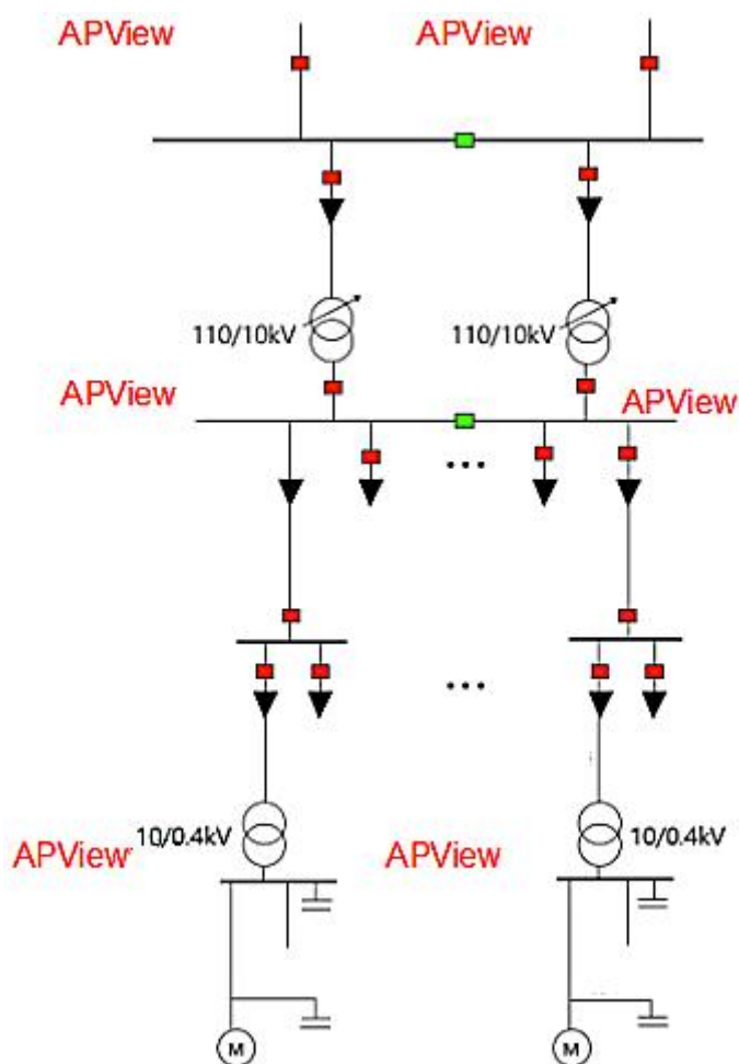
图 4.24 110kV 供电系统 APView 配置图
