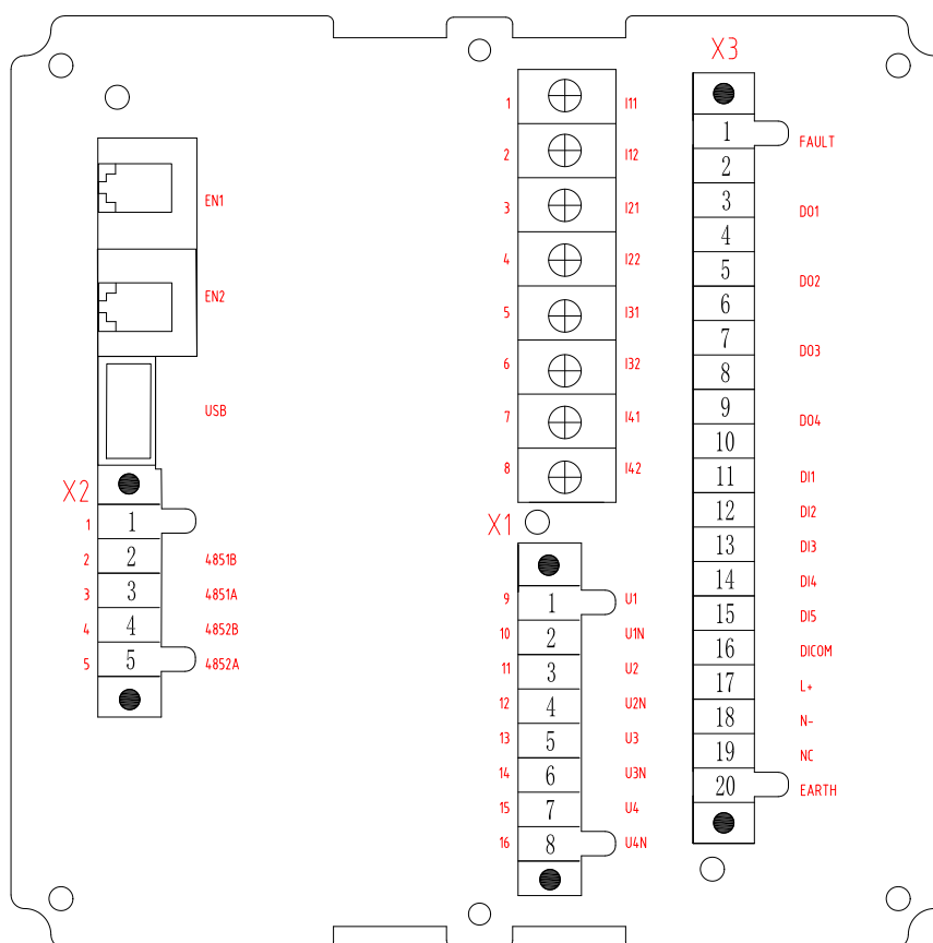
图 3.3 背部端子图
