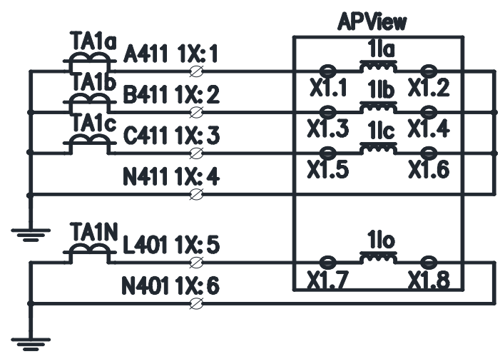
图 3.5 3CT 电流接线 Fig. 3.5 3CT Current wiring
