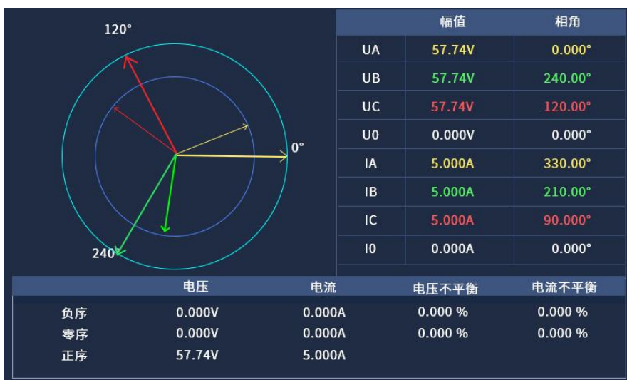
图4.8 矢量图
