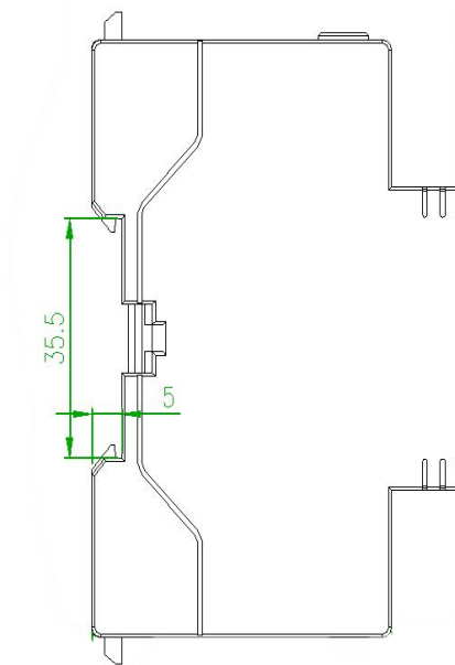
图2 安装方式图
