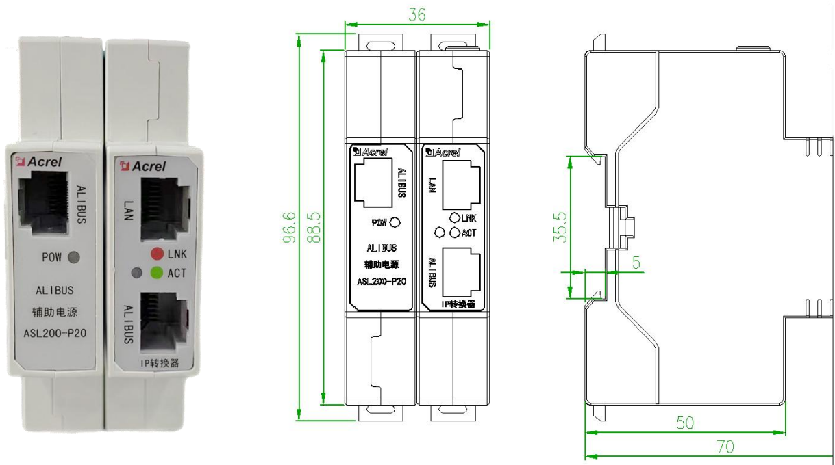
图1 外观及外形尺寸图
