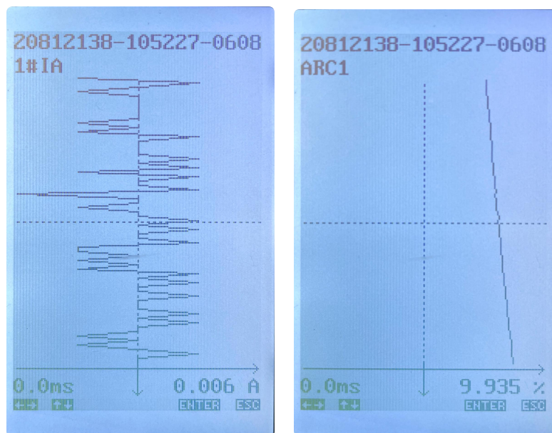
图 4.27 录波数据
