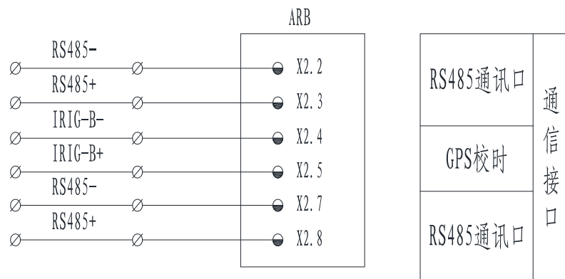
图 3.9 通信接口示意图
