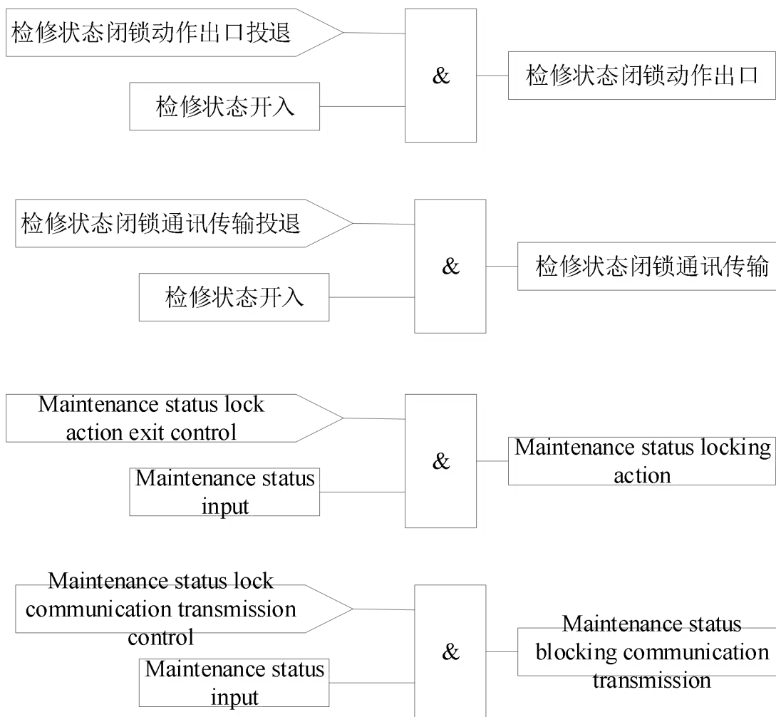
图 1.9 检修状态闭锁逻辑示意图
