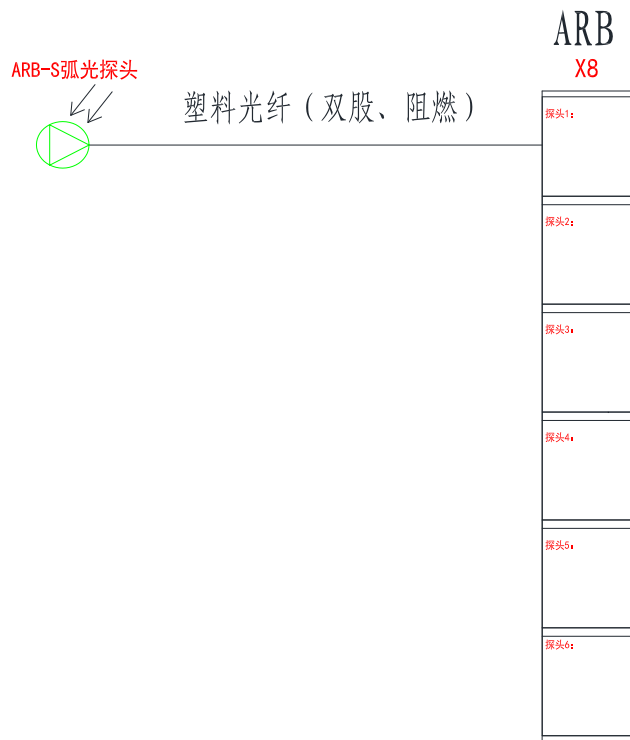
图 3.10 弧光采集接口光纤连接示意图
