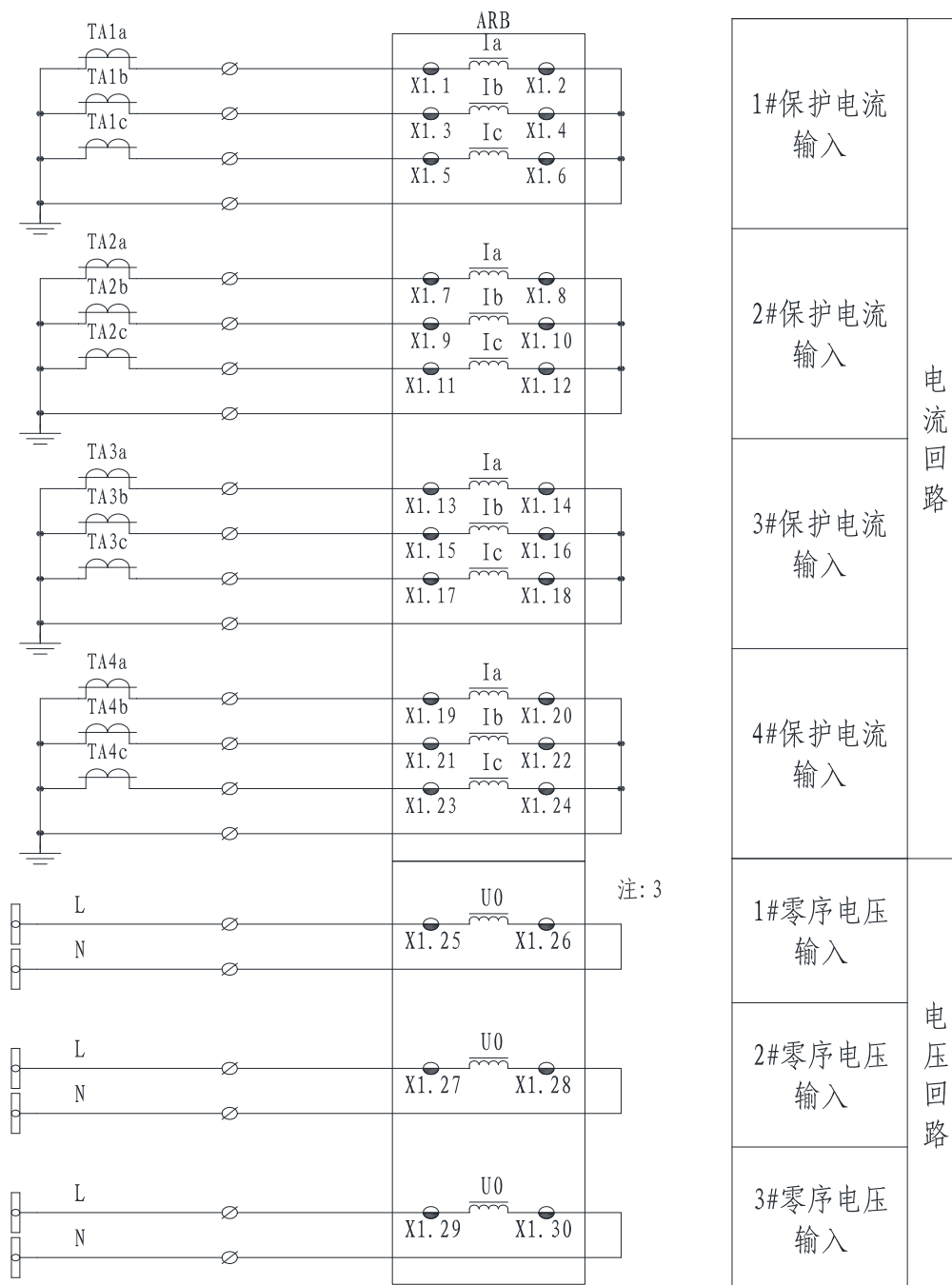
图 3.6 电流、电压回路二次原理图
