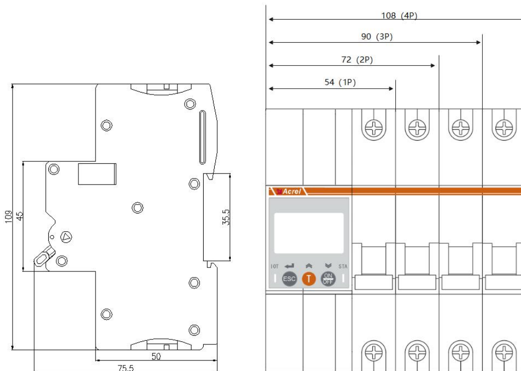
图2 智能微型断路器外形尺寸图（ZL型）
