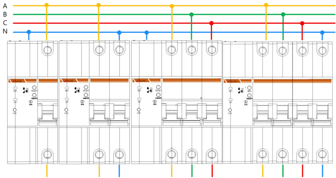
图5 安装接线范例图
