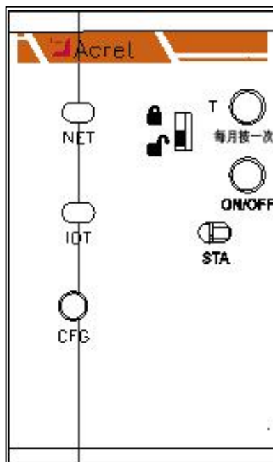
图6 智能微型断路器按键面板说明
