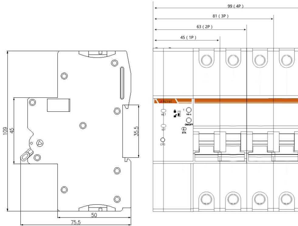
图1 智能微型断路器外形尺寸图（Z型）
