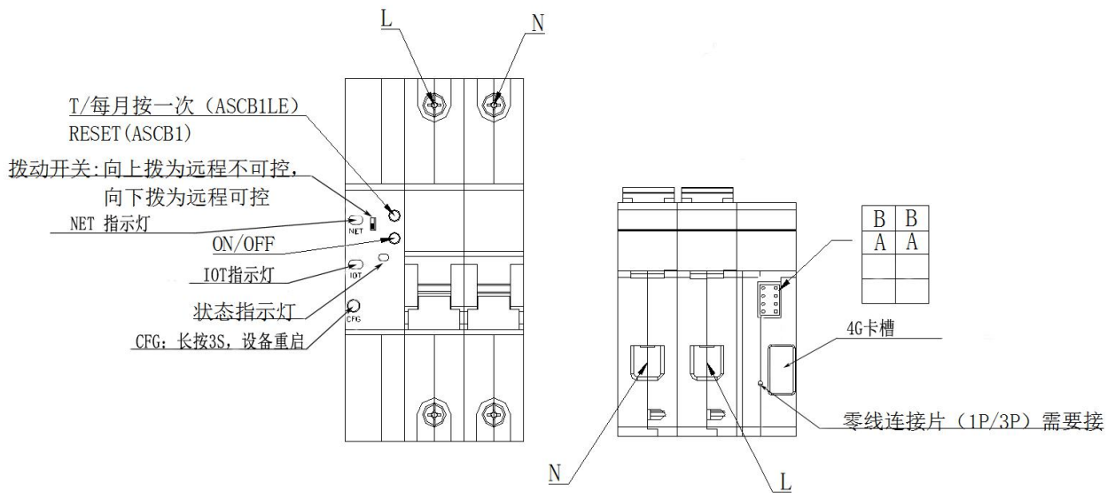
图3 智能微型断路器接线端子示意图 (Z4G型)
