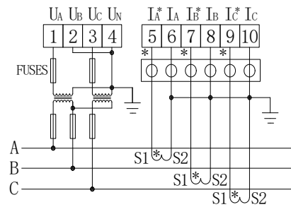
三相三线2PT、3CT
