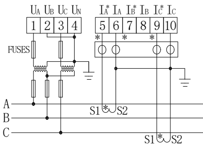
三相三线2PT、2CT
