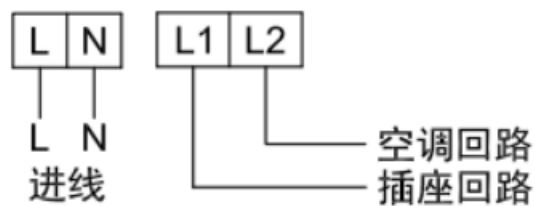
图 4 ADL200-2DM 接线示意图
