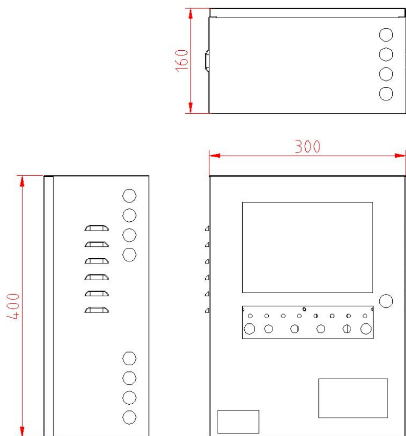
图 1 外形尺寸图
