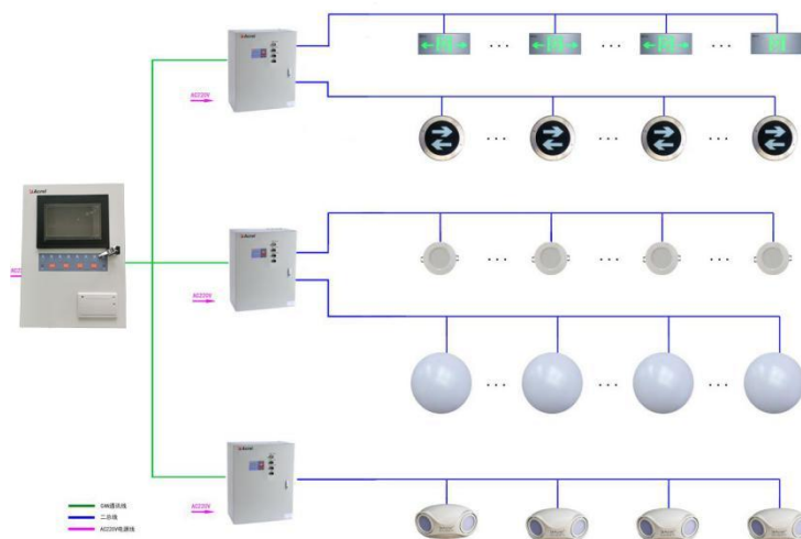
图 3 系统组网示意图
