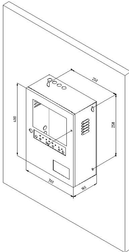
图 2 安装尺寸图
