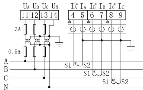
三相四线3PT、3CT
