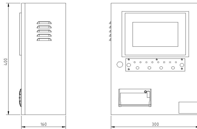
A-C-A100/B3 外观尺寸图
