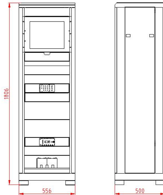
A-C-A100/B3 外观尺寸图
