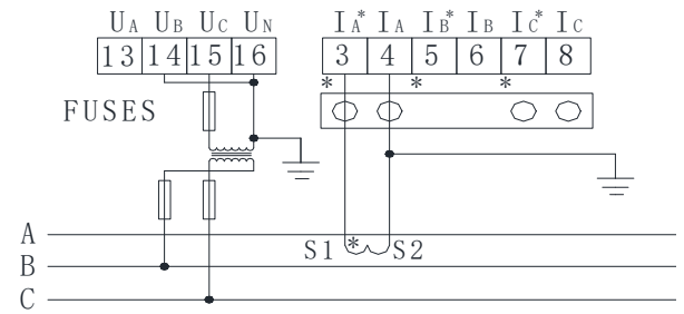
三相三线1PT、1CT
