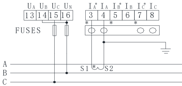
三相三线1CT
