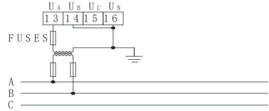
三相三线1PT
