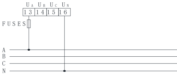
三相四线无PT
