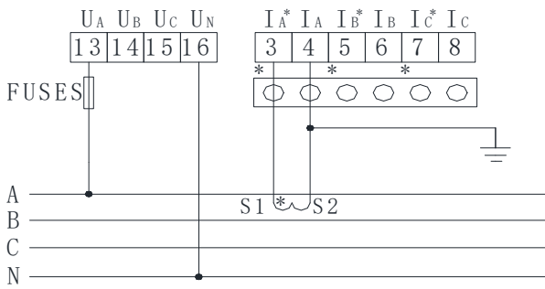
三相四线1CT
