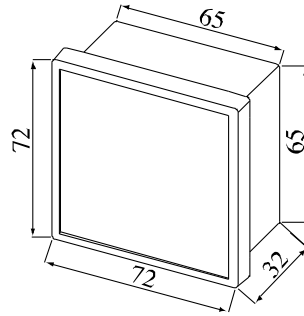
BD-4EA 显示头尺寸
