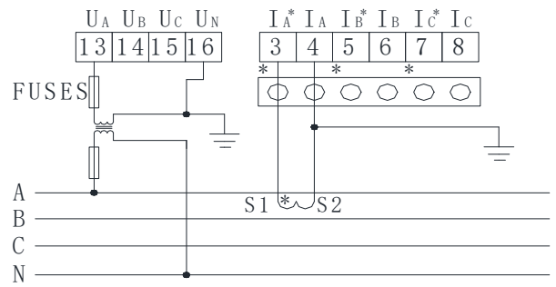
三相四线1PT、1CT
