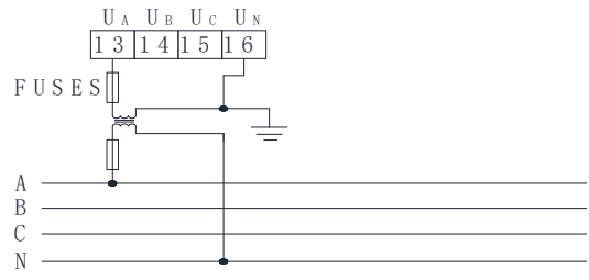
三相四线1PT
