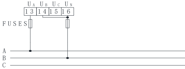
三相三线无PT
