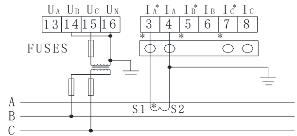
三相三线1PT、1CT
