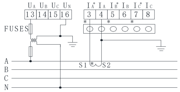
三相四线1PT、1CT
