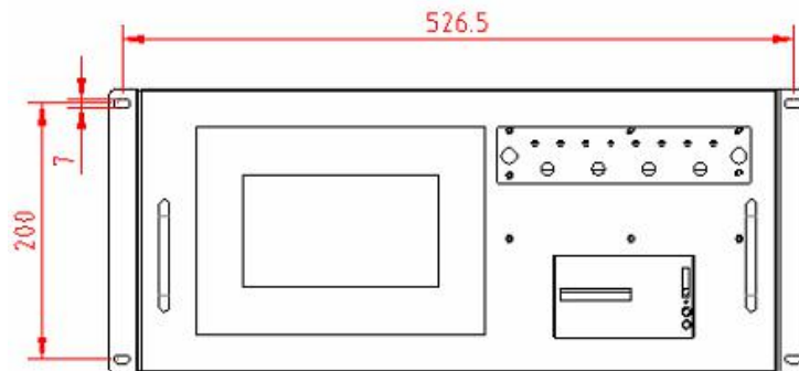
图 3 安装尺寸图
