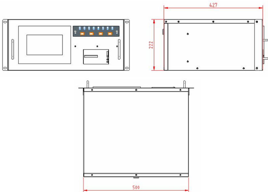
图 4 外形尺寸图
