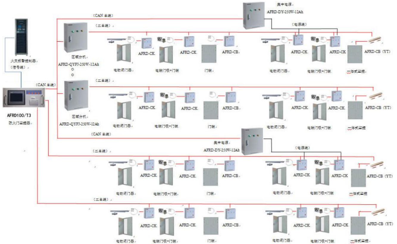
图 2 系统示意图
