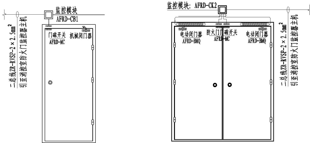
分体式防火门监控模块安装示意图（单扇、双扇）
