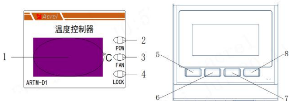
1.3 ARTM-D1 面板图
