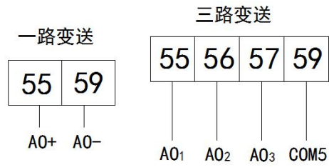
模拟量输出
