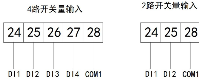
开关量输入
