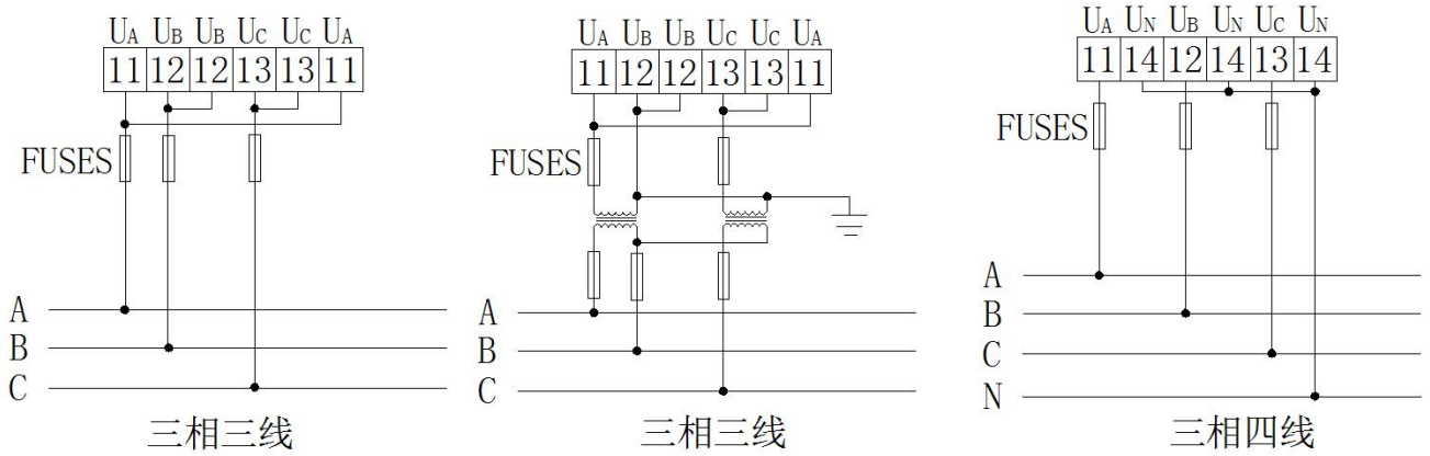
PZ48电压接线
