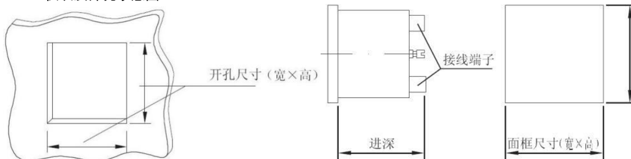
图1 开孔示意图
