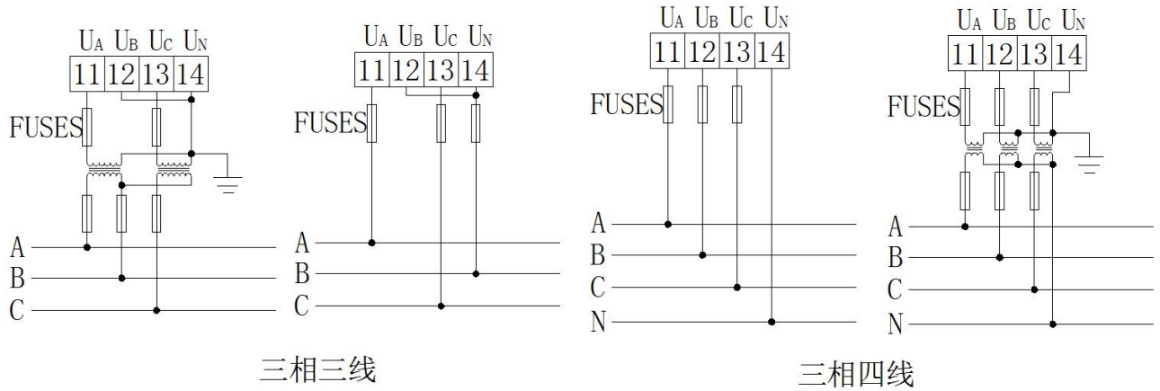
PZ72/80/96电压接线
