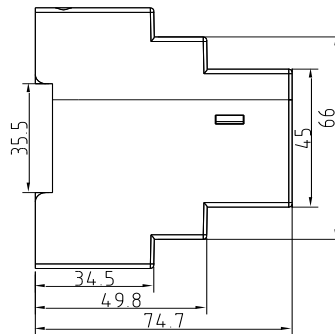
侧视图
