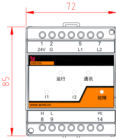
正视图
