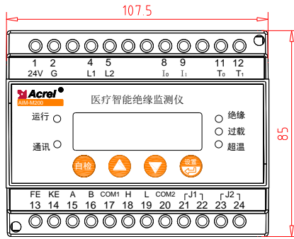
正视图
