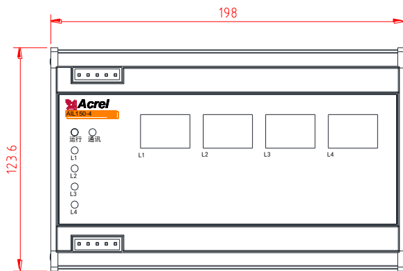
正视图
