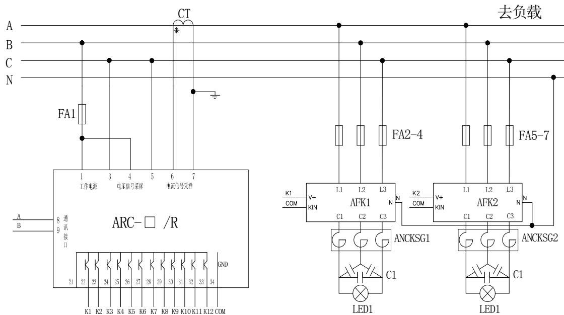
图6 工作电源为AC380V，线电压采样，带隔离的复合开关输出
