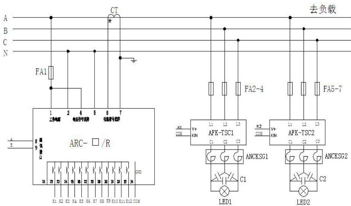
图7 工作电源为220V，相电压采样，带隔离的晶闸管开关输出
