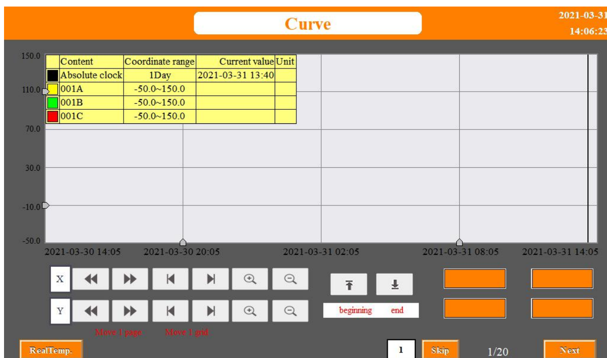
图 2.5 温度曲线
