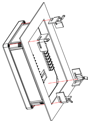
图 1.2 ASD100L/ASD100G 安装方法
