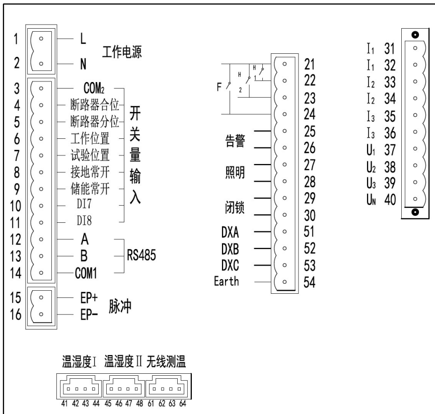
图 1.16 ASD300 背面端子图
