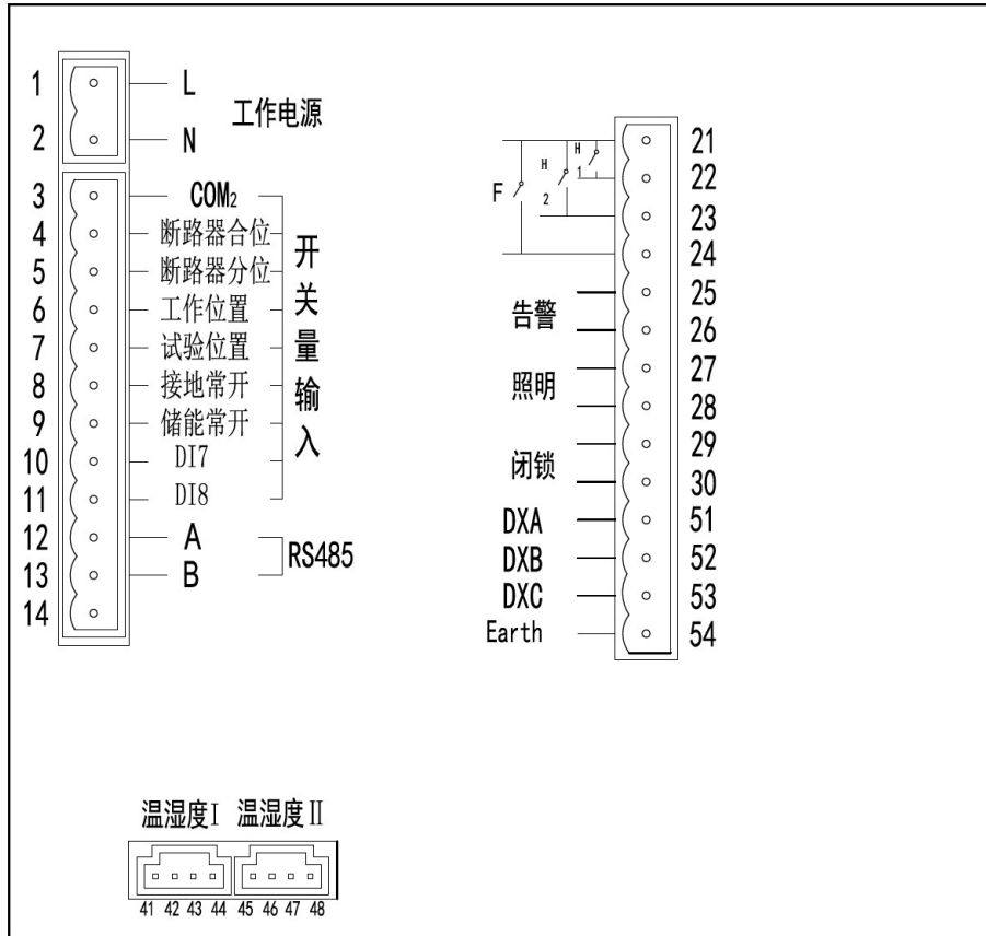
图 1.18 ASD200/310 背面端子图
