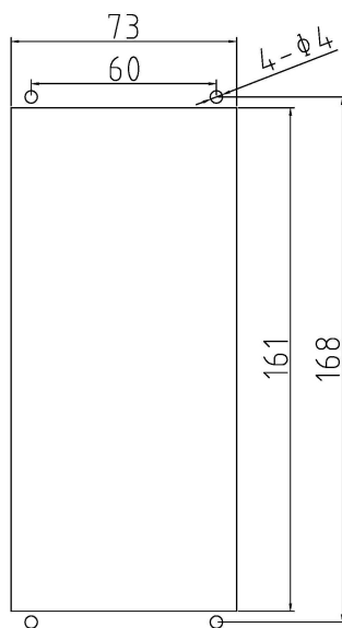
图 1.4 ASD100L 安装开孔尺寸
