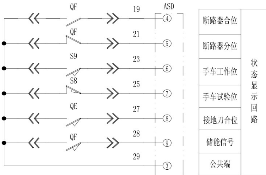
图 1.19 ASD 开关量输入回路典型接线图
