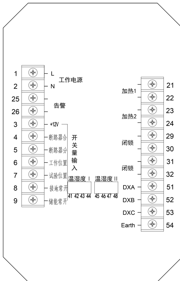
图 1.15 ASD100G 背面端子图
