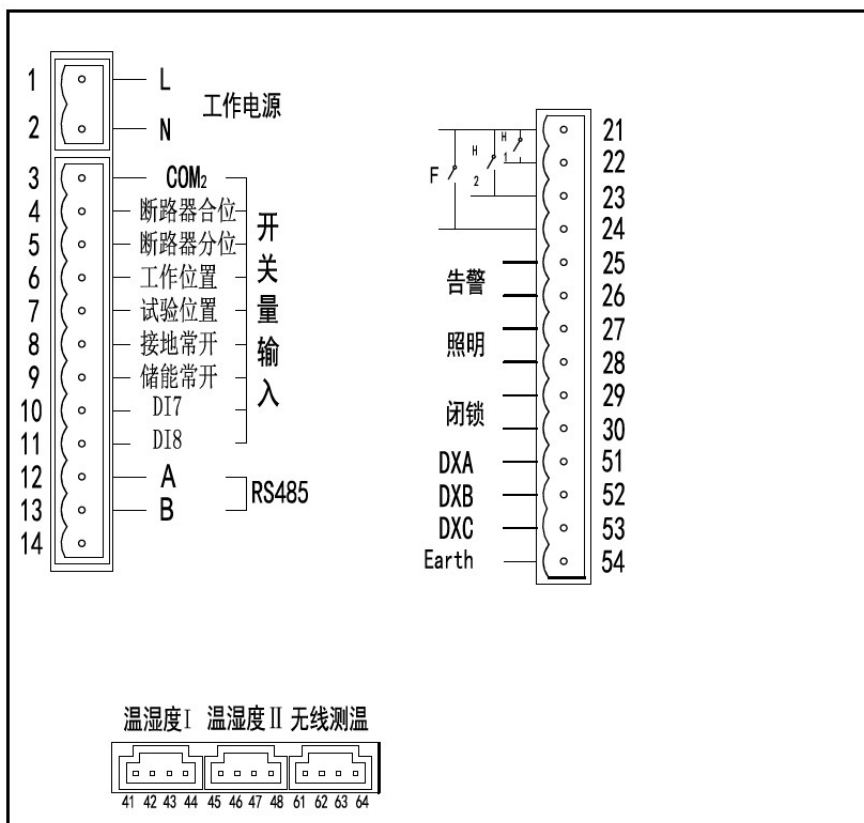
图 1.17 ASD320 背面端子图
