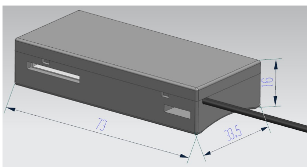
图 1.11 无源无线温度传感器 ATE300
